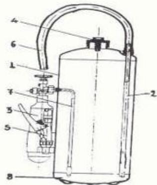
Πυροσβεστήρας ξηράς σκόνης με εξωτερικό φιαλίδιο CO 2
