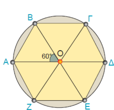
Κανονικό εξάγωνο
