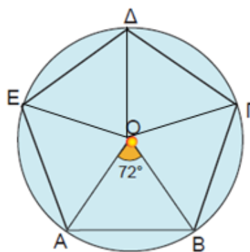
Κανονικό πεντάγωνο
