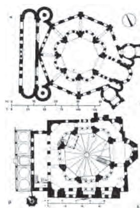
2. Κάτοψη περίκεντρου ναού α) Αγ. Βιταλίου, Ραβέννα. β) Αγ. Σεργίου και Βάχχου, Κωνσταντινούπολη.
