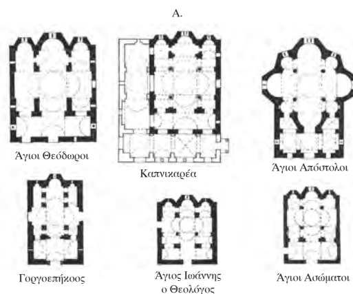
4. Κατόψεις σταυροειδούς βυζαντινού ρυθμού.
