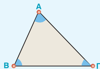
Γωνίες τριγώνου
