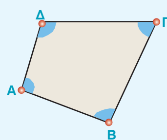
Γωνίες τετραπλεύρου
