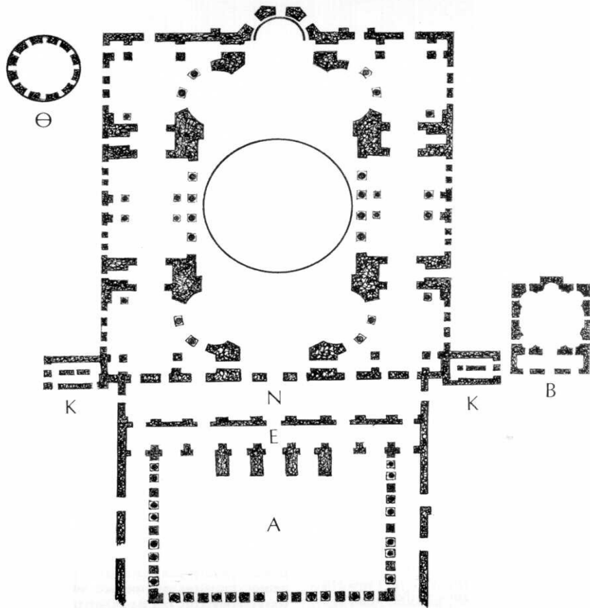
Κάτοψη Αγίας Σοφίας Κωνσταντινούπολη
