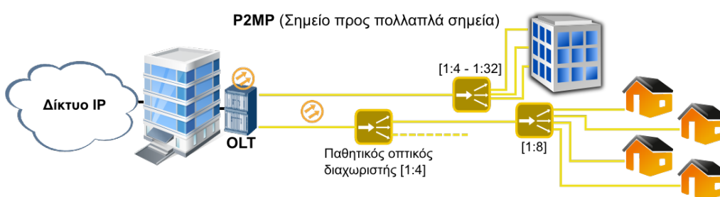
Εικόνα 5.2.δ: Αρχιτεκτονική «σημείο προς σημεία»
