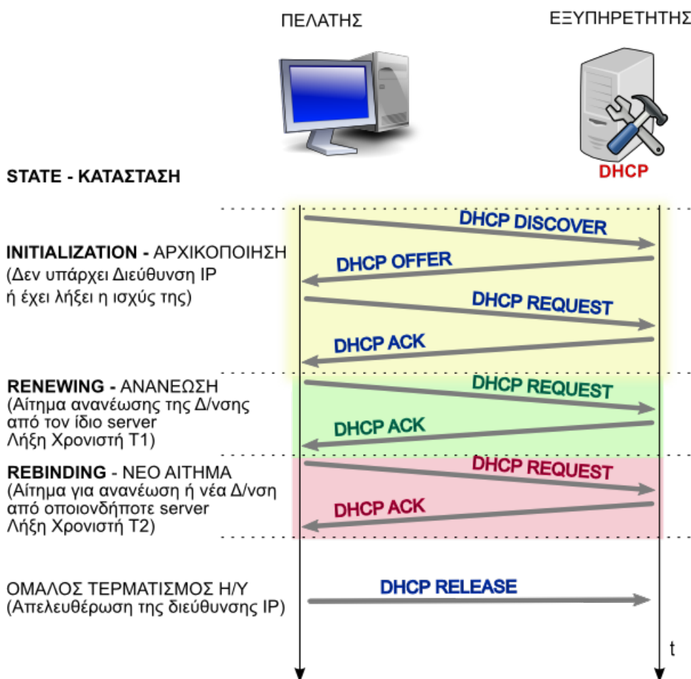
Εικόνα 3.2.2.α: Λειτουργία DHCP
