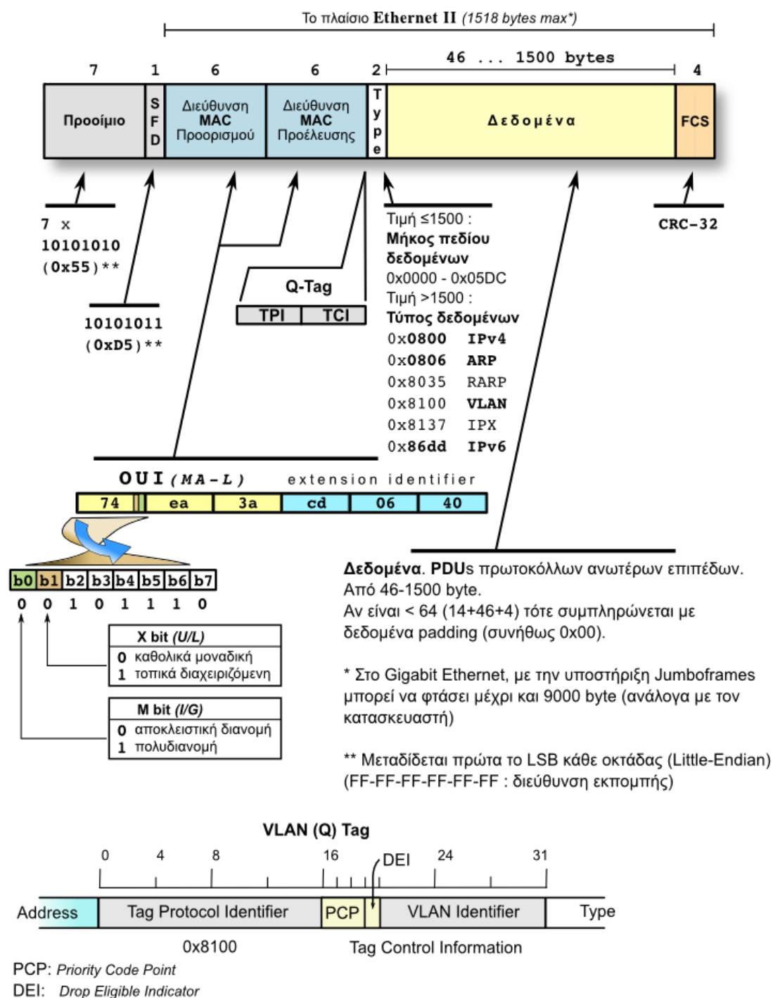
Εικόνα 2.4.2.δ: Δομή πλαισίου και διεύθυνσης MAC στο Ethernet
