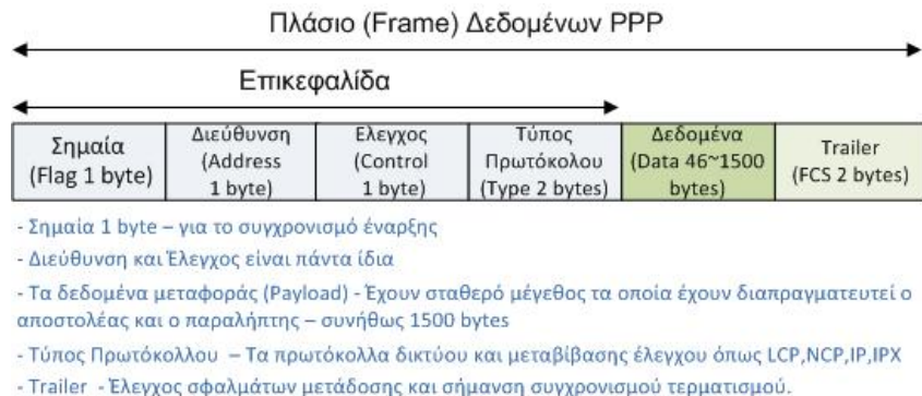
Εικόνα 2.7.β: Πλαίσιο PPP
