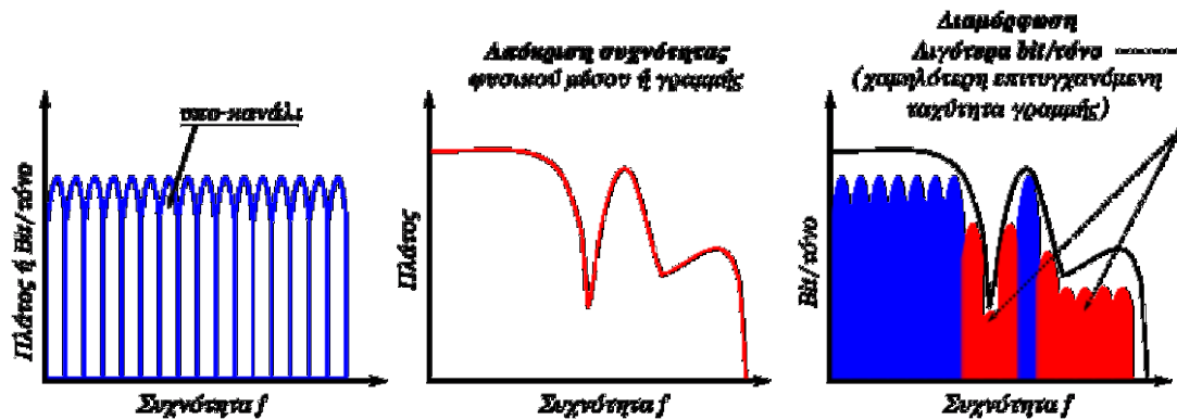
Εικόνα Π.3.α: Διαμόρφωση Διακριτής Πολυτονίας (DMT)
