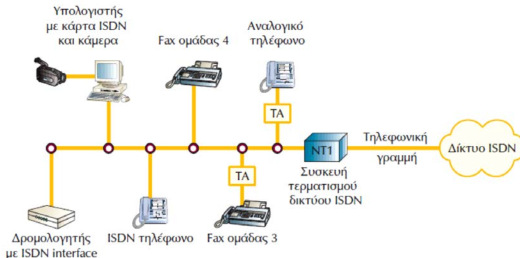
Σχήμα 5.1.3.β. Ο εξοπλισμός του ISDN
