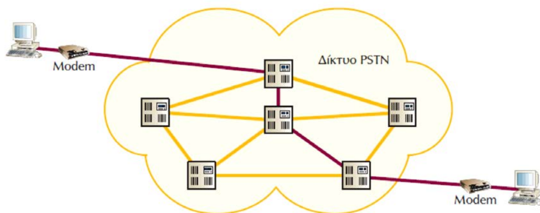
Σχήμα 5.1.1.α: Σύνδεση σταθμών μέσω δικτύου PSTN
