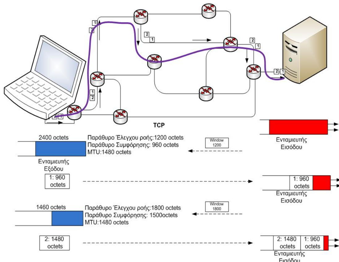
Εικόνα 4.1.4.β: Εγκατάσταση νέας Σύνδεσης με τριμερή χειραψία.
