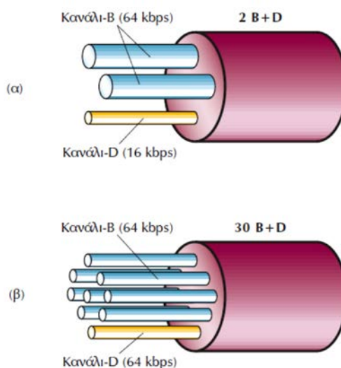
Σχήμα 5.1.3.α. Διεπαφή βασικού ρυθμού BRA (α) και Διεπαφή πρωτεύοντος ρυθμού PRA (β)
