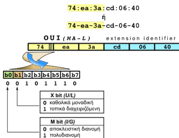
Εικόνα 2.4.2.α: Δομή διεύθυνσης MAC στο Ethernet
