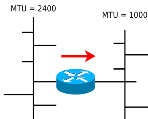
Εικόνα 3.2.ε: Δίκτυα με διαφορετικό MTU
