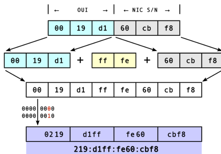
Εικόνα 3.5.1.α: Μεταγραφή διεύθυνσης MAC 48 bit σε EUI-64
