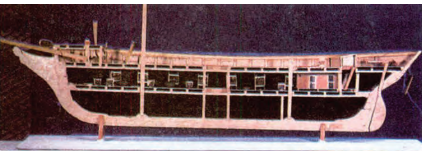
Ομοίωμα πυρπολικού του '21 (τομή). Αθήνα, Εθνικό Ιστορικό Μουσείο.
