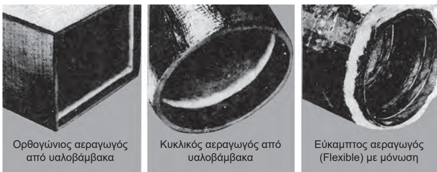
Εικόνα 12.4. Διατομές αεραγωγών από υαλοβάμβακα
