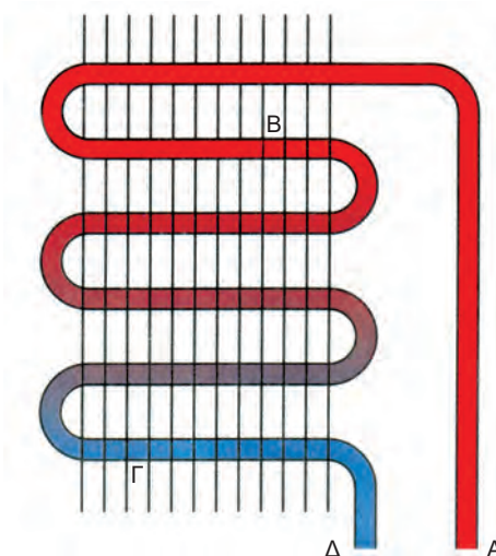
Σχήμα 4.3 Συμπυκνωτής οικιακού ψυγείου
