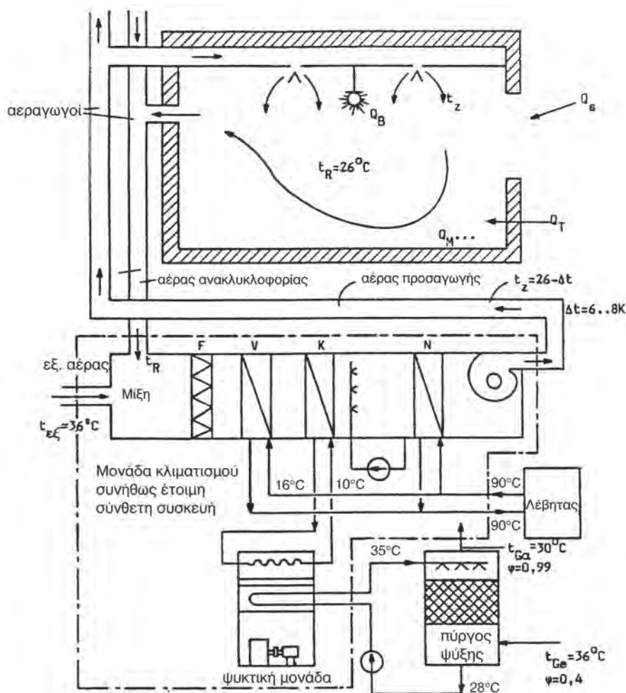
Σχήμα 9.4. Σύστημα κλιματισμού μόνο με αέρα
