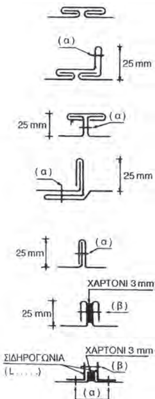
Σχήμα 12.3. Τρόποι σύνδεσης τμημάτων αεραγωγών από γαλβανισμένη λαμαρίνα
