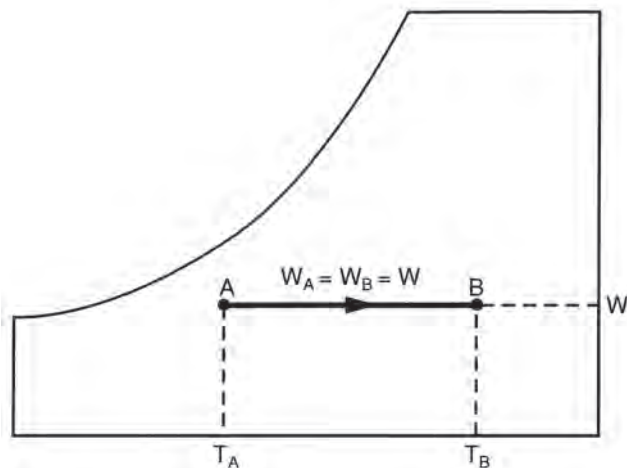
Διάγραμμα 10.10 Θέρμανση χωρίς ύγρανση
