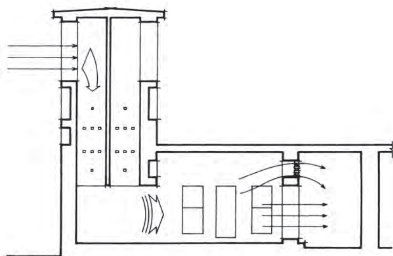
Σχήμα 1.2. Τομή παραδοσιακού αραβικού ανεμόμυλου
