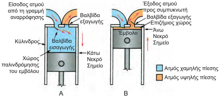
Σχήμα 6.4 Παλινδρομικός συμπιεστής A: φάση εισαγωγής B: φάση εξαγωγής
