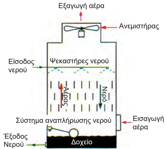
Σχήμα 6.11 Αρχή λειτουργίας του πύργου ψύξης
