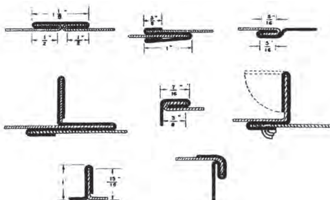
Σχήμα 12.3. Τρόποι σύνδεσης τμημάτων αεραγωγών από γαλβανισμένη λαμαρίνα
