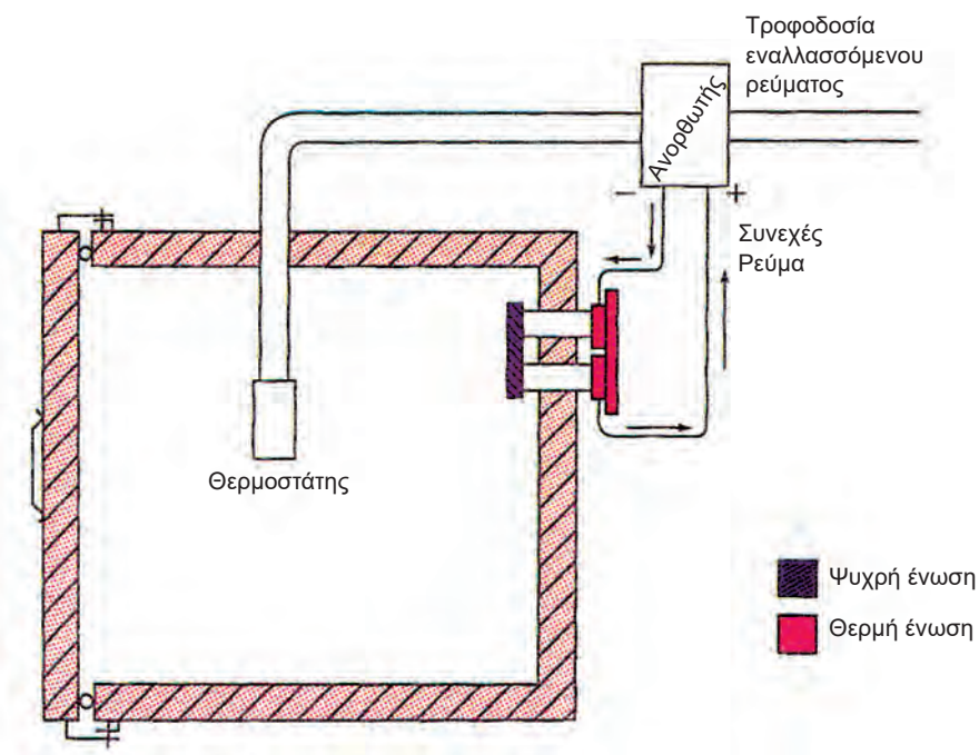
Σχήμα 7.4 Θερμοηλεκτρική ψύξη
