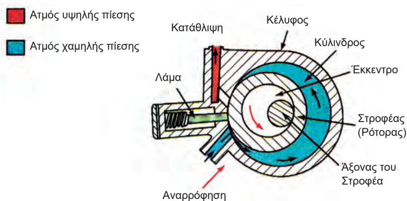
Σχήμα 6.6 Συμπιεστής τύπου τύμπανου (αρχή λειτουργίας)
