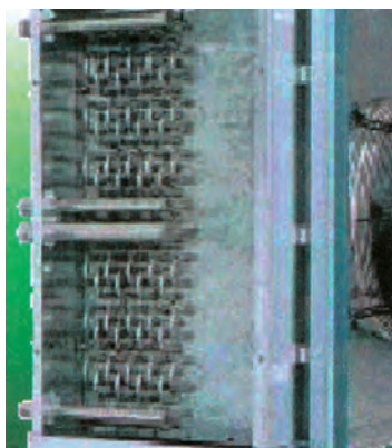
Εικόνα 6.22 Αποψη ενός τμήματος εξατμιστή αμμωνίας. Οι σωλήνες είναι από ανοξείδωτο ασάλι και τα περύγια από αλουμίνιο
