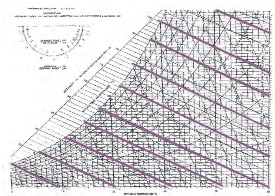
Διάγραμμα 10.2 Ευθείες θερμοκρασίας υγρού βολβού
