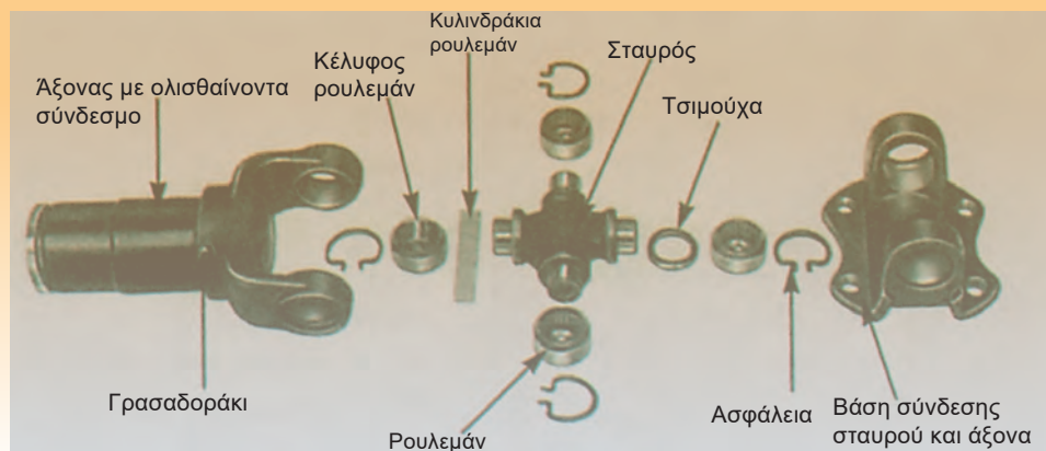
Σχήμα 1: Σύνδεσμος Cadran.
