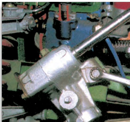
Σχήμα 5: Αφαίρεση πυξίδας.
