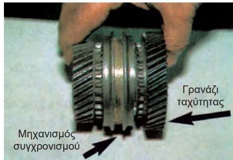
Σχήμα 2: Αποσυναρμολόγηση δευτερεύοντα.
