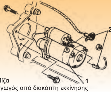
Σχήμα 2: Αφαίρεση του εκκινητή από το όχημα.
