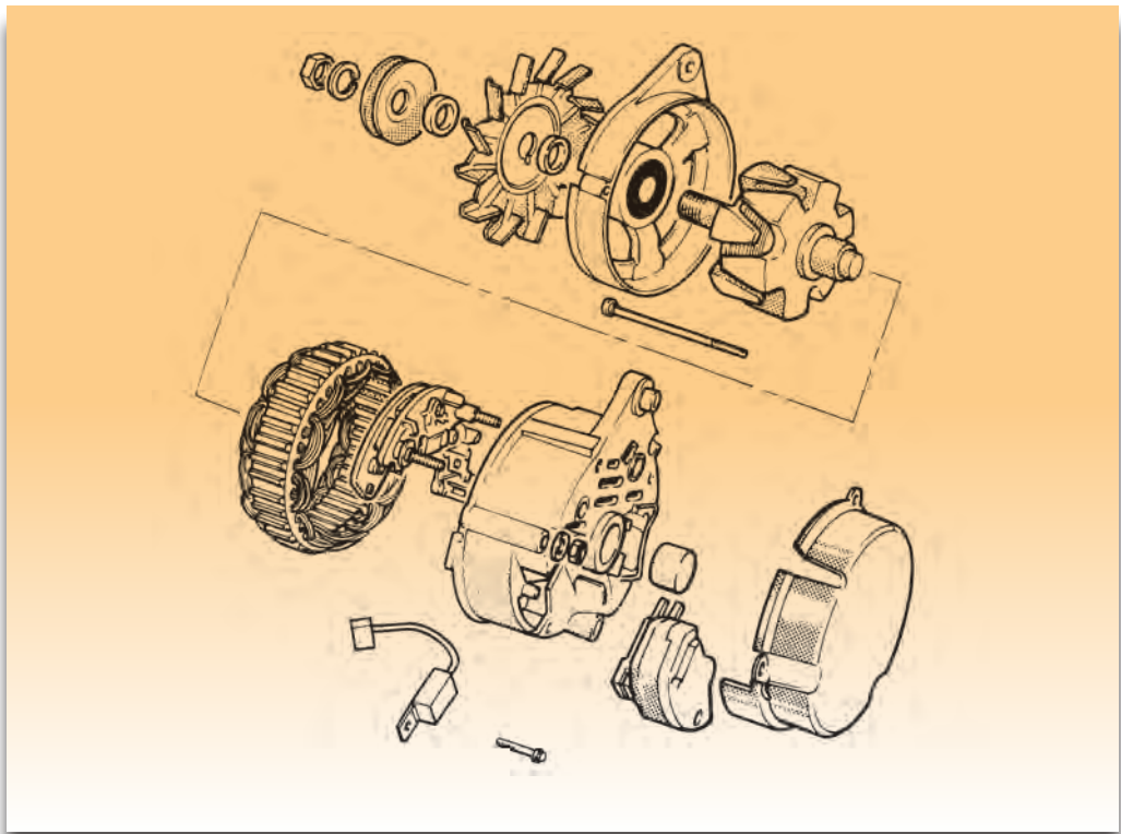
Σχήμα 1: Εναλλακτήρας αποσυναρμολογημένος.
