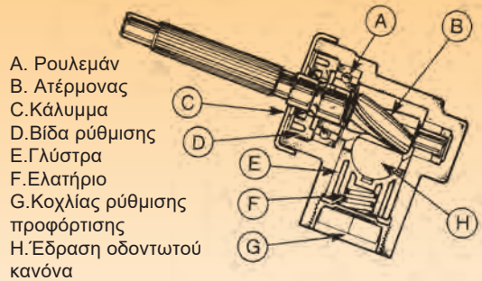
Διάταξη ρύθμισης της έδρασης του οδοντωτού κανόνα
