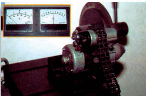
Σχήμα 4: Συγκράτηση και έλεγχος του εκκινήτη σε τραπέζι δοκιμής.
