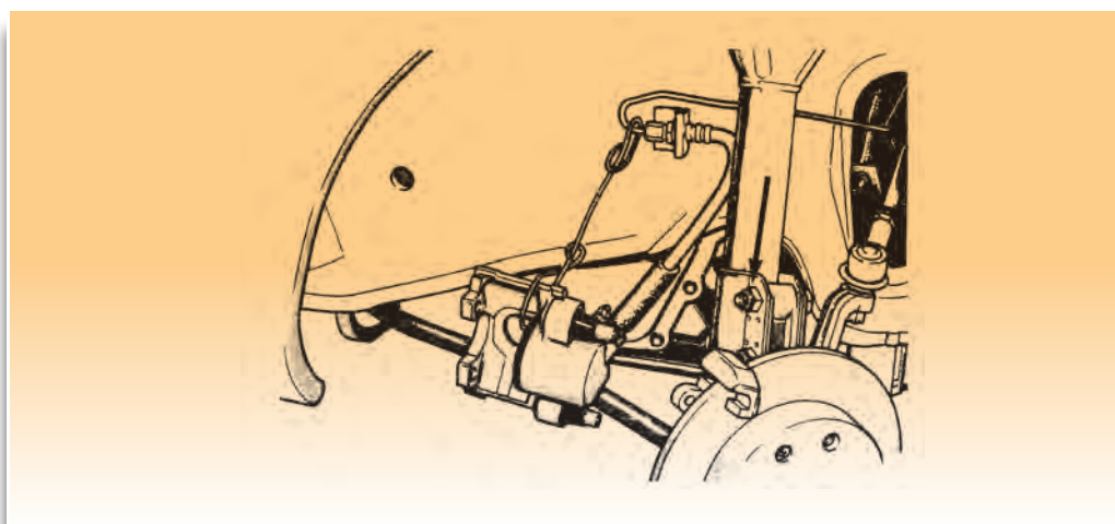
Σχήμα 5: Αφαίρεση της σύνδεσης της ανάρτησης και του δίχαλου των φρένων.
