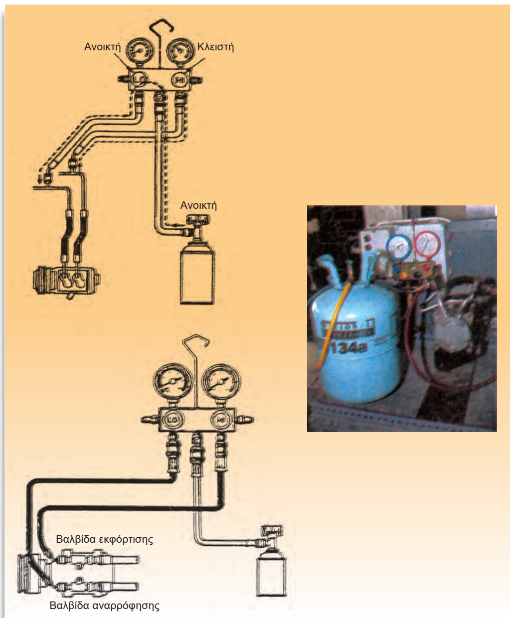
Σχήμα 4: Συμπληρωματική πλήρωση.
