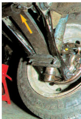
Σχήμα 6: Αφαίρεση των στηριγμάτων του ελατηρίου από το πλαίσιο ή το αμάξωμα.
