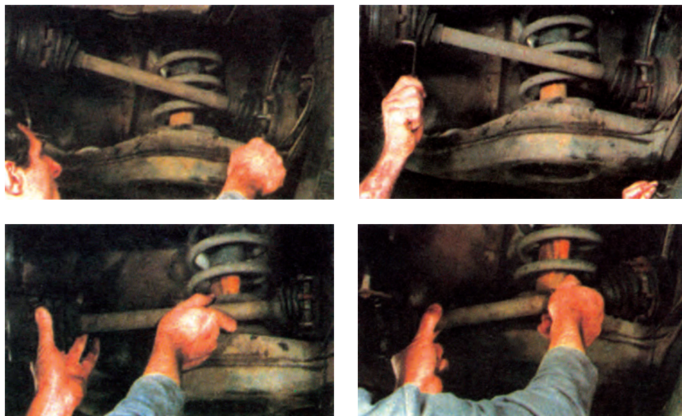
Σχήμα 11: Αφαίρεση της φούσκας των ημιαξόνων, και του ημιαξονίου.
