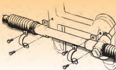
Σχήμα 5: Αφαίρεση κρεμαγιέρας.
