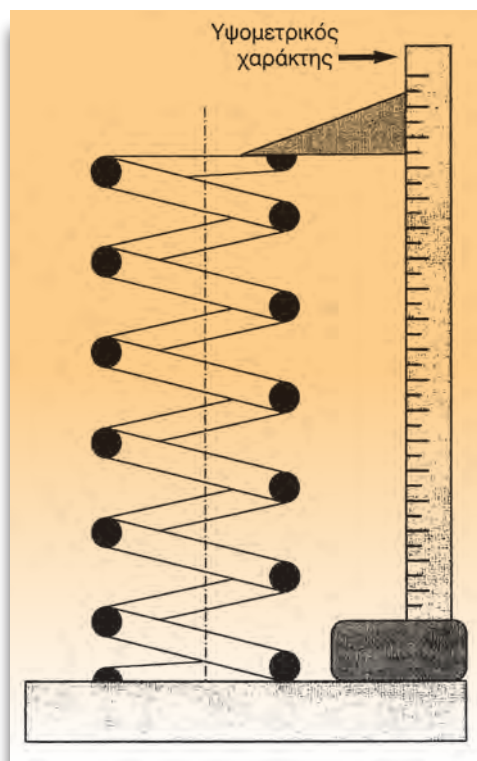
Σχήμα 9: Μέτρηση του ύψους του αφόρτιστου του ελατηρίου.
