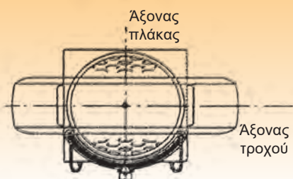
Σχήμα 3: Τοποθέτηση των μπροστινών τροχών στις πλάκες περιστροφής.
