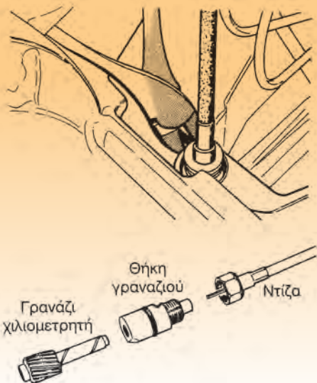
Σχήμα 11: Αφαίρεση του γραναζιού του χιλιομετρητή.
