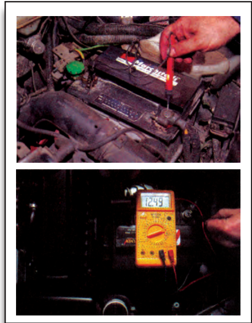
Σχήμα 5: Έλεγχος του συσσωρευτή με δοκιμαστικό και με βολτόμετρο.
