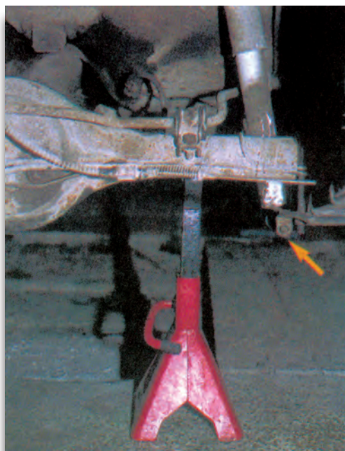
Σχήμα 2: Στήριξη του άξονα και αφαίρεση του αμορτισέρ.
