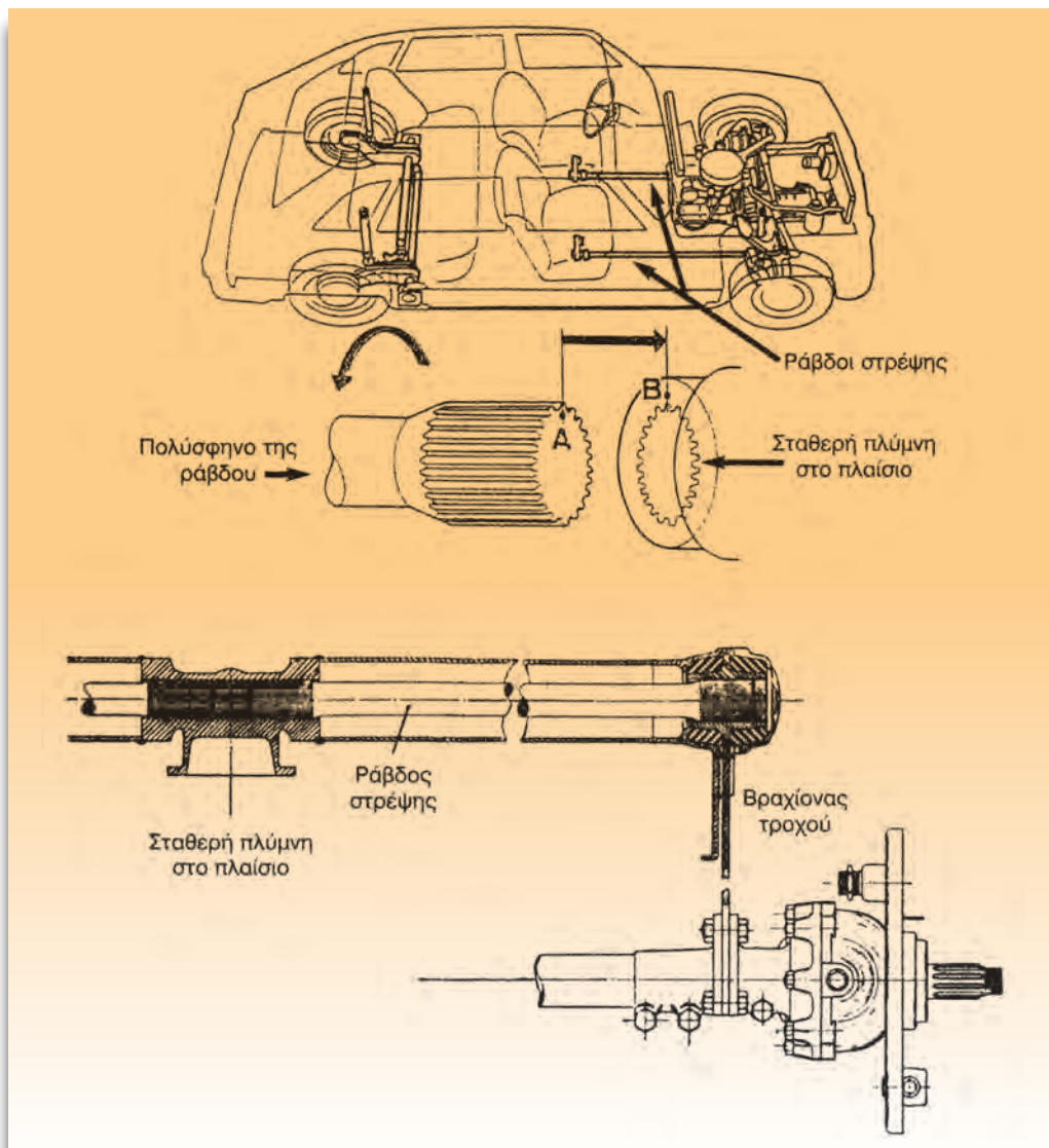
Σχήμα 1: Ανάρτηση με ράβδο στρέψης εμπρόσθιου και οπίσθιου άξονα.
