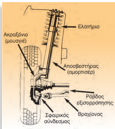
Σχήμα 1: Ανάρτηση MacPherson.
