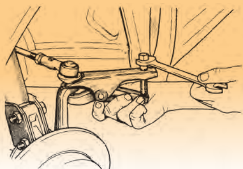
Σχήμα 3: Αφαίρεση κινητηρίων τροχών και ακρόμπαρα.
