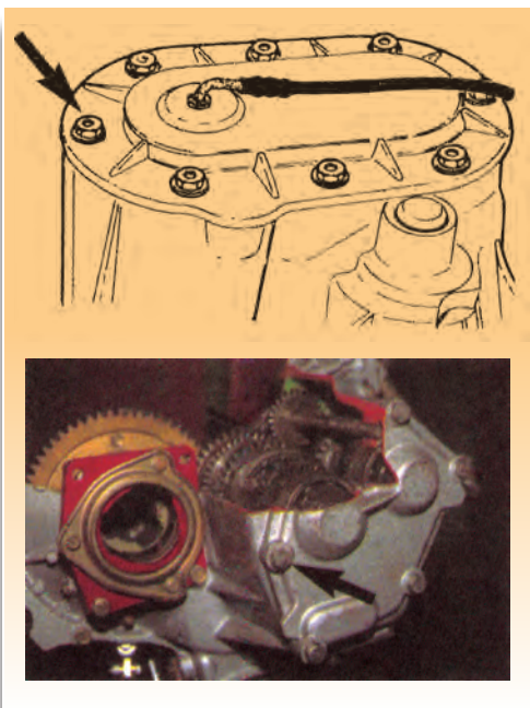
Σχήμα 5: Αφαίρεση του καπακιού του κιβωτίου ταχυτήτων.
