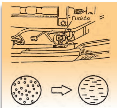
Σχήμα 5: Οπτικός έλεγχος του δείκτη ροής.
