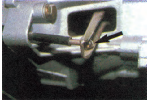
Σχήμα 4: Αποσύνδεση της ντίζας του συμπλέκτη.
