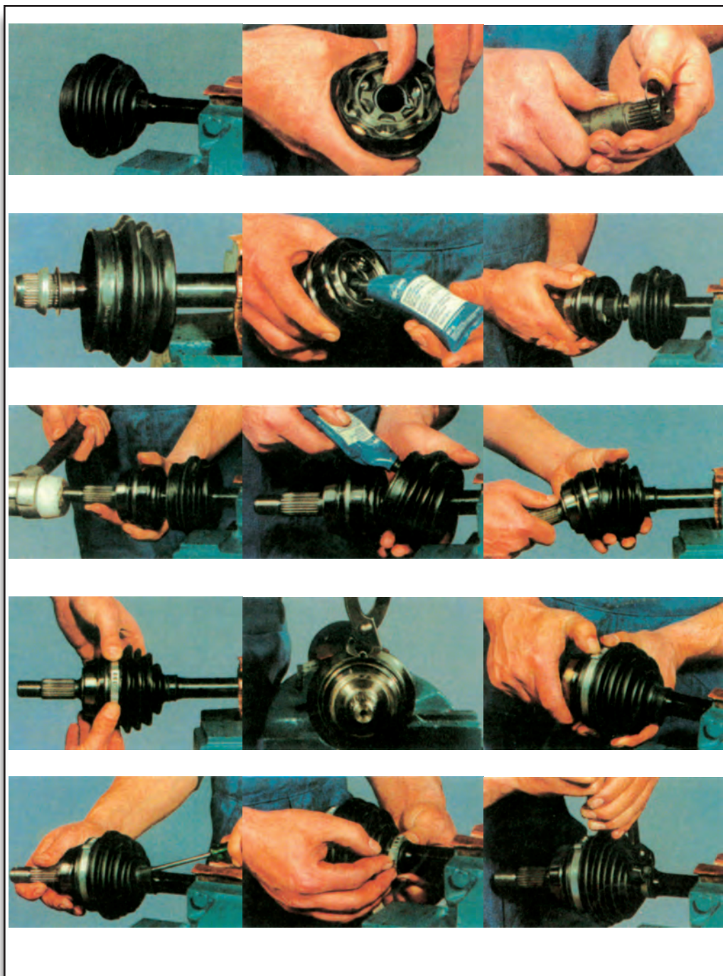
Σχήμα 9: Συναρμολόγηση του συνδέσμου με το ημιάξονιο.
