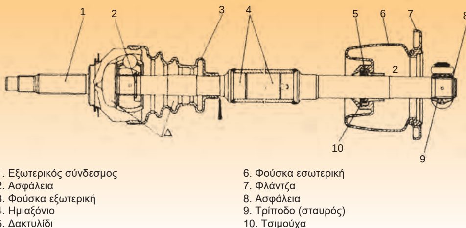
Σχήμα 1: Σύνδεσμοι σταθερής ταχύτητας.
