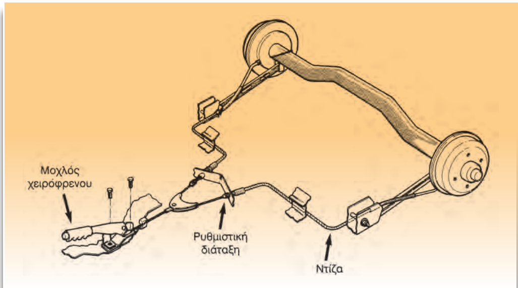
Σχήμα 1: Διάταξη χειροφρένου.
