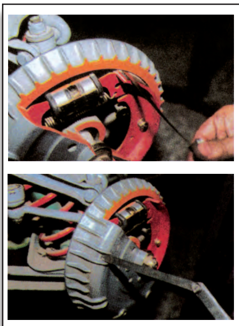
Σχήμα 2: Έλεγχος διακένου σιαγόνας - ταμππούρου.
