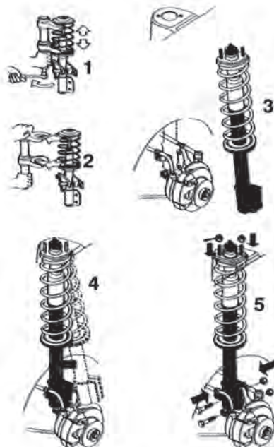
Σχήμα 4: Διαδικασία αντικατάστασης αμορτισέρ.
