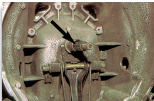
Σχήμα 12: Έλεγχος του κελύφους του συμπλέκτη για διαρροές.
