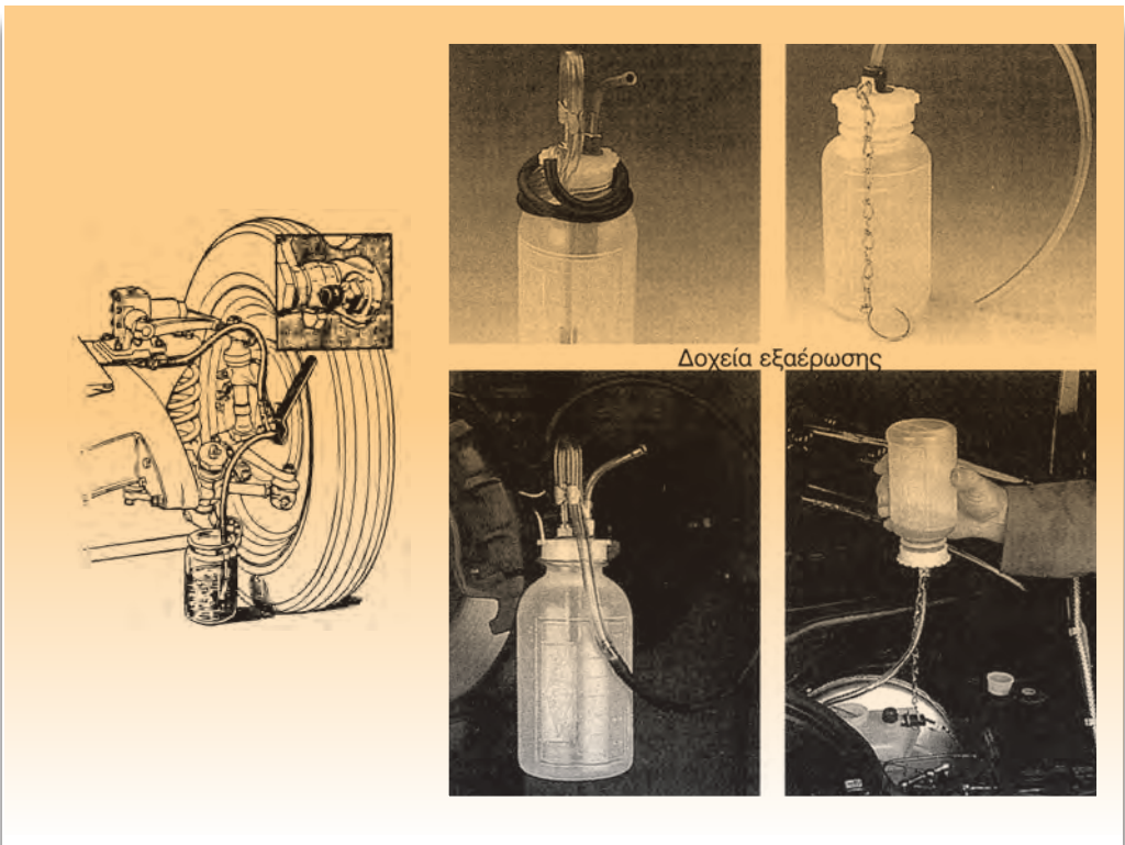
Σχήμα 2: Προετοιμασία για εξαέρωση.
