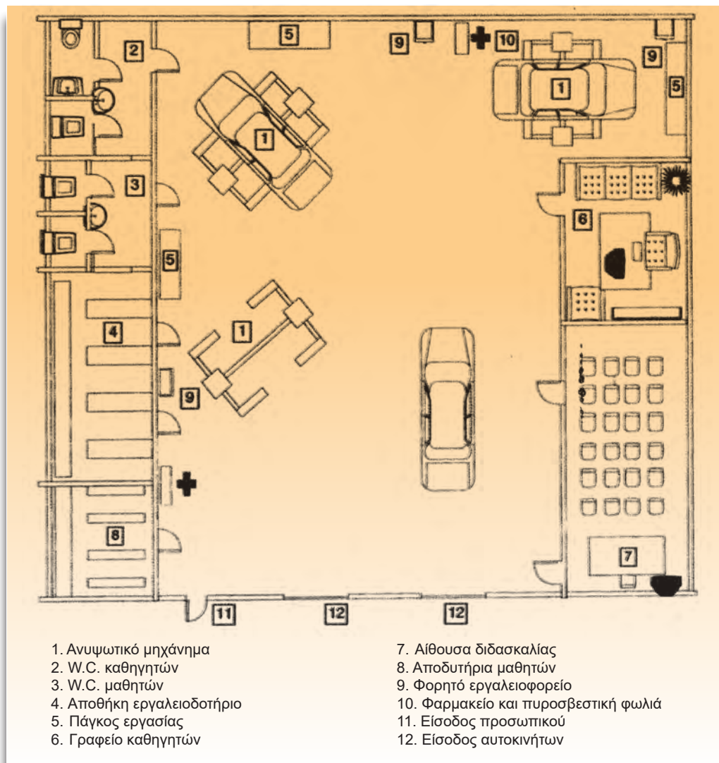
Σχήμα 1: Κάτοψη εργαστηρίου.
