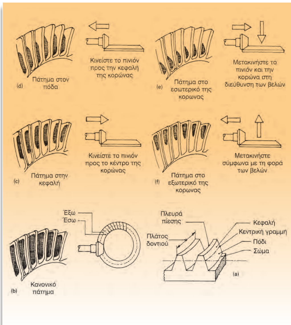
Σχήμα 4: Έλεγχος πατήματος κορώνας - πινιόν.
