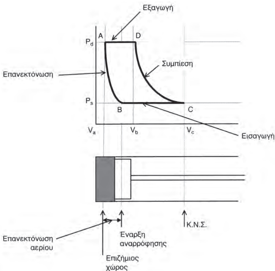
Σχήμα 4.1.4 Διάγραμμα πίεσης-όγκου.
