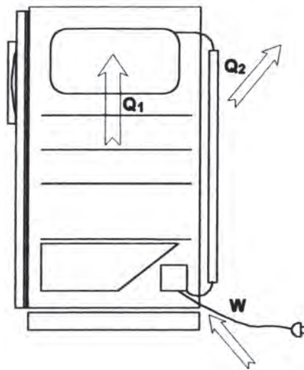
Σχήμα 1.3.1 “Οικιακό ψυγείο
