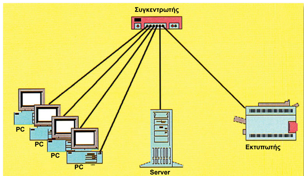
Σχήμα 2.1: Τοπολογία αστέρα.
