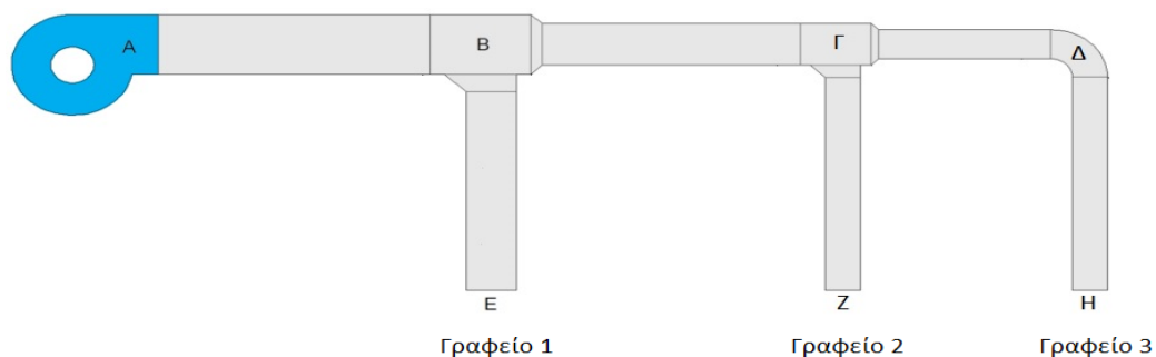
Σχήμα 1: Κάτοψη δικτύου αεραγωγών ενός μελετητικού γραφείου.
