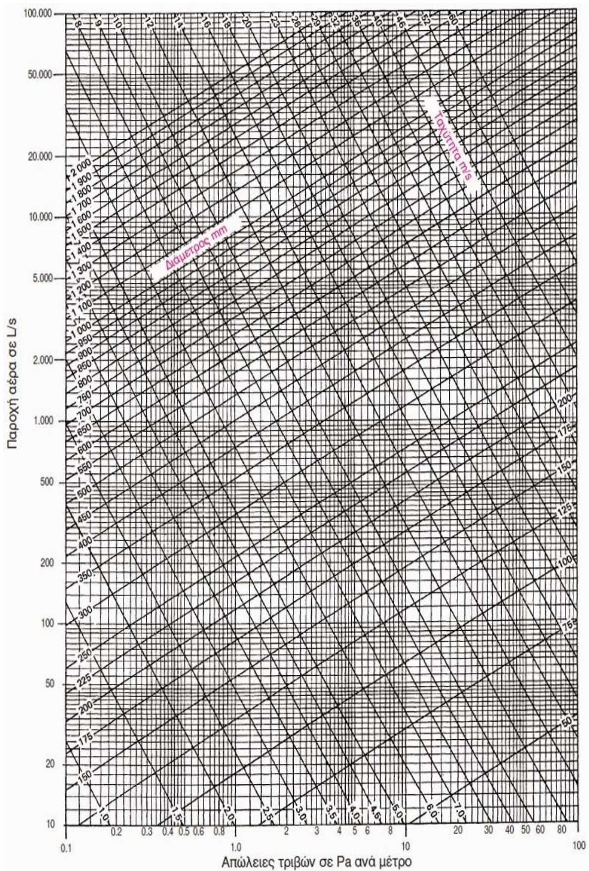
Διάγραμμα 1: Διάγραμμα υπολογισμού της διαμέτρου κυκλικού αεραγωγού.
