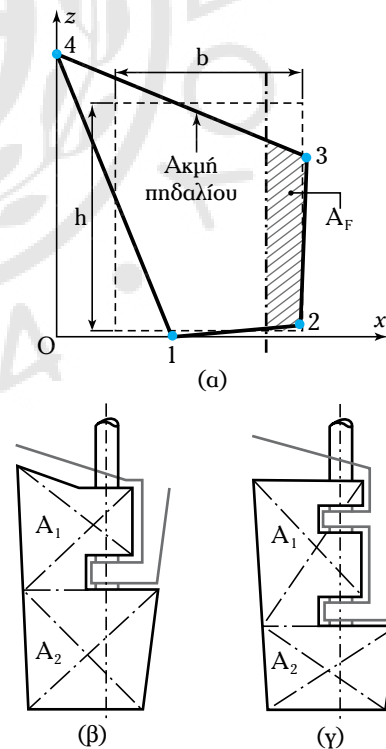
(α) Περιγραφή κρεμαστού πηδαλίου σε καρτεσιανό σύστημα. (β) Πηδάλιο με ποδόστημα και μονό πείρο. (γ) Πηδάλιο με ποδόστημα και διπλό πείρο.
