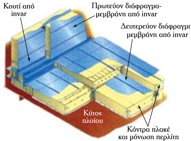
(α) Διάταξη υλικών μονώσεων
