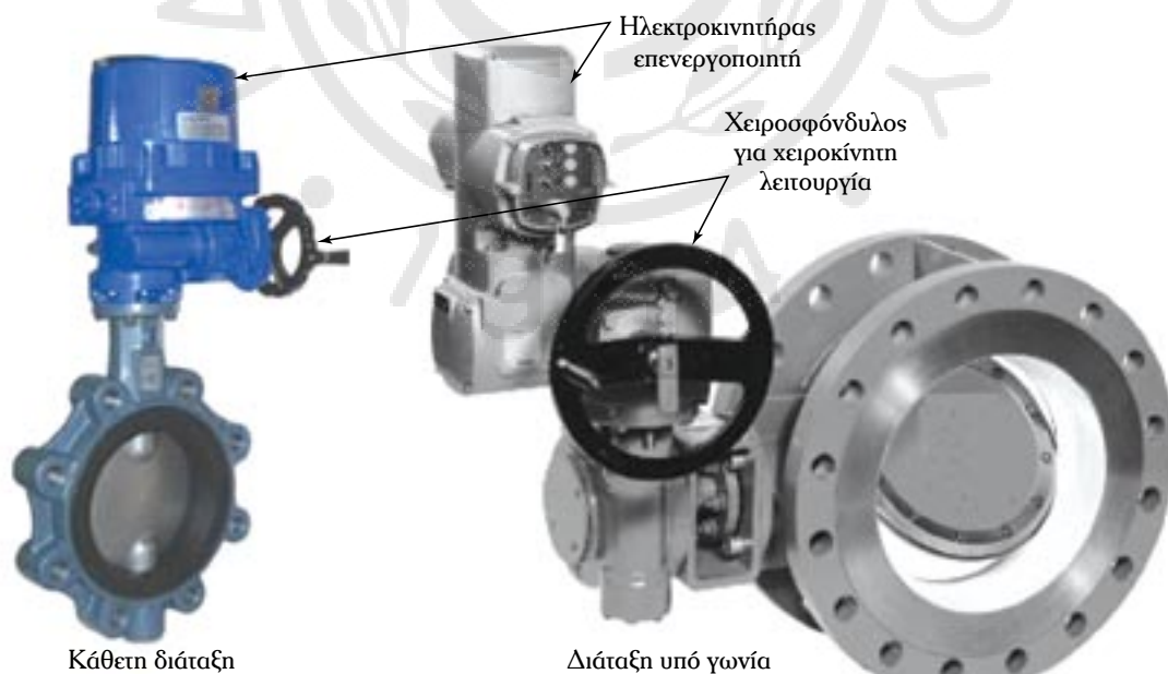
Σχ. 7.7γ Ηλεκτροκίνητος επενεργοποιητής συνδεδεμένος σε επιστόμιο τύπου πειαλούδας.
