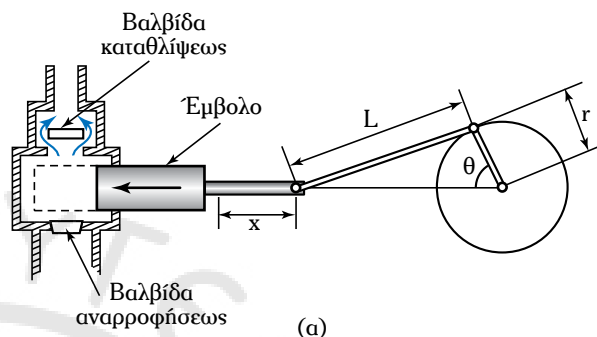
Τυπική διάταξη στροφαλοκίνητης αντλίας
