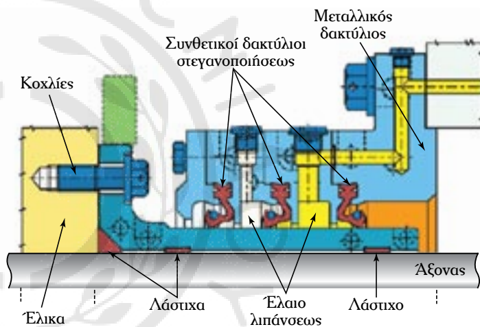
(β) Διαρρέσιμο σύστημα στεγανοποίησης.
