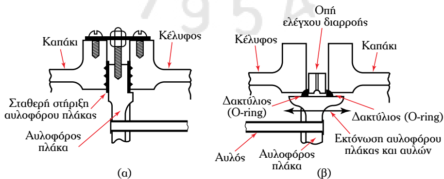
Σχ. 3.4δ Στεγανοποίηση αυλοφόρου πλάκας στις δύο πλευρές ενός εναλλακτήρα.
