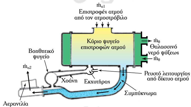
Σχ. 5.6α Ἐνισχυτής κενού.
