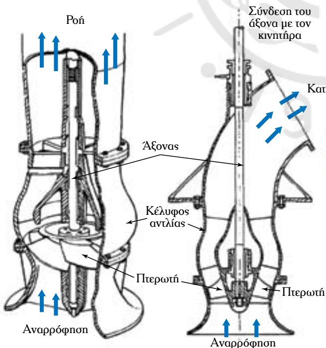
(α) Τομή κάθετης διατάξεως αντλίας αξονικής ροής
