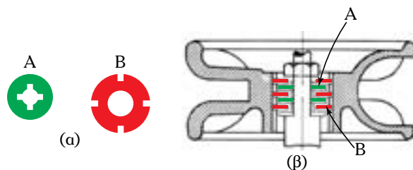
Σχ. 13.5β (α) Μορφή δίσκων αλυσέλικτρου και (β) διάταξή τους σ' αυτό.
