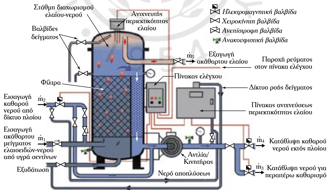
Σχ. 15.2β Διαχωριστής με φίλτρα.
