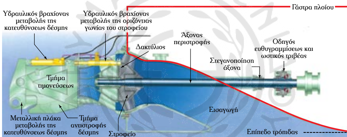
Σχ. 19.12α Διάταξη ουστήματος υδροπροώσεως.
