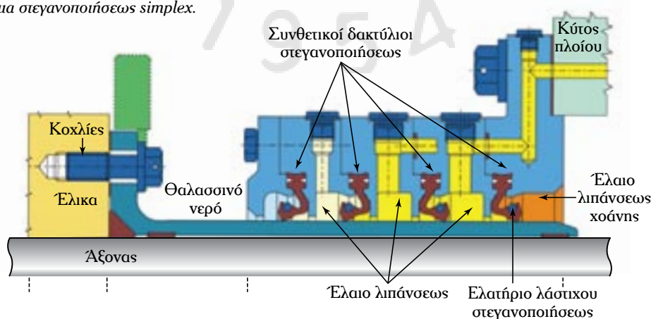
(γ) Μη διαρρέσιμο σύστημα στεγανοποίησης.
