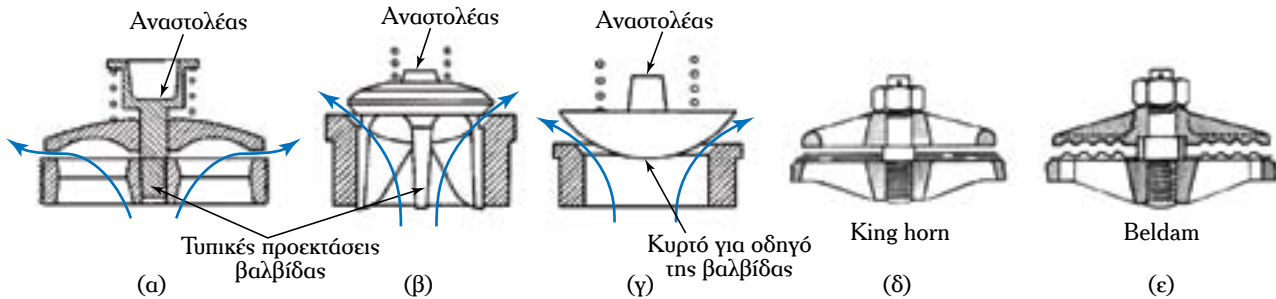
Σχ. 2.8n Τύποι βαλβίδων.
