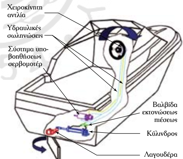
Σχ. 14.4δ Υδραυλικό σύστημα πηδαλίου σε λέμβο.
