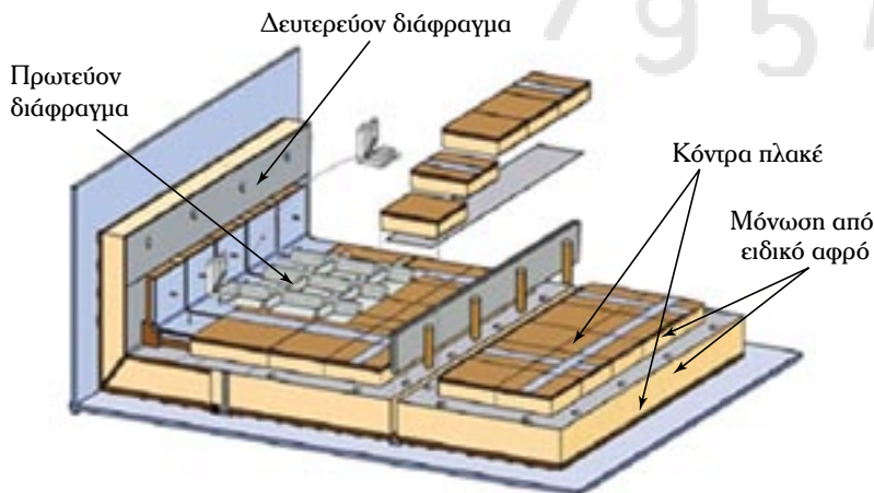
(α) Διάταξη υλικών μονώσεων
