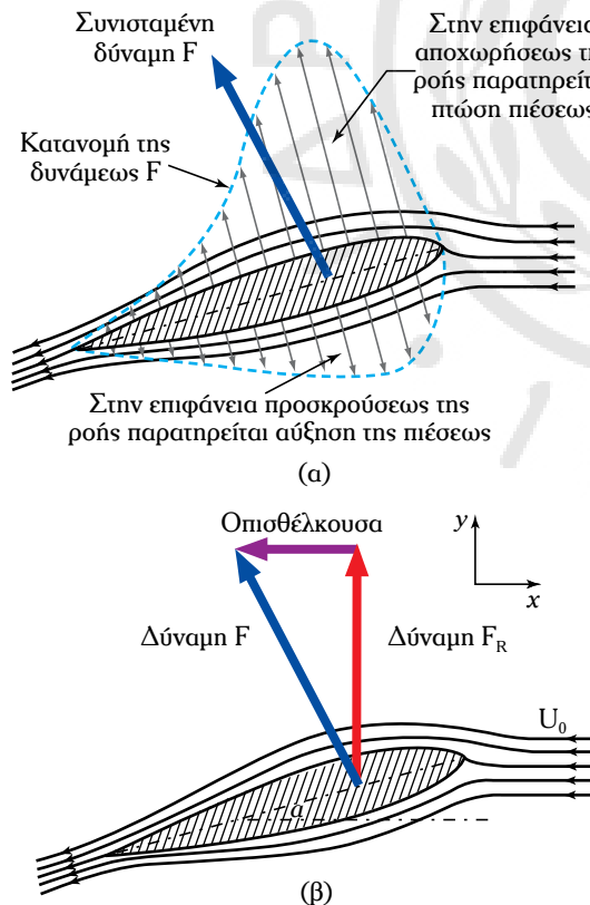
Σχ. 14.3α Δυνάμεις που αναπτύσσονται στο πηδάλιο όταν αυτό έχει γωνία \hat{\alpha} , σε ρευστό με ταχύτητα U_0 .
