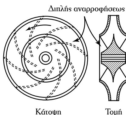
Στροφεία-περωτές κλειστού τύπου
