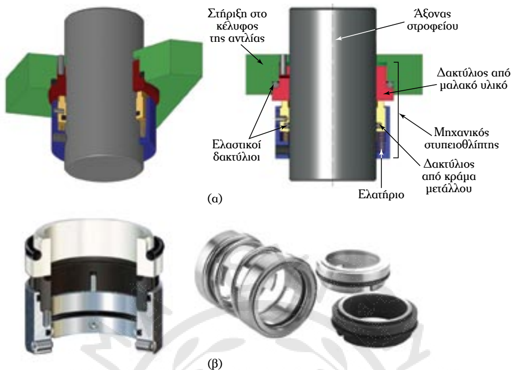
Σχ. 2.20β Μηχανικός στυπιοθλίπτης.
