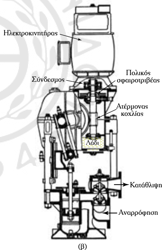
Τομή στροφαλοκίνητης αντλίας
