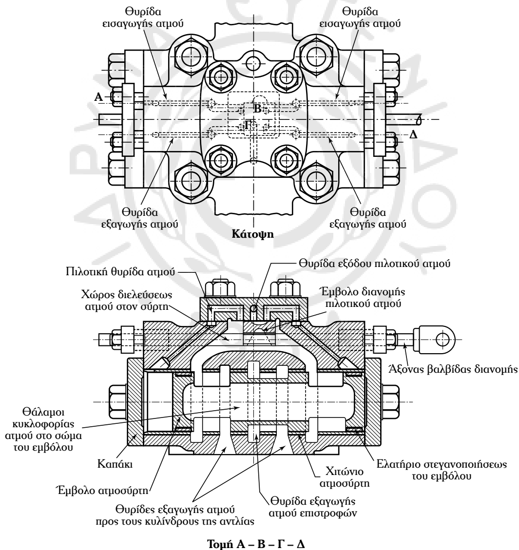
Σχ. 2.8ιβ Μηχανισμός διανομής ατμού.
