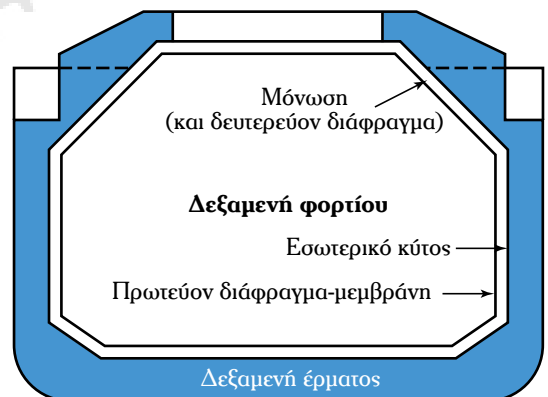
(β) Τομή δεξαμενής
