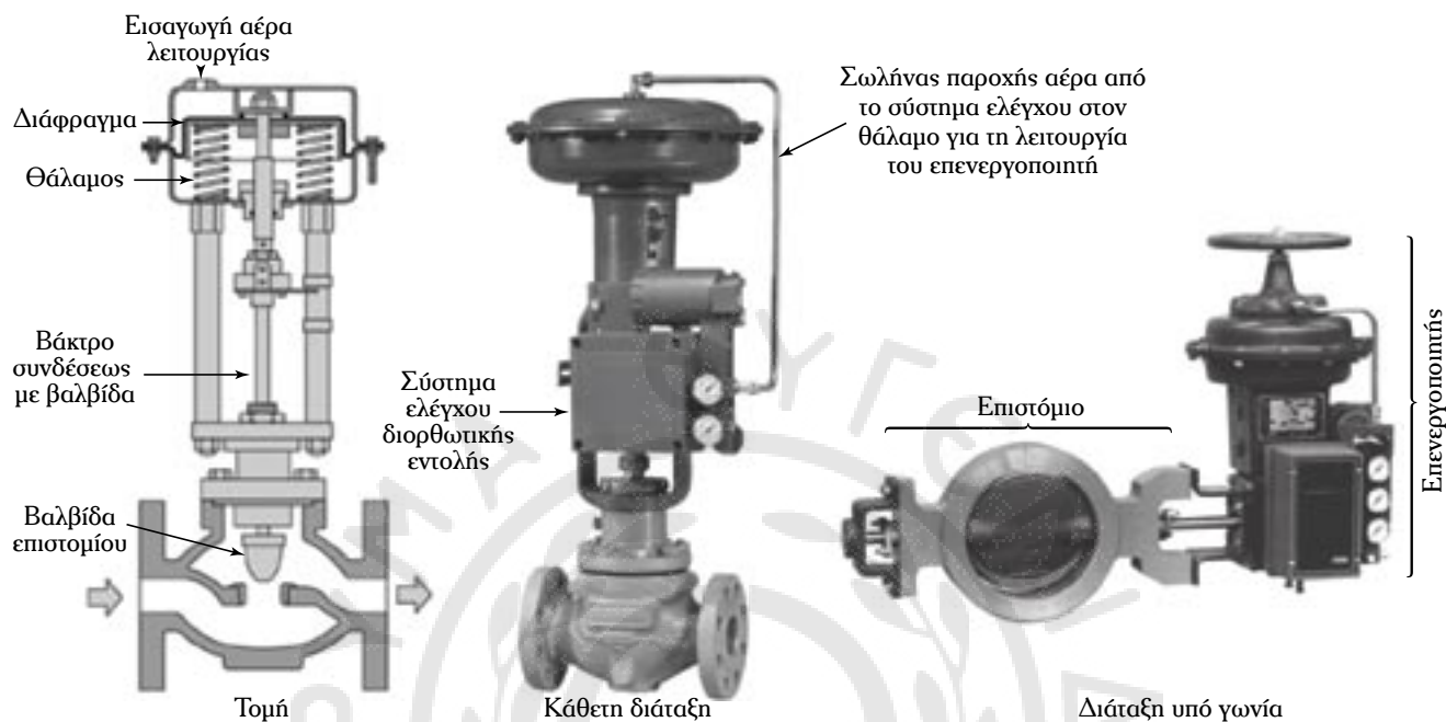
Σχ. 7.7β Επενεργοποιητής με επιστόμιο.
