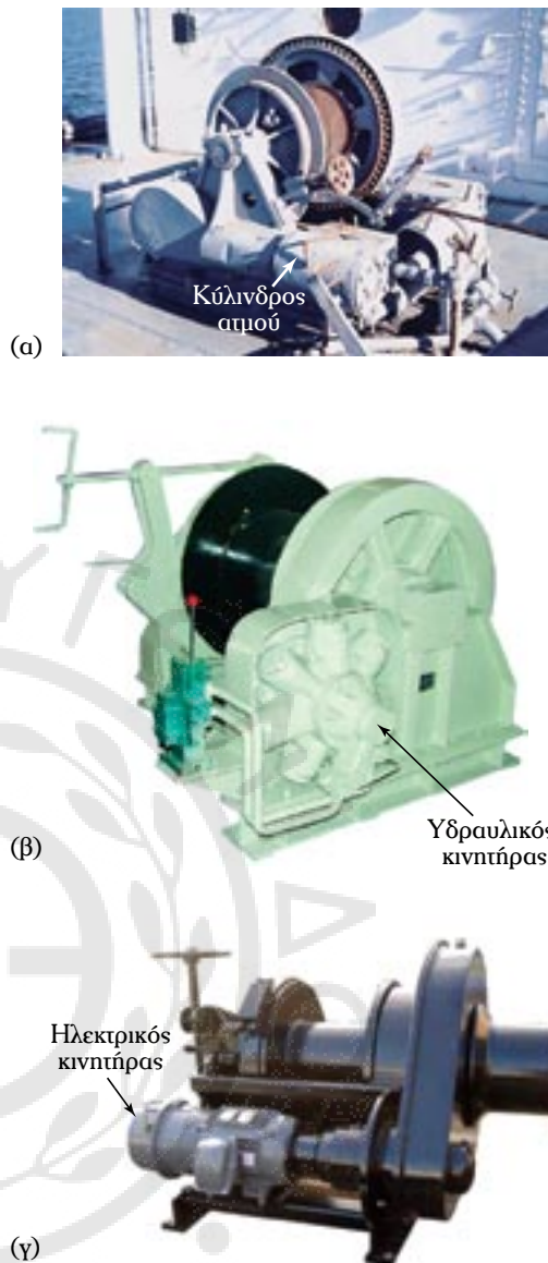
Σχ. 13.6β Τύποι βιντζιών.
