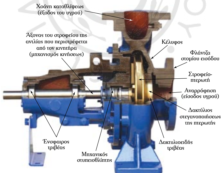
Σχ. 2.10α Φυγοκεντρική αντλία.
