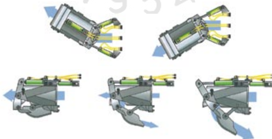
Σχ. 19.12β Διάταξη και κινήσεις του στομίου εξαγωγής (νερού σε σύστημα υδροπροώσεως).
