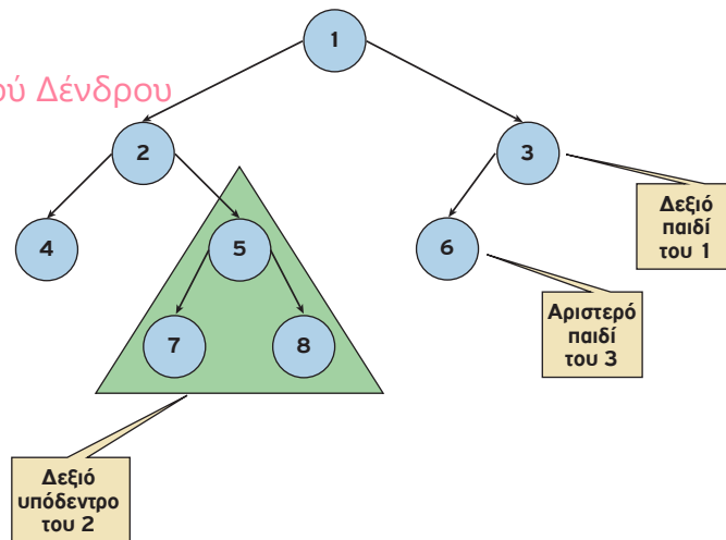
Εικόνα 1.3.21. Δυαδικό δένδρο
