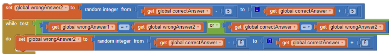
Εικόνα 152 - Ο έλεγχος της δεύτερης λανθασμένης απάντησης
