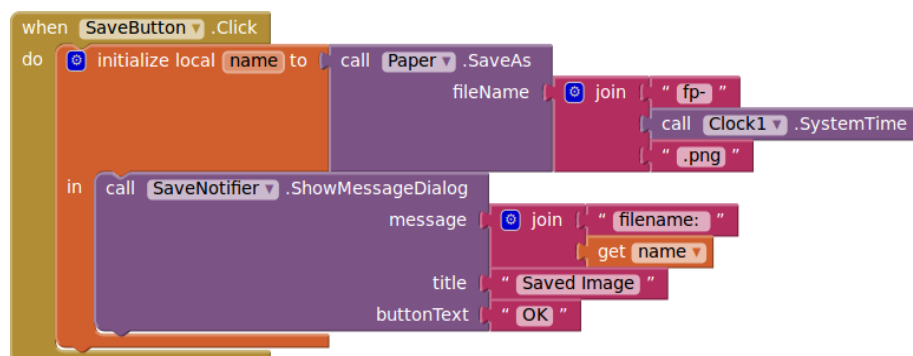
Εικόνα 122 - Αποθήκευση του σχεδίου με αυτόματη καταχώρηση ονόματος
