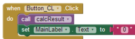
Εικόνα 143 - Κλήση της διαδικασίας καθαρισμού
