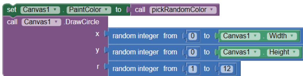
Εικόνα 162 - Τυχαία σχεδίαση ενός κύκλου
