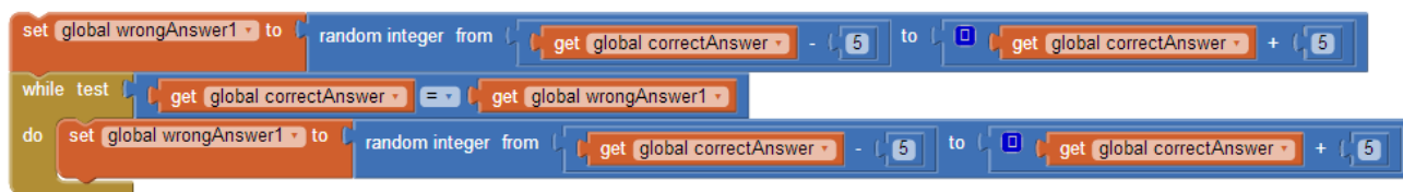
Εικόνα 151 - Η ολοκληρωμένη εντολή while
