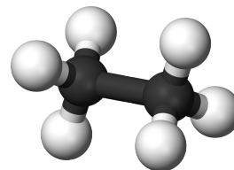
Μοντέλο δομής του αιθανίου ( C_2H_6 ).
