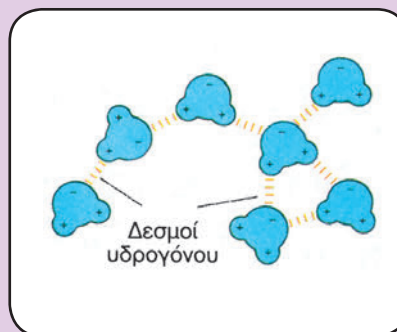
Δεσμοί υδρογόνου μεταξύ του μορίου του νερού.
