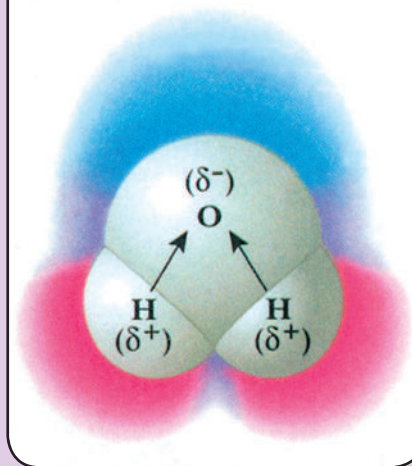
Μόριο νερού.
