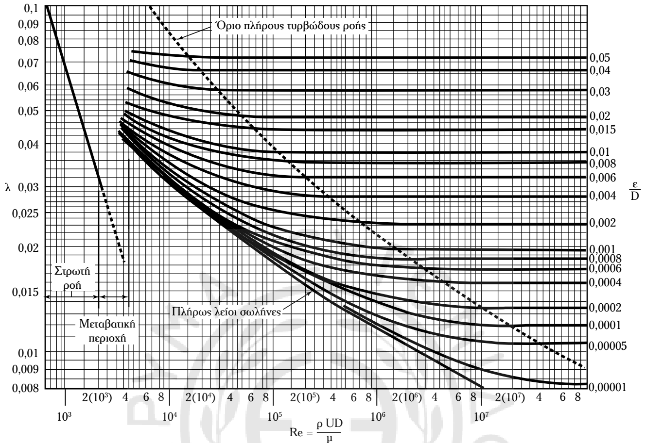
Σχ. Π.Β.1α Το διάγραμμα Moody.
