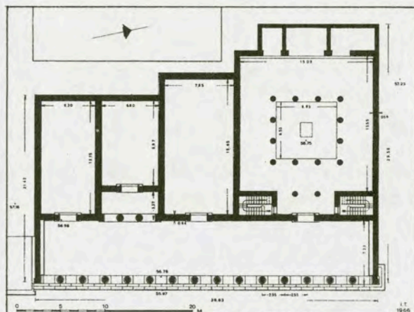
Κάτοψη του Μητρούου
