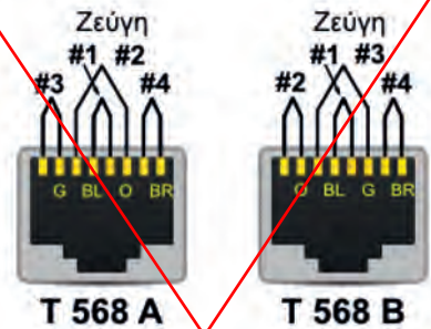
Εικόνα 2.4.1.α: Συρμάτωση
