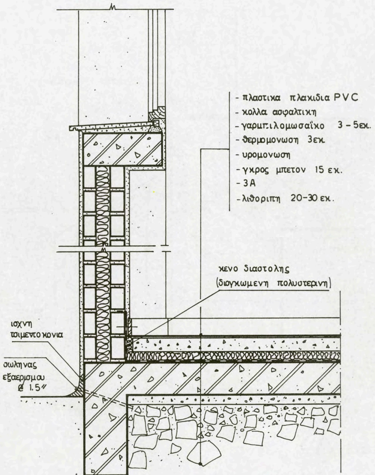
7.40. Λεπτομέρεια τομής κάτω από την ποδιά του παράθυρου. Δημιουργείται Εσοχή για την τοποθέτηση θερμαντικού σώματος (καλοριφέρ)
