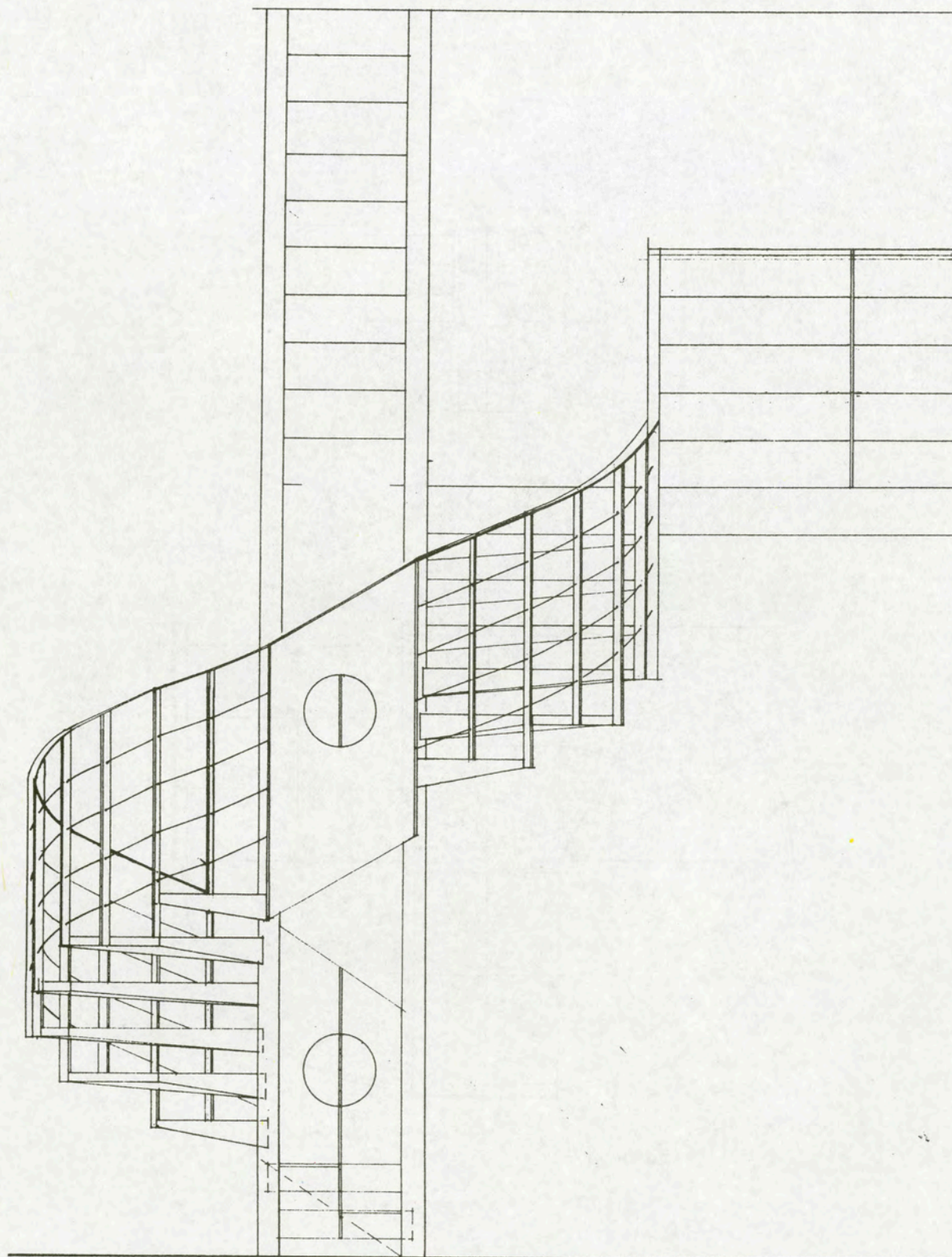
6.20.2. Όψη κλιμακοστάσιου
