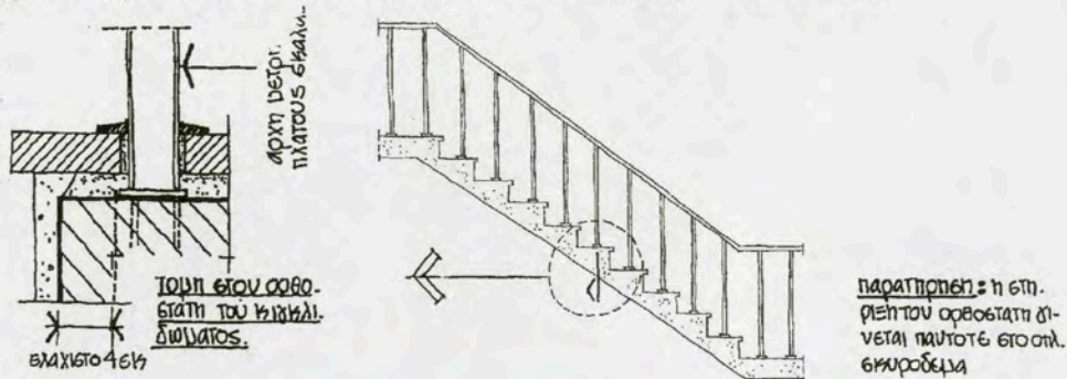
5.16.1. Κιγκλίδωμα στηριγμένο πάνω στα πατήματα
