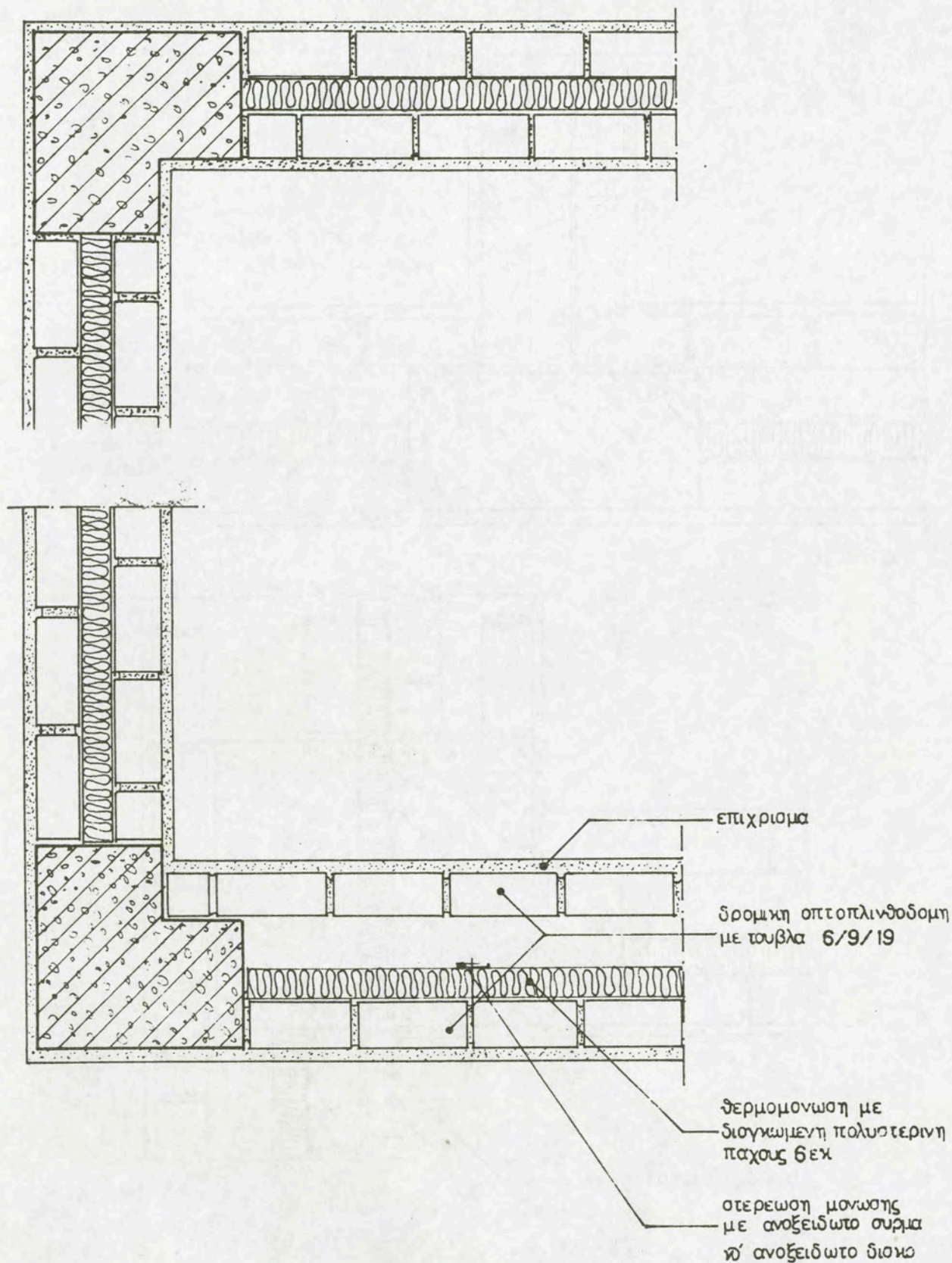
7.37. Λεπτομέρειες οπτοπλινθοδομών ( τούβλα ) σε κάτοψη
