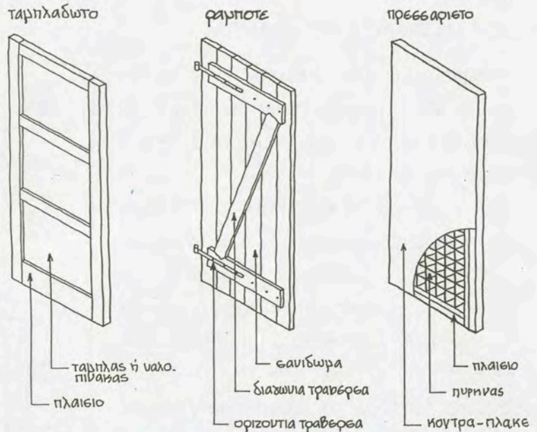
5.30. Τύποι φύλλου ξύλινης πόρτας
