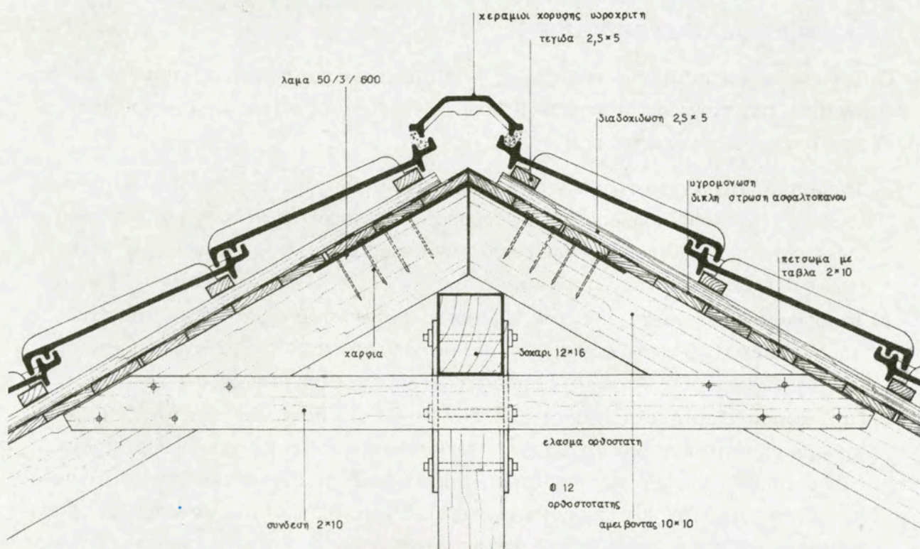
5.41.1.. Λεπτομέρεια Λ11: κορφιά
