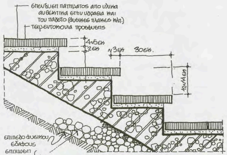
5.13. Λεπτομέρεια σκάλας κήπου
