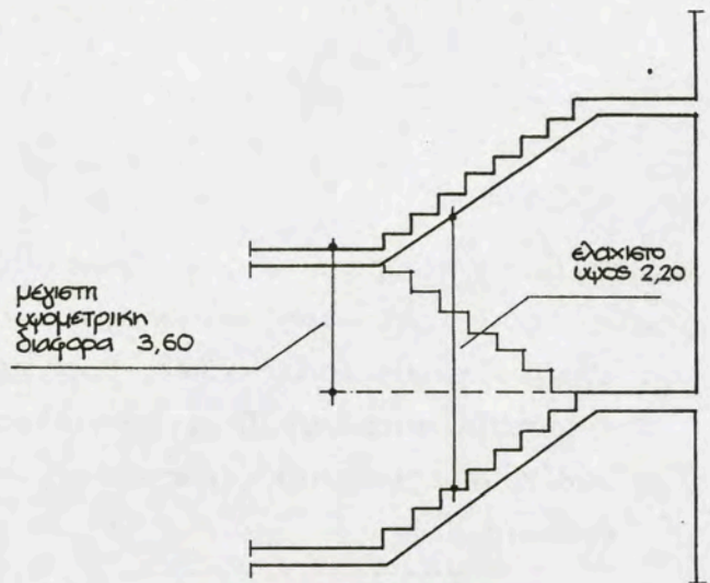
5.5. Τομή κλιμακοστασίου
