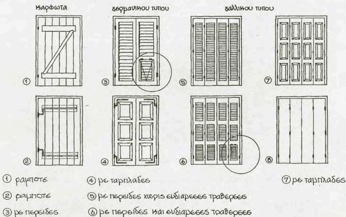
5.27. Τύποι ανοιγόμενων φύλλων παραθύρων
