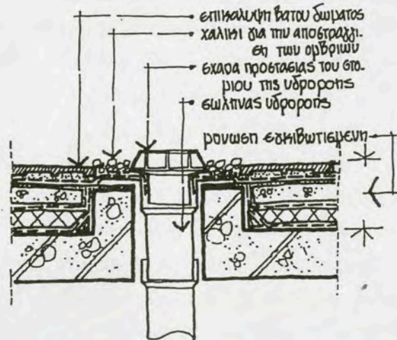
5.20.2. Διαμόρφωση θέσης εσωτερικής υδρορροής
