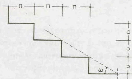
5.1. Τομή σκαλοπατιών
