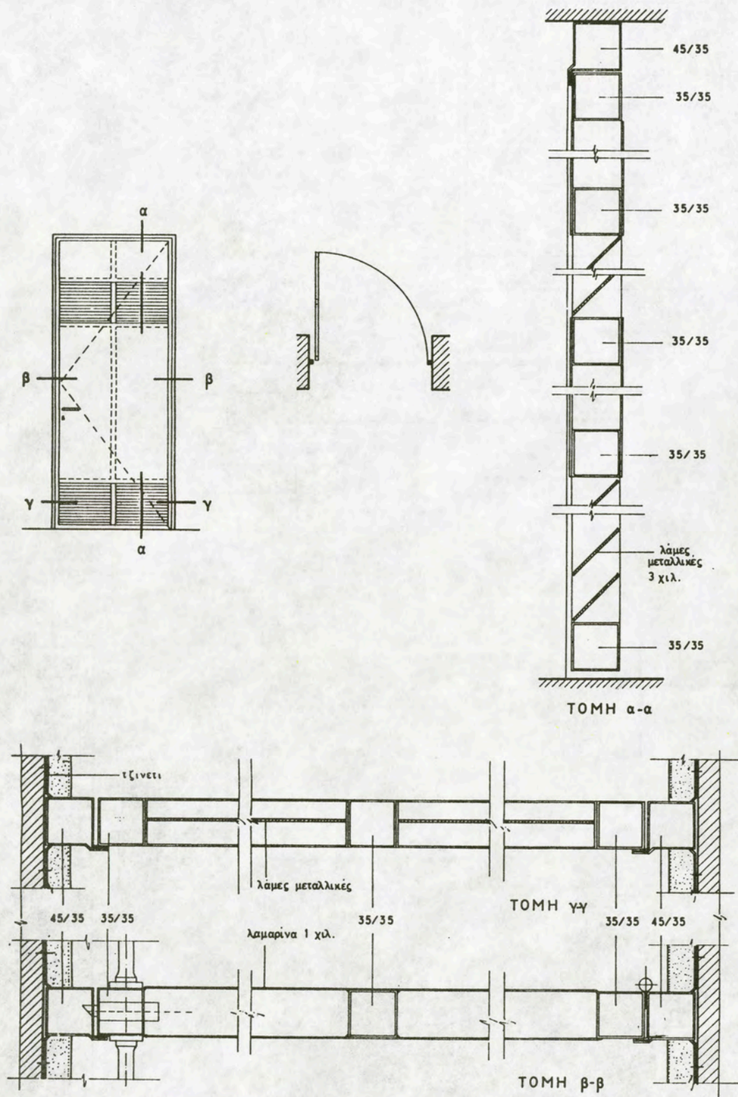
7.55. Λεπτομέρεια μονόφυλλης μεταλλικής πόρτας με περσίδες (γρίλλες) εξαερισμού
