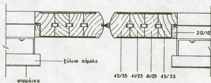
ΤΟΜΗ γ-γ
