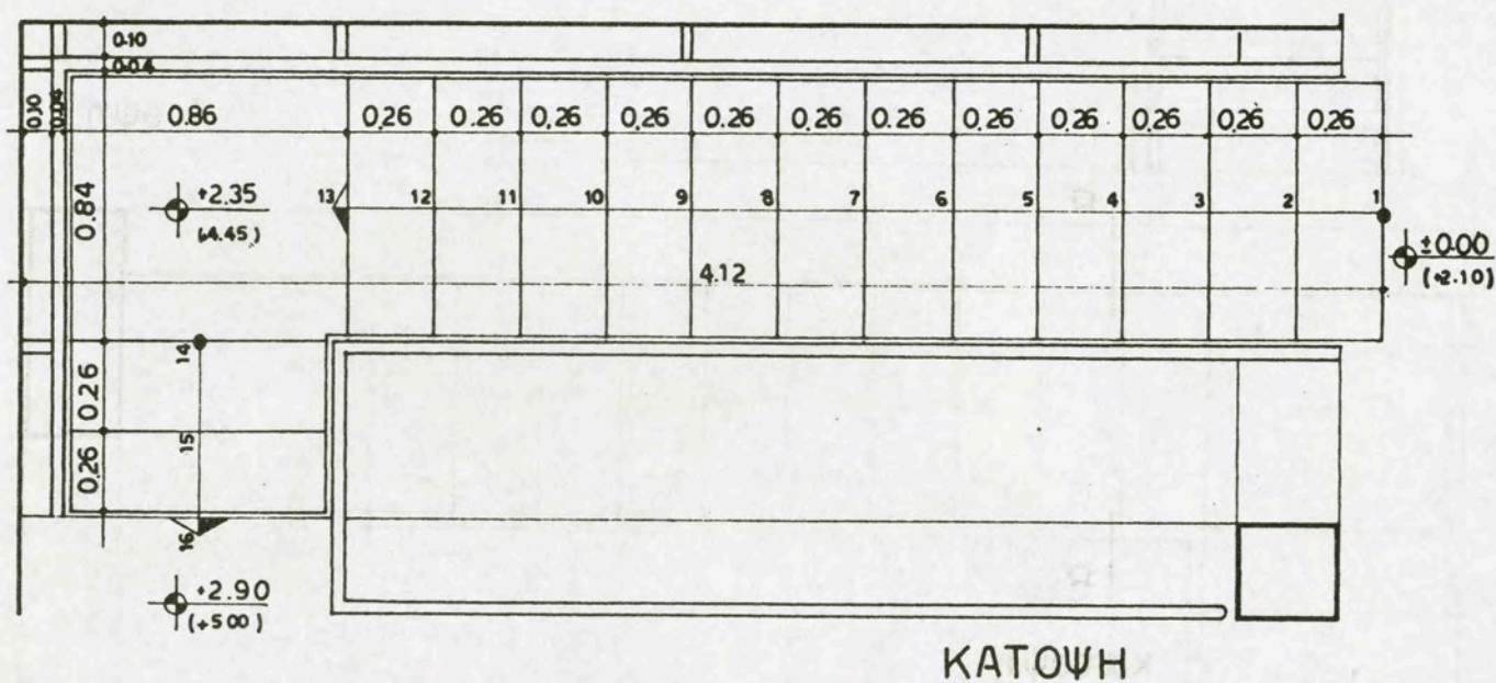
7.29. Κάτοψη- τομή ευθύγραμμης γωνιακής σκάλας (παραλλαγή)
