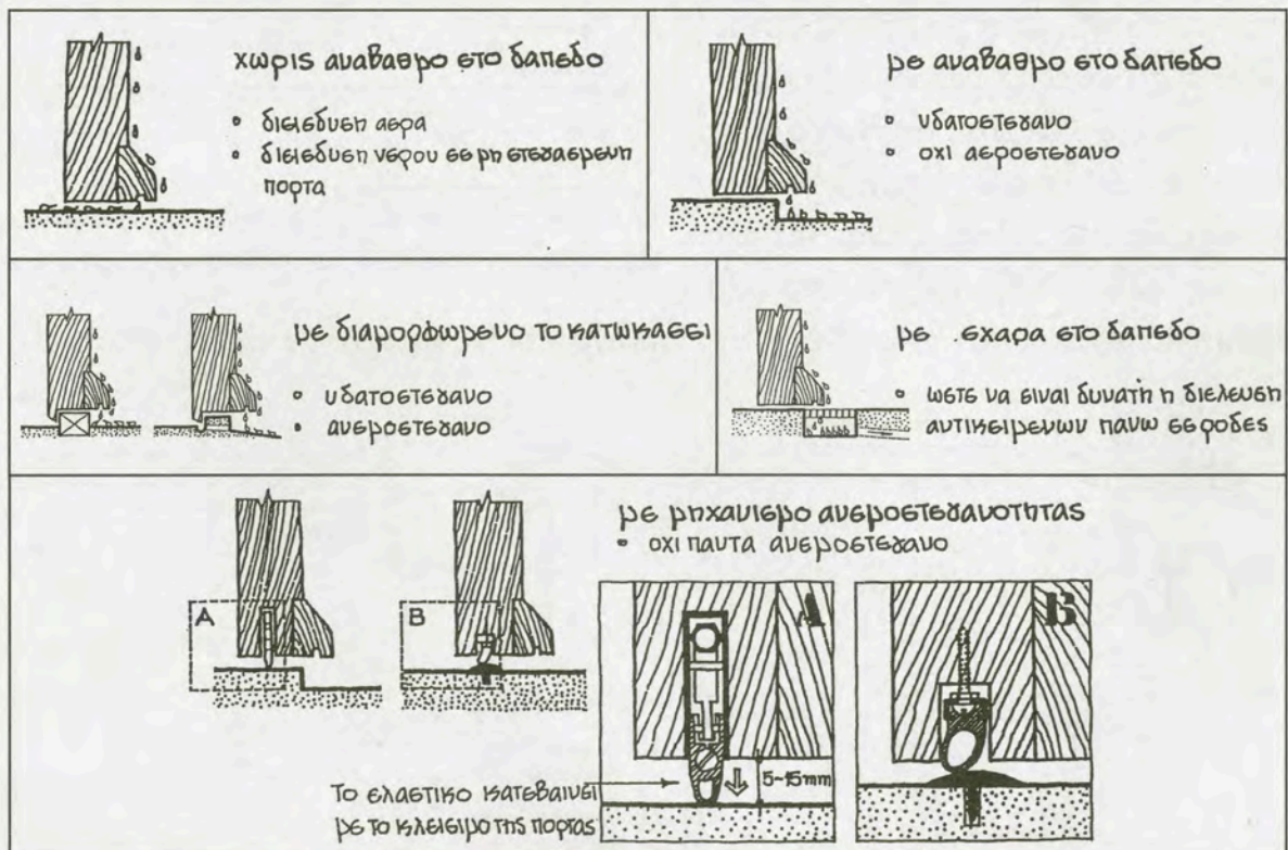
5.31. Τρόποι διαμόρφωσης κάτω τμήματος εξωτερικής πόρτας
