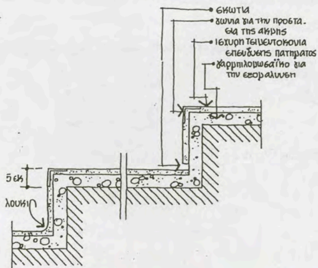
5.10. Λεπτομέρειες επένδυσης σκάλας με τσιμεντοκονία
