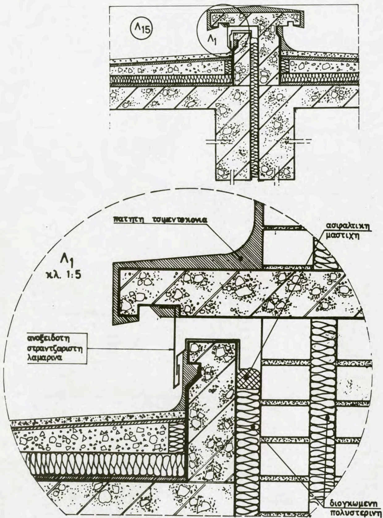
7.43. Λεπτομέρειες διαμόρφωσης οριζόντιων αρμών διαστολής
