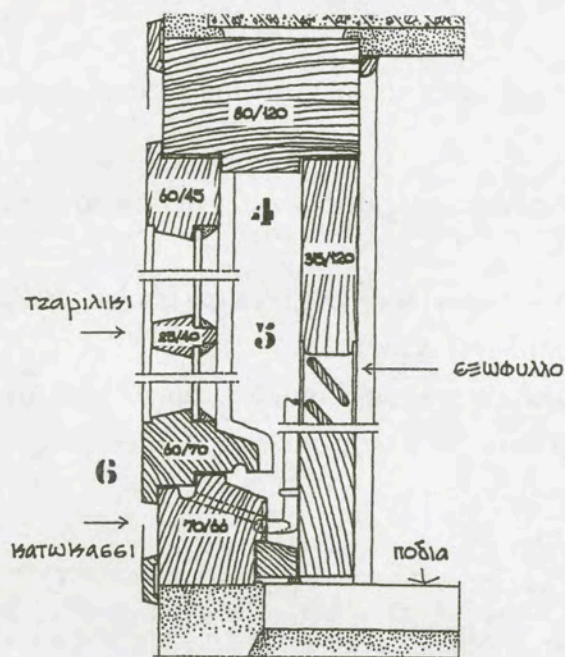
κατακόρυφη τομή ξύλινου παραθύρου.
