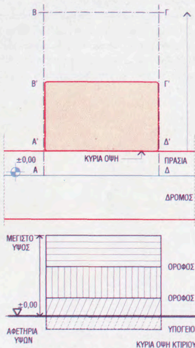
1.23. Τα στοιχεία του κτιρίου
