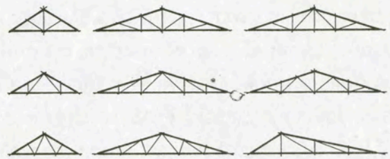
5.38. Διάφορες μορφές ζευκτών
