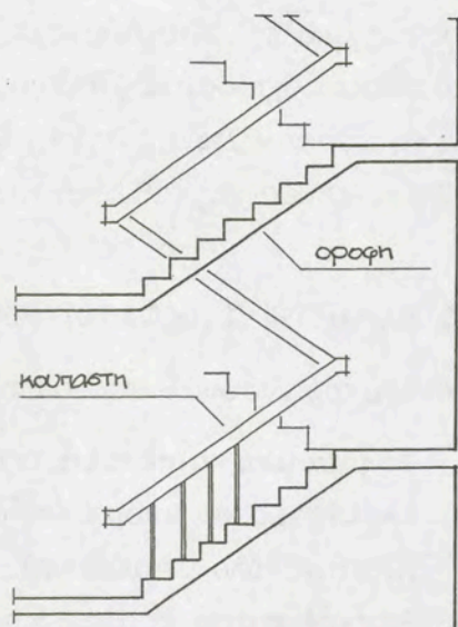
5.3.1. Τομή κλιμακοστασίου
