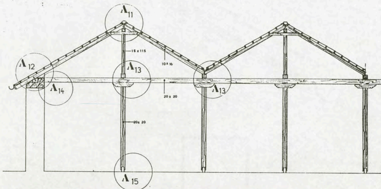
5.41. Τομή υπόστεγου που καλύπτεται από δίδυμη δώριχη στέγη.
