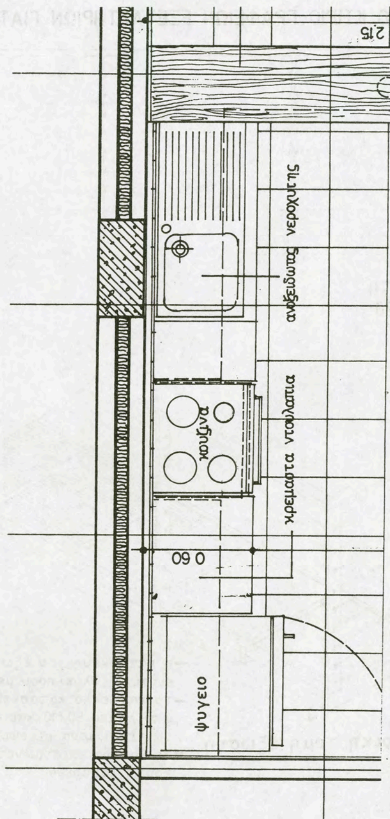
7.33. Κάτοψη παρασκευαστηρίου
