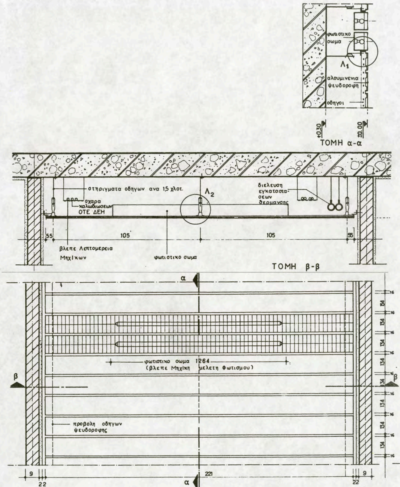
7.56. Λεπτομέρεια ( άνοψη και τομές ) προτεινόμενης ψευδοροφής
