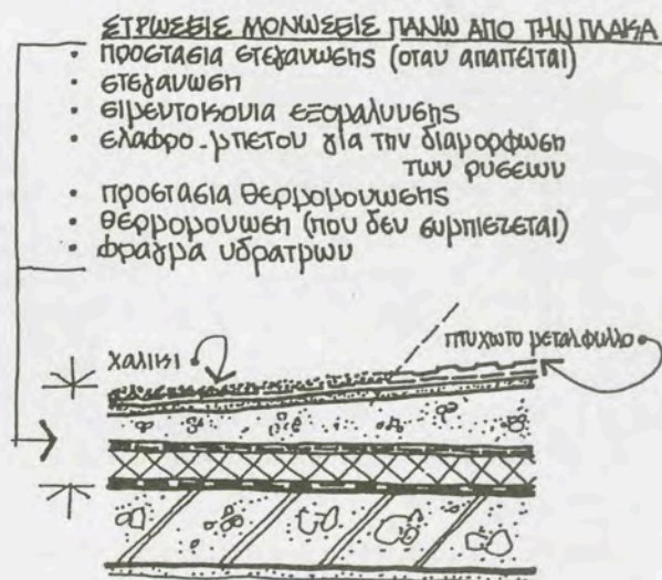
5.19.1. Συμβατική μόνωση σε μη βατό δώμα
