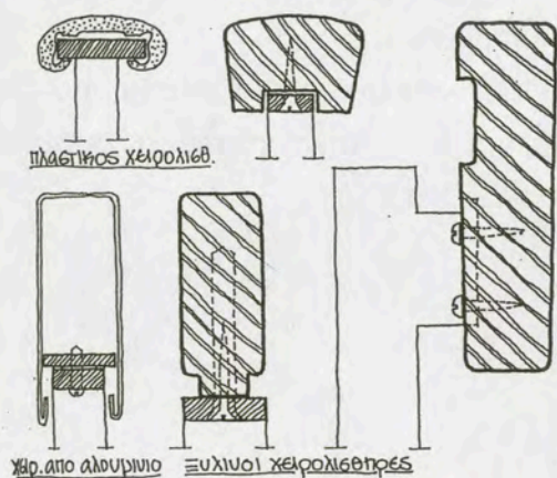
5.17. Διάφοροι τύποι χειρολισθήρων
