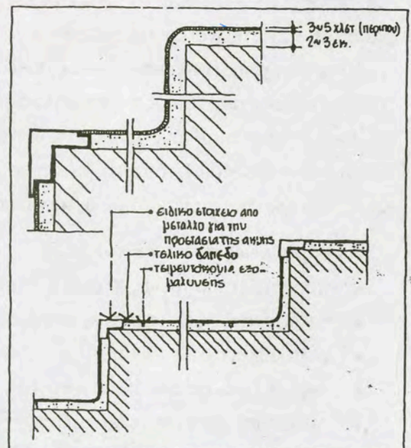
5.11:1. Επίστρωση πατημάτων με συνθετικά υλικά
