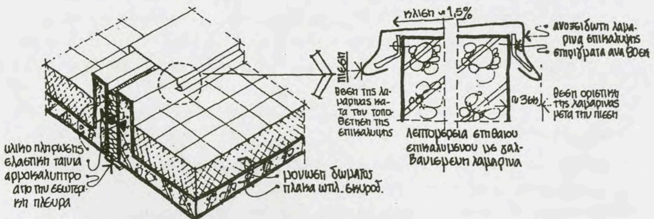
5.22. Τομή αρμού διαστολής
