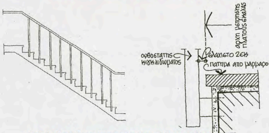
5.16.2. Κιγκλίδωμα στηριγμένο στο πλάι της σκάλας
