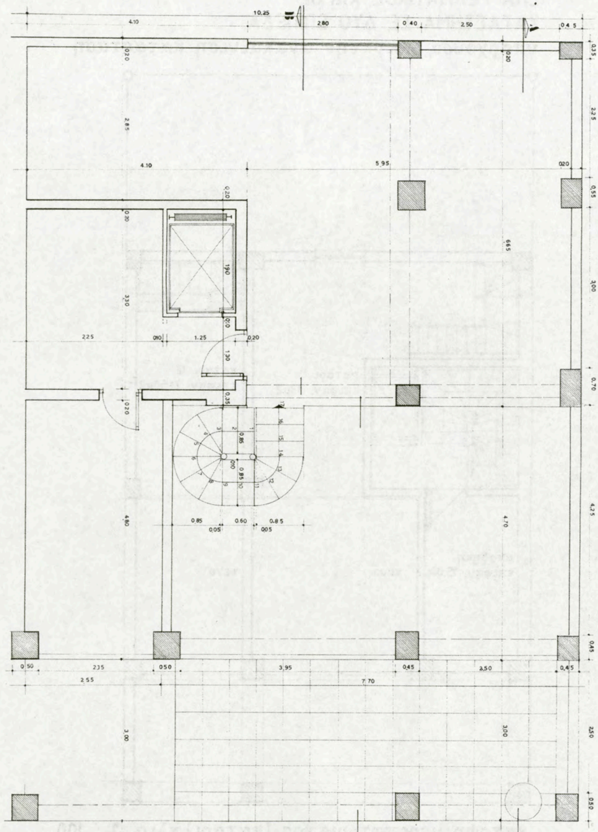
6.19.1. Κάτοψη ισόγειου
