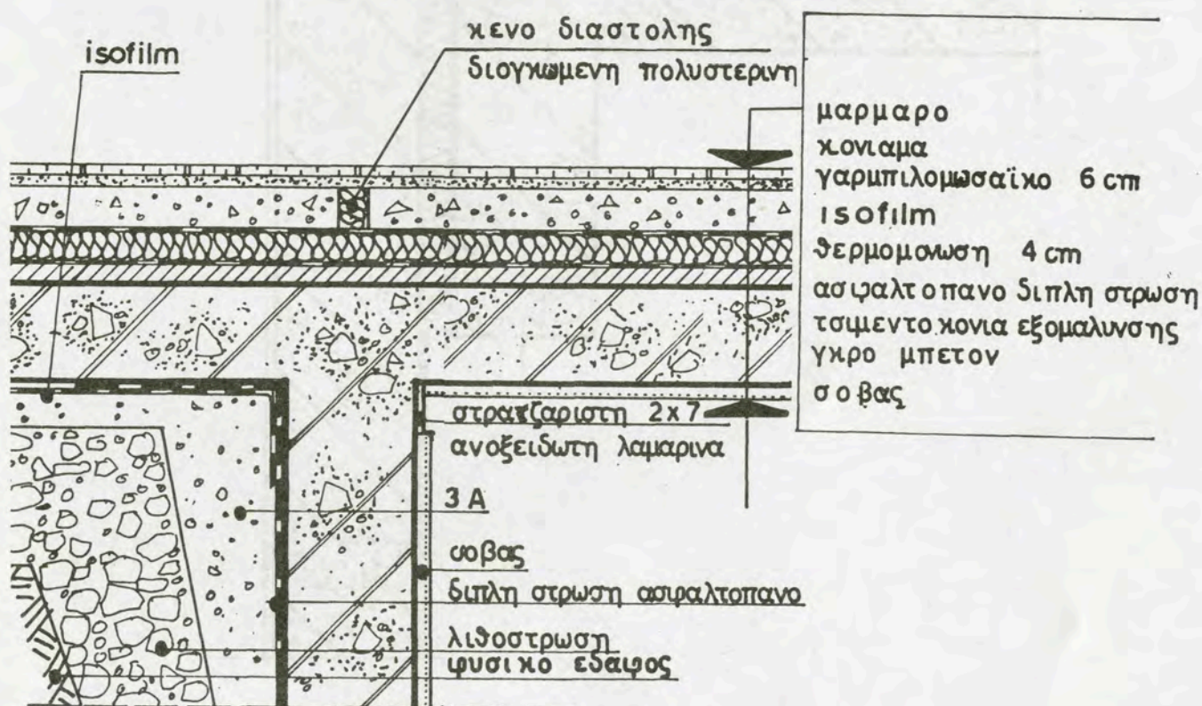
7.45. Λεπτομέρειες διάστρωσης δαπέδων εσωτερικού χώρου
