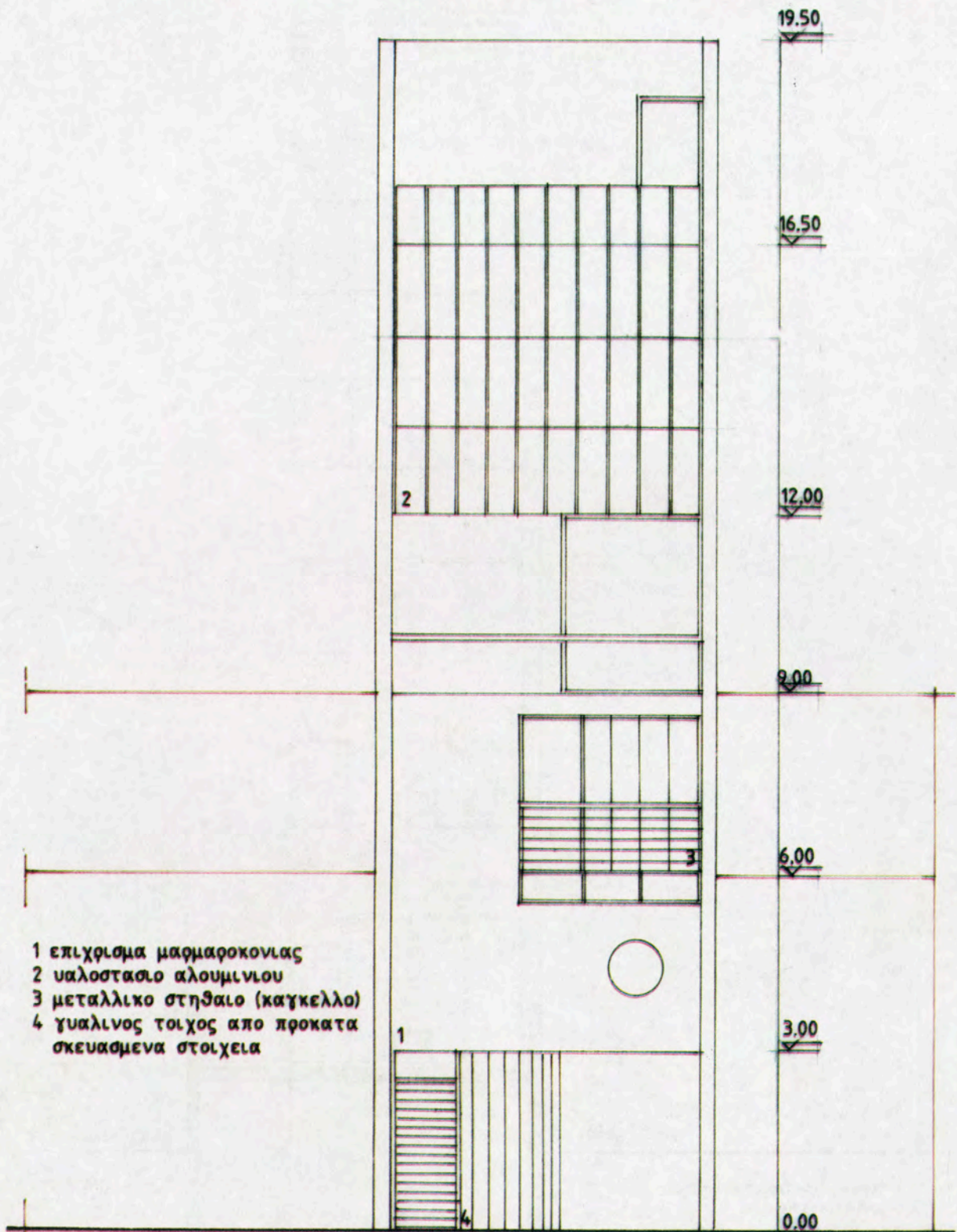
7.21. Όψη οδού Ευρώτα
