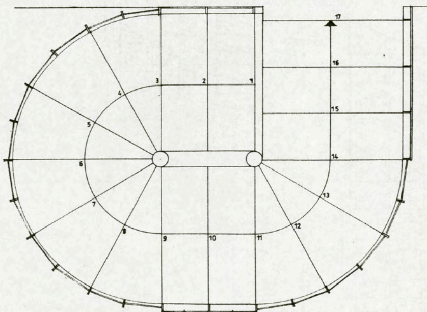
ΚΑΤΟΨΗ ΚΛ. 1: 10
