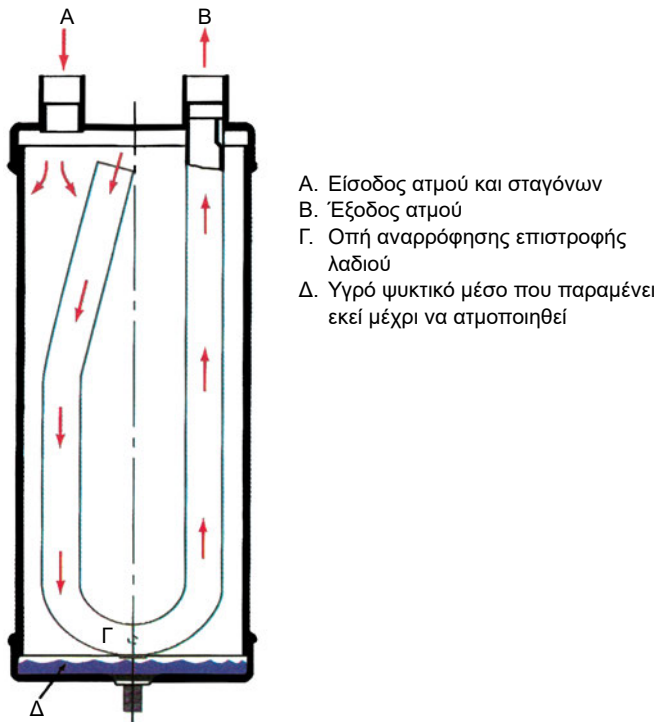
Σχήμα 6.21 Αρχή λειτουργίας παγίδας σταγόνων ψυκτικού μέσου
