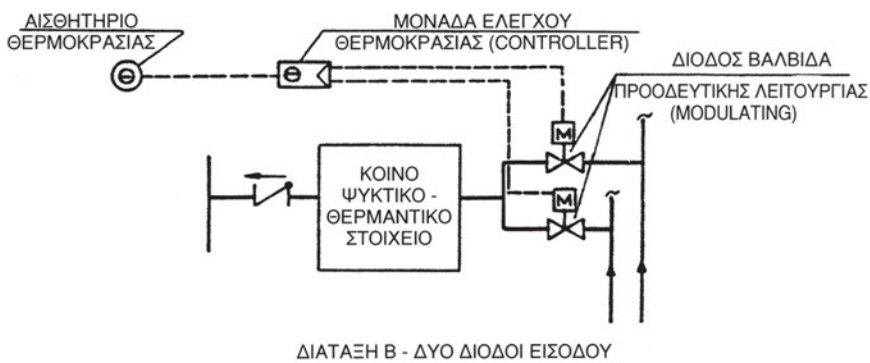
Σχήμα 9.11. Λειτουργία Συστήματος ΤΜΑΣ 3 σωλήνων
