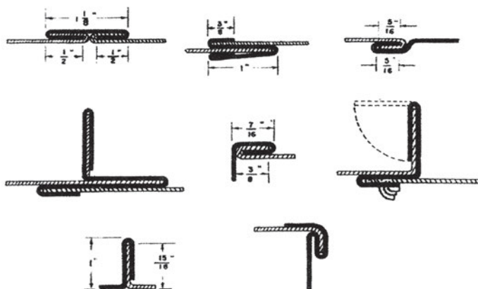
Σχήμα 12.3. Τρόποι σύνδεσης τμημάτων αεραγωγών από γαλβανισμένη λαμαρίνα
