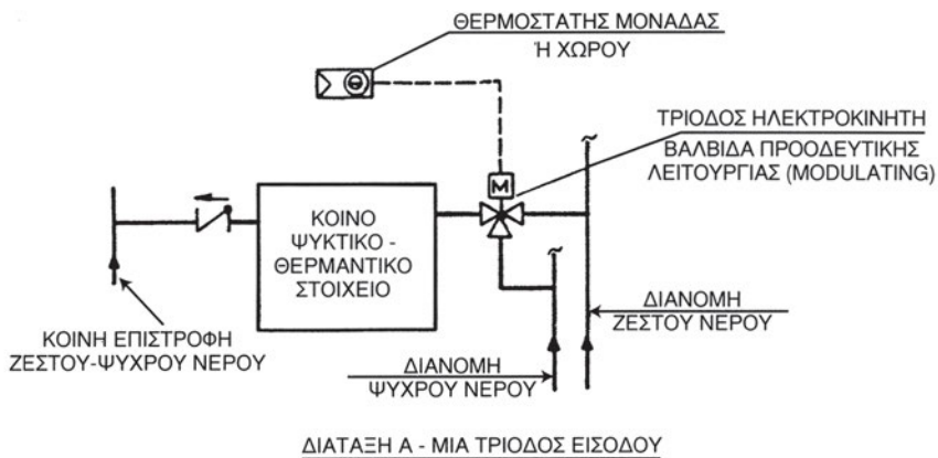
ΔΙΑΤΑΞΗ Α - ΜΙΑ ΤΡΙΟΔΟΣ ΕΙΣΟΔΟΥ
