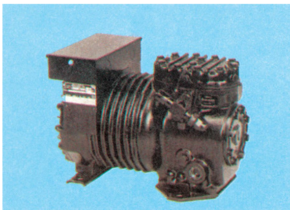
Εικόνα 6.10 Ημιερμητικός συμπιεστής
