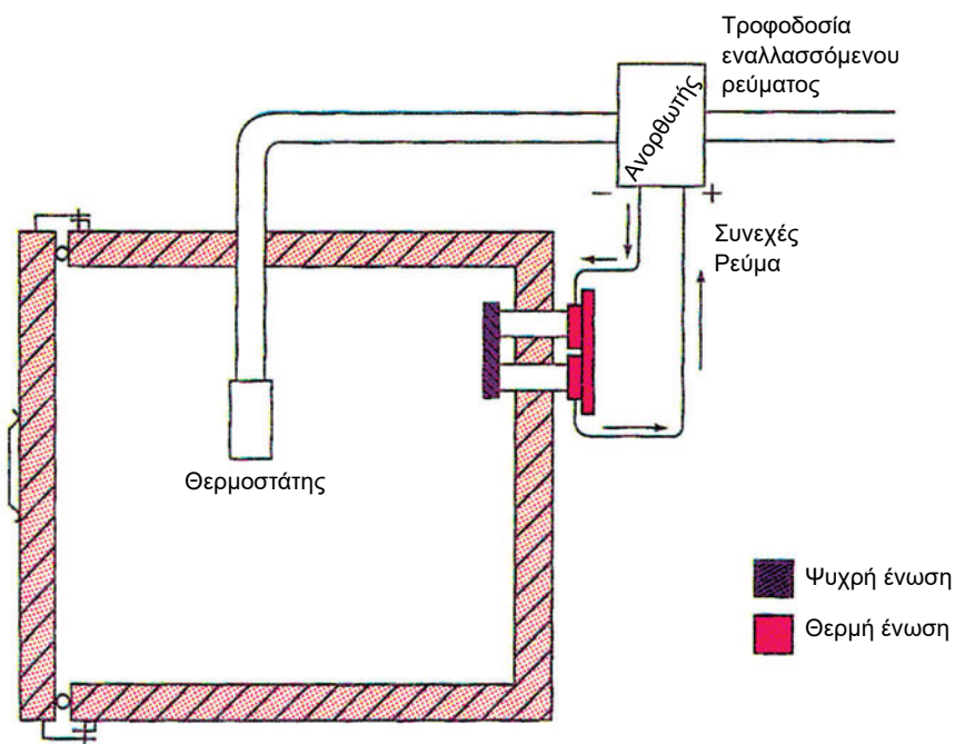
Σχήμα 7.4 Θερμοηλεκτρική ψύξη
