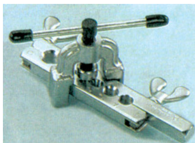
Εικόνα 6.1 Εργαλείο εκχείλωσης
