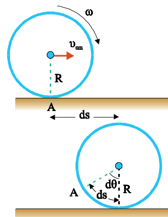
Όταν το κέντρο μάζας του τροχού μετακινηθεί κατά ds , κάθε σημείο στην περιφέρειά του στρέφεται κατά το ίδιο τόξο.
