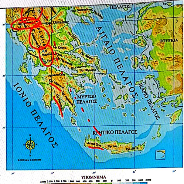
Εικόνα 13.2: Γεωμορφολογικός χάρτης της Ελλάδας
