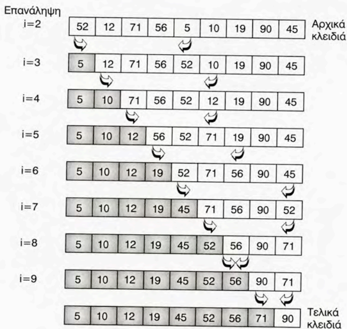
Σχήμα 3.2. Ταξινόμηση ευθείας επιλογής.
