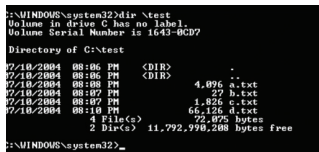
Εικόνα 3.2. Επικοινωνία με απευθείας εντολές (Λ.Σ. MS DOS)
