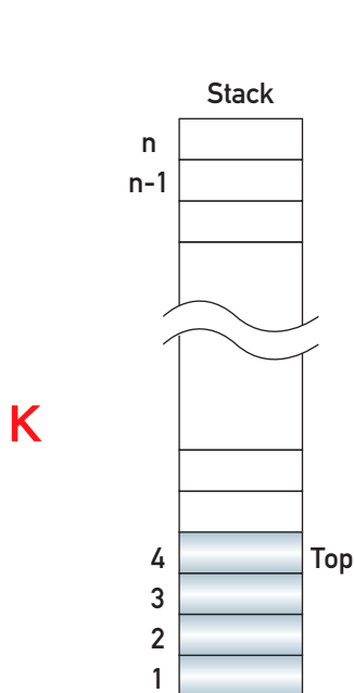
Σχ. 3.3 Υλοποίηση στοίβας με χρήση πίνακα
