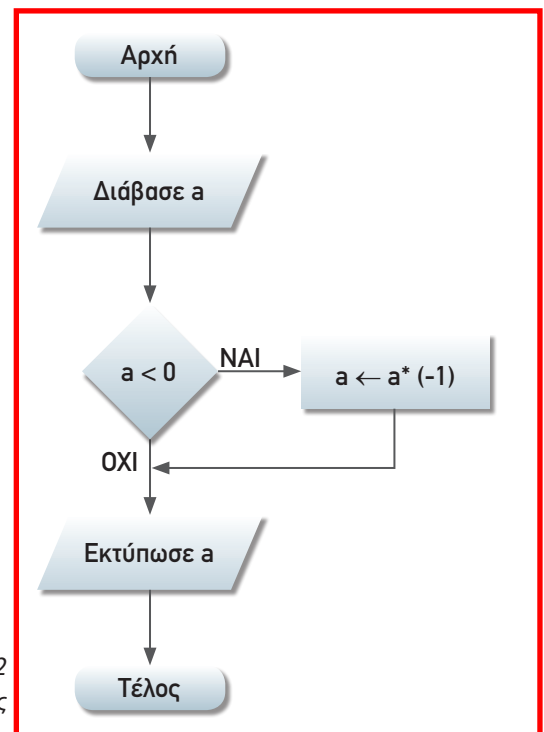
Σχ. 2.2. Ο αλγόριθμος του παραδείγματος 2 με διάγραμμα ροής
