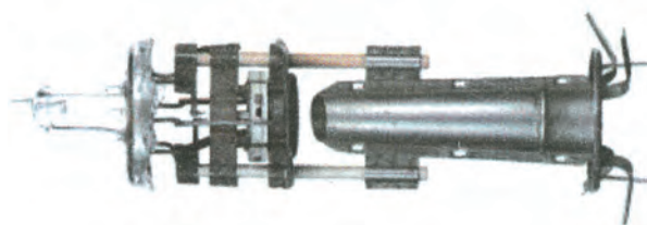
Εικ. 5.3 Τηλεβόλο ηλεκτρονίων.
