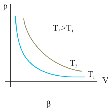
Σχ. 3.1 α) Το αέριο βρίσκεται μέσα σε ογκομετρικό δοχείο. Το δοχείο με το αέριο περιβάλλεται από λουτρό με νερό του οποίου η θερμοκρασία διατηρείται σταθερή. Στο δοχείο υπάρχει προσαρμοσμένο μανόμετρο για τη μέτρηση της πίεσης του αερίου. β) Στο διάγραμμα παριστάνεται γραφικά η πίεση του αερίου σε συνάρτηση με τον όγκο του, για θερμοκρασίες T_1 και T_2 για τις οποίες ισχύει T_2 > T_1 .
