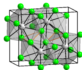
Κρυσταλλική δομή του υδριδίου του ασβεστίου, \text{CaH}_2 .
