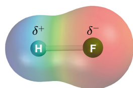
Κατανομή ηλεκτρικού φορτίου στο μόριο του HF.
