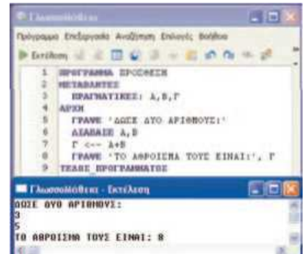
Εικόνα 1.4. Ο κώδικας για την άθροιση δύο αριθμών στο προγραμματιστικό περιβάλλον Γλωσσολόγιο.
