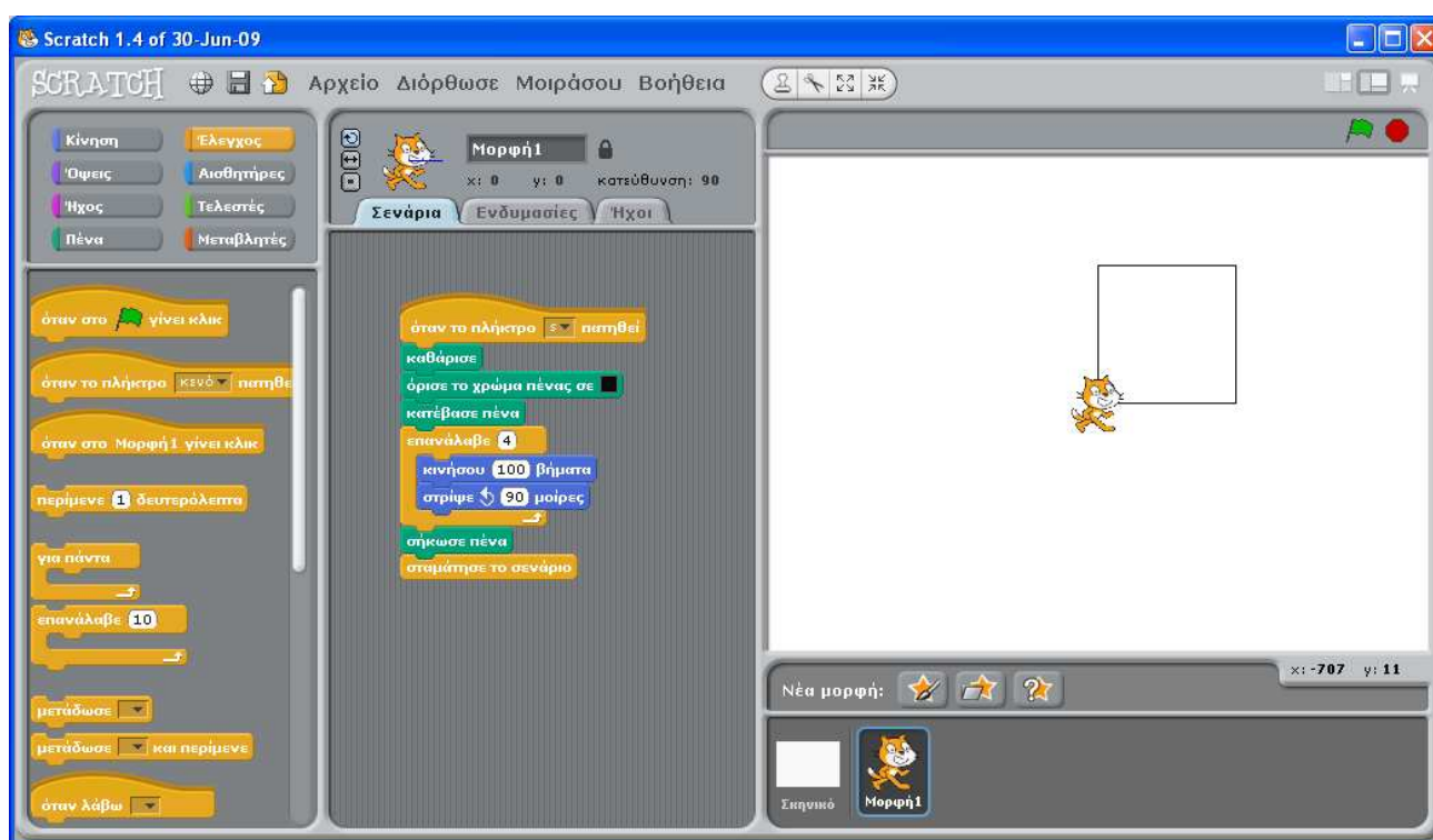
Εικόνα 2.5. Το σενάριο s έχει δημιουργήσει ένα τετράγωνο
