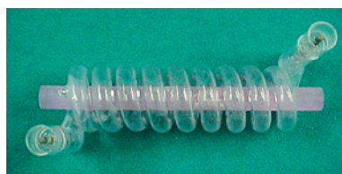
Εικόνα 2.18 Ράβδος YAG με το σύστημα σωλήνα ψύξης της από Λείζερ Nd:YAG.
