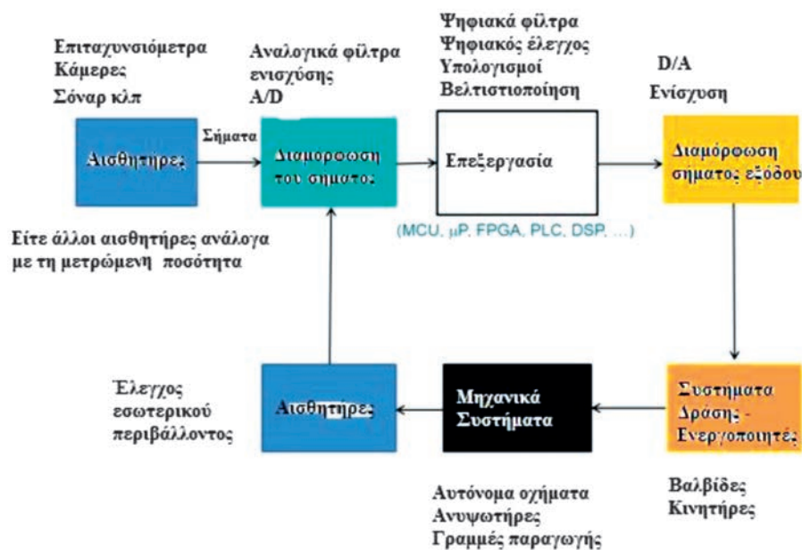
Εικόνα 3. Διάγραμμα μηχανικού συστήματος
