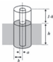
Εικόνα 20. Χωρητικός αισθητήρας στάθμης
