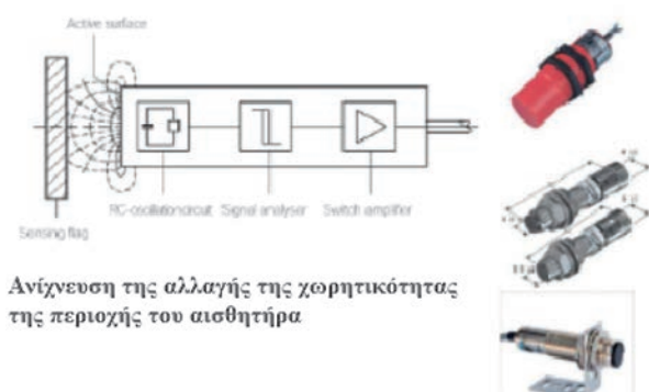
Εικόνα 15. Χωρητικός αισθητήρας
