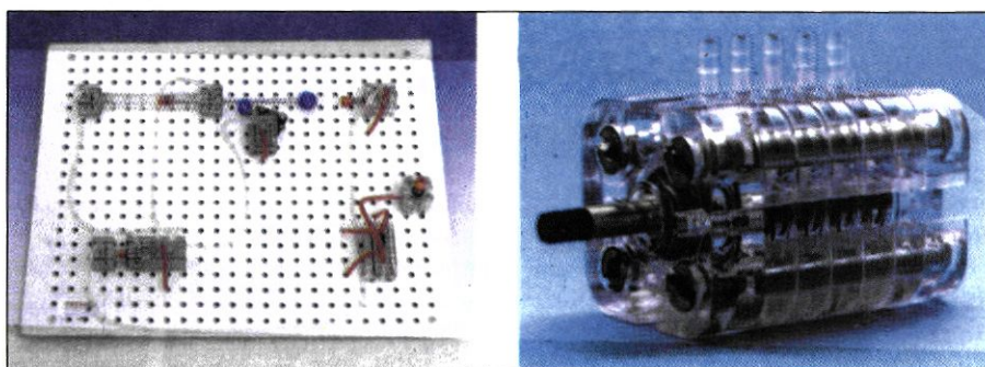
Εικ. 2.9. Μονάδα (Module) «πνευματικού» συστήματος που σταματά και ξεκινά τη ροή του αέρα.
