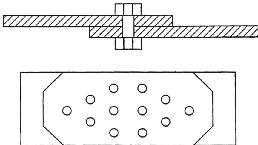
Εικ.1.6. Έλεγχος αντοχής συνδέσμων με ηλώσεις.
