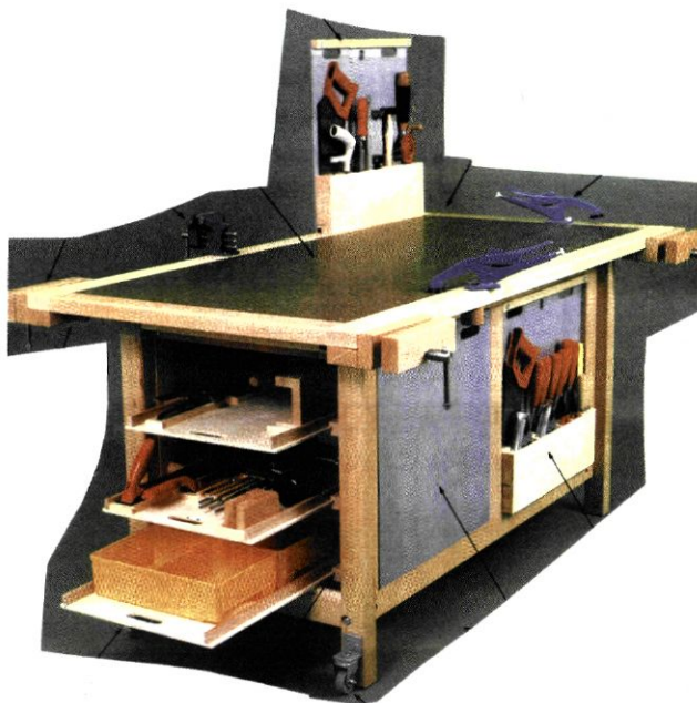
Εικ. 2.1. Πάγκος εργασίας και βασικά εργαλεία.
