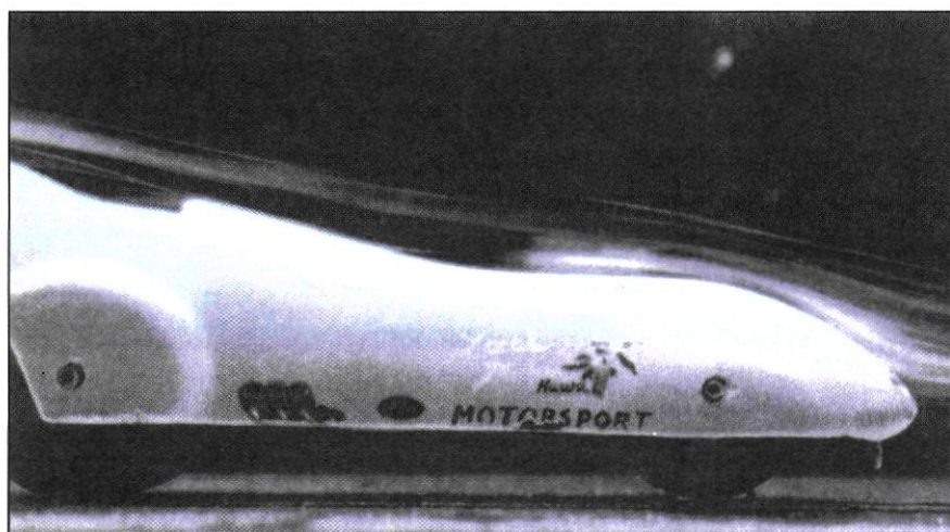
Εικ. 1.2. Έρευνα της αντίστασης σε αέρα σχημάτων διαφόρων μοντέλων αυτοκινήτων.
