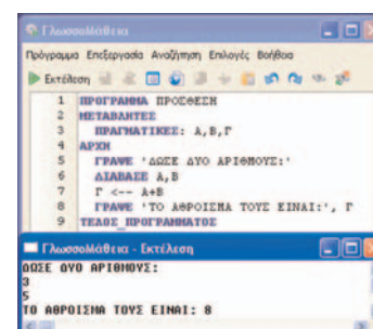
Εικόνα 1.4. Ο κώδικας για την άθροιση δύο αριθμών στο προγραμματιστικό περιβάλλον Γλωσσολόγος
