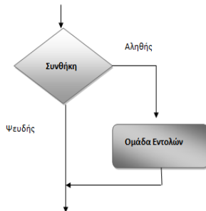
Εικόνα 4-1. Διάγραμμα ροής για τη δομή επιλογής if...else (AN...ΑΛΛΙΩΣ)
