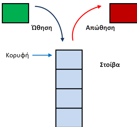
Εικόνα 8-1. Οι βασικές λειτουργίες σε μια στοίβα είναι η ώθηση και η απώθηση
