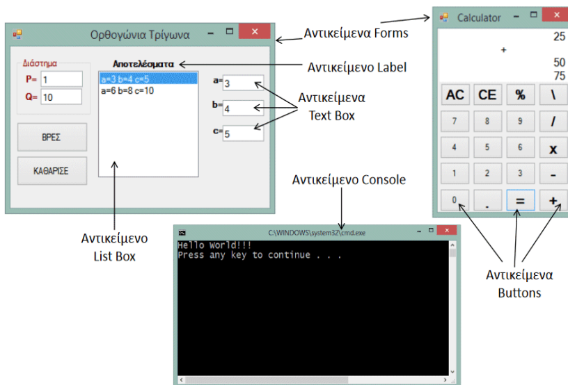
Εικόνα 2-5. Προγραμματιστικά αντικείμενα
