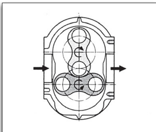
Εικόνα 2.5.2 Ελικοειδής υπερσυμπίεστής
