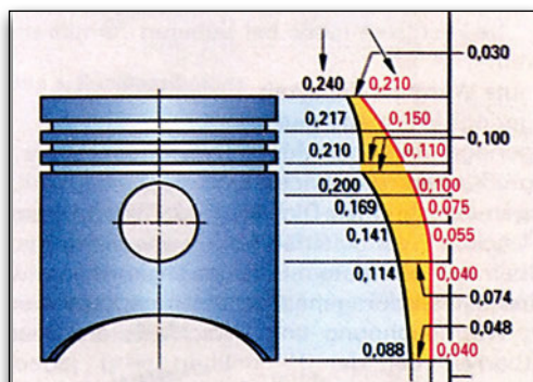
Εικόνα 2.2.5 Κατασκευαστικές λεπτομέρειες εμβόλου
