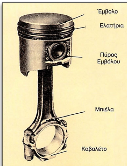
Εικόνα 2.2.4 Έμβολο με ελατήρια.
