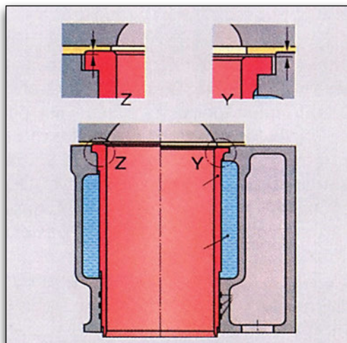
Εικόνα 2.2.3 Τοποθέτηση χιτώνιου σε κινητήρα
