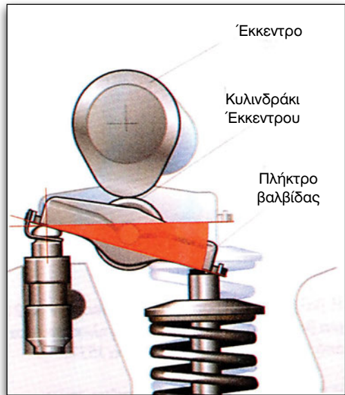
Εικόνα 2.3.4 Εκκεντροφόρος επικεφαλής, επιδρά στη βαλβίδα μέσω ζυγώθρου
