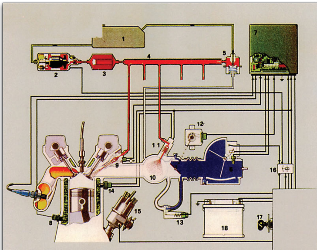
Εικόνα 3.1.50 Συνδεσμολογία L-Jetronic
