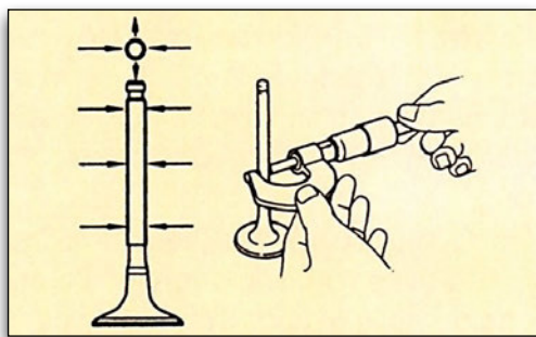
Εικόνα 2.1.9 Μέτρηση βαλβίδας
