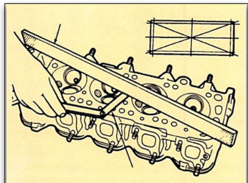
Εικόνα 2.1.3 Έλεγχος επιπεδότητας
