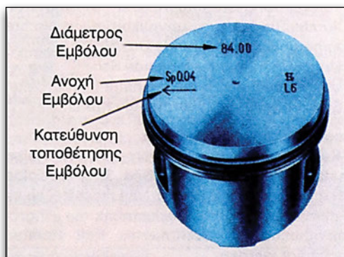
Εικόνα 2.2.6 Χαρακτηριστικά εμβόλου
