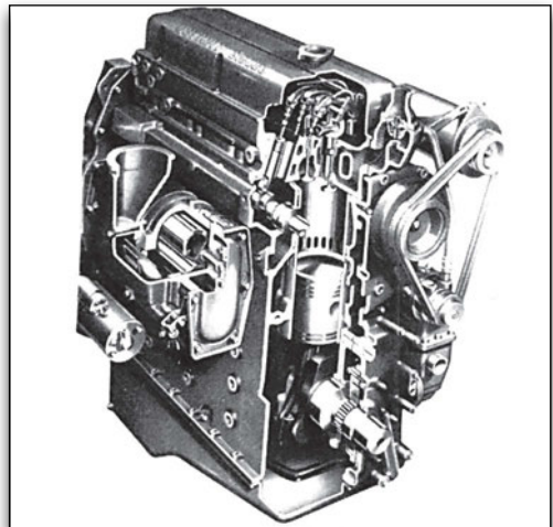
Εικόνα 1.2.13 Δίχρονες πετρελαιομηχανές
