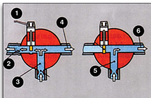
Εικόνα 2.5.8 Στιγμαία υπερπλήρωση (Overboost)
