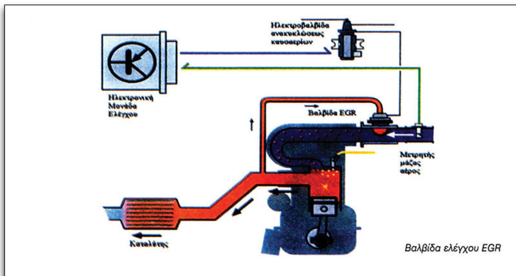
Εικόνα 4.1.8 Ανακυκλοφορία καυσαερίων
