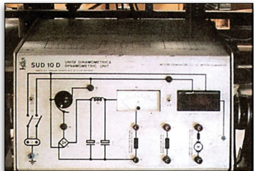
Εικόνα 1.3.4 Συσσκευές ηλεκτρικών δυναμοδεικτών και δυναμομέτρων κινητήρων
