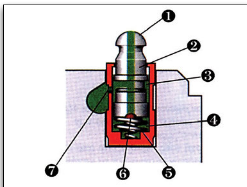
Εικόνα 2.3.2 Υδραυλικό ωστήριο
