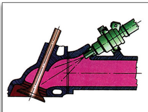
Εικόνα 3.1.1 Μπεκ βενζίνης
