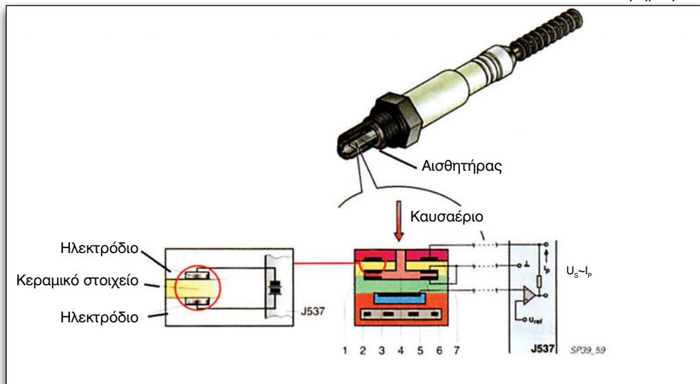
Εικόνα 4.2.13 Αισθητήρας “λ”.
