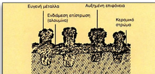
Εικόνα 4.2.8 Επίστρωση αλουμίνας.
