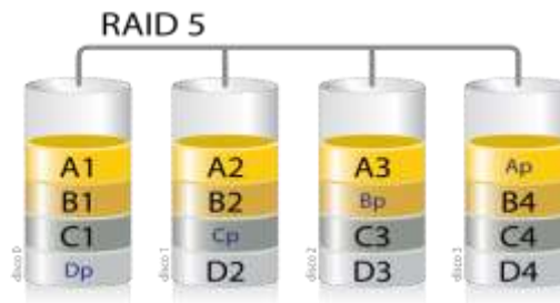
Εικόνα 3.5. Συστοιχία RAID 5.
