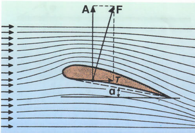
Εικόνα 7.59: Η εμφάνιση της δυναμικής άνωσης
