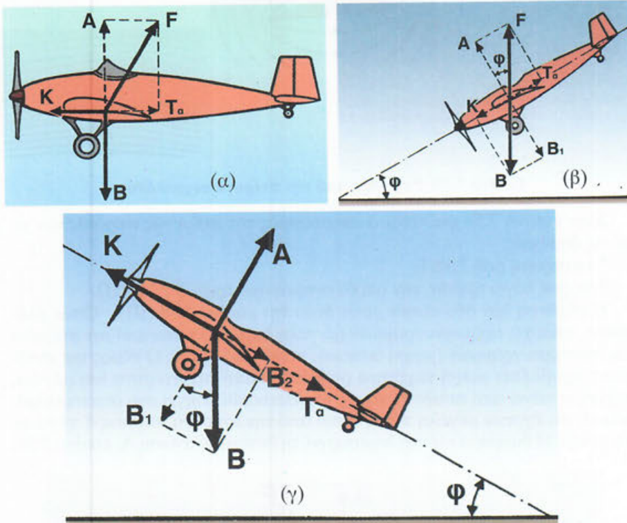
Εικόνα 7.60: Στρατιωτικό αεροπλάνο στις τρεις φάσεις πτήσης του
