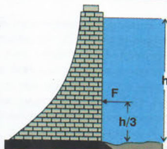
Εικόνα 7.21: Φράγμα
