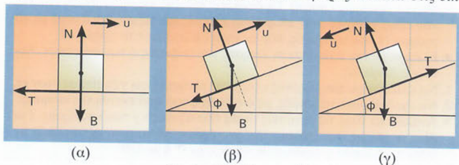
Εικόνα 5.12: Έργο τριβής
