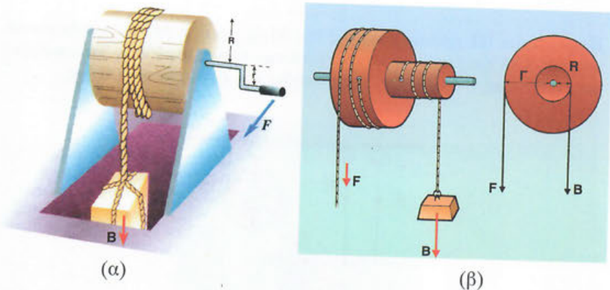
Εικόνα 5.10: Το βαρούλκο
