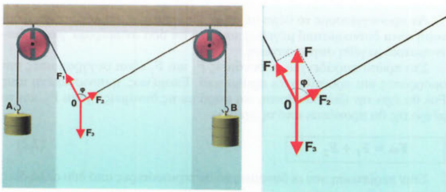
Εικόνα 2.24 Πείραμα με νήμα και με βάρη.
