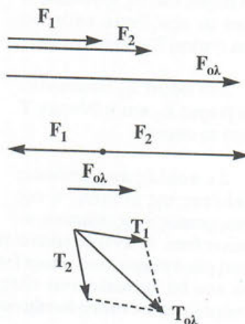
Εικόνα 2.23 Ρυμούλκηση πλοίου
