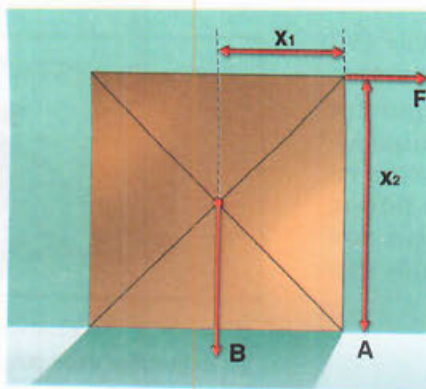
Εικόνα 3.20 Ισορροπία κιβωτίου
