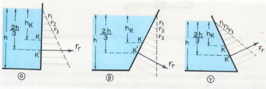
Εικόνα 7.18: Κατανομή δυνάμεων σε πλευρικό τοίχωμα
