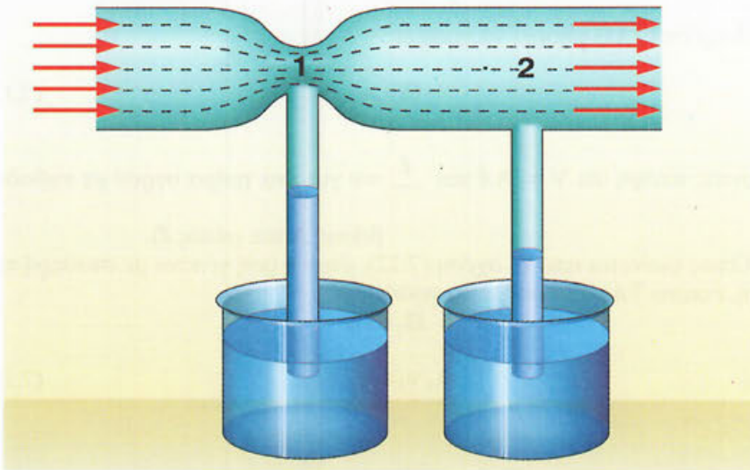
Εικόνα 7.42: Πειραματική επιβεβαίωση του νόμου Bernoulli
