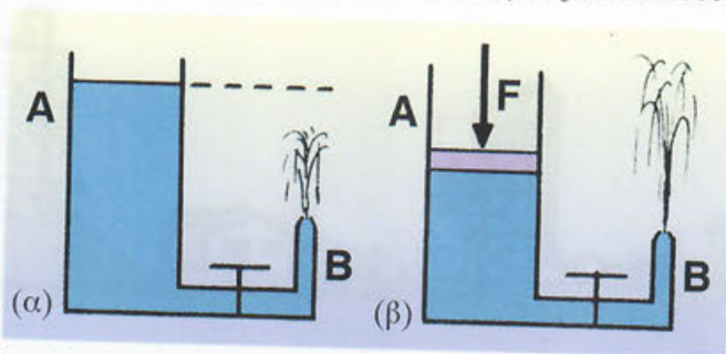
Εικόνα 7.7: Δημιουργία πίδακα ανθόρμητα(α) ή με εξαναγκασμό(β)
