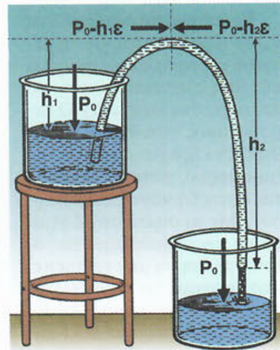
Εικόνα 7.32: Ο σίφωνας
