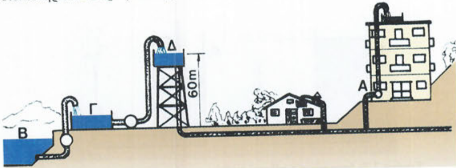
Εικόνα 7.9: Δίκτυο ύδρευσης
