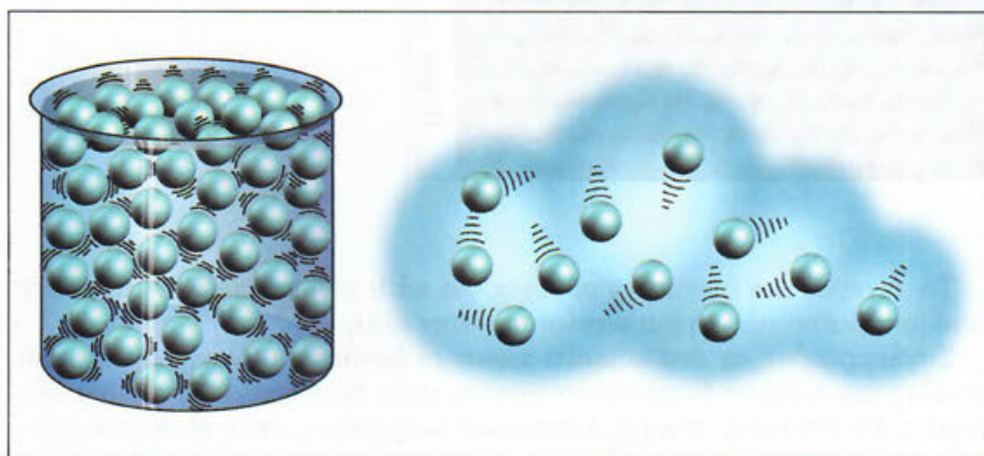
Εικόνα 2.13 Κινήσεις των μορίων στα ρευστά: (α) σε υγρό, (β) σε αέριο
