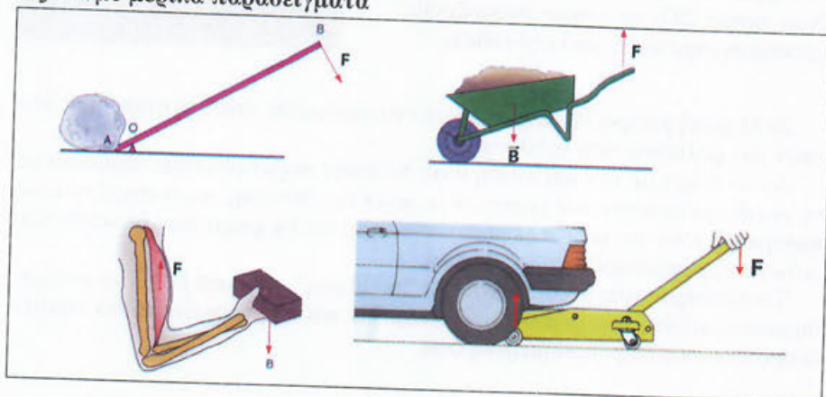
Εικόνα 3.5 Παραδείγματα περιστροφής σωμάτων
