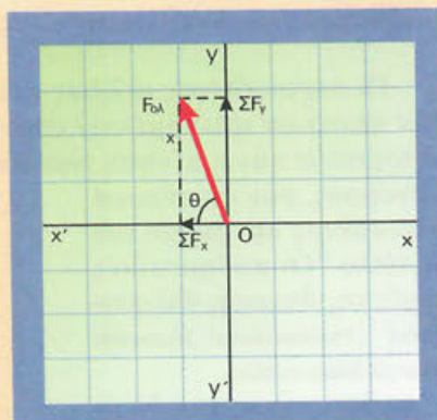
Εικόνα 2.30 Συνισταμένη τριών δυνάμεων.
