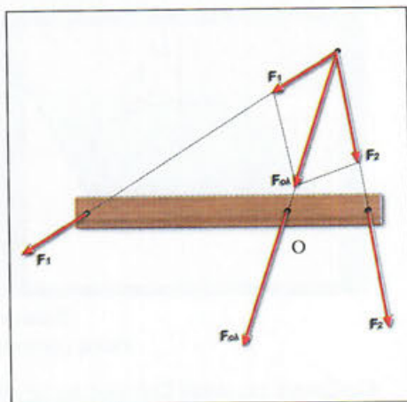
Εικόνα 3.11 Ισορροπία στερεού με την επίδραση δύο δυνάμεων
