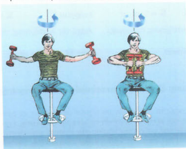
Εικόνα 6.19: Για την επιβεβαίωση της διατήρησης της στροφορμής
