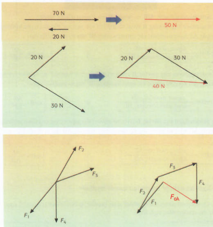
Εικόνα 1.14 Σύνθεση διανυσματικών μεγεθών
