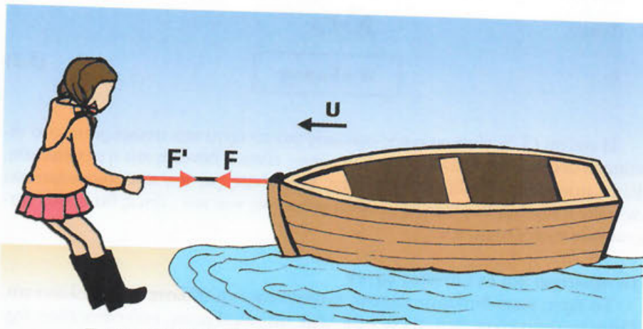
Εικόνα 5.2: Έργο δύναμης συγγραμμικής με τη μετατόπιση
