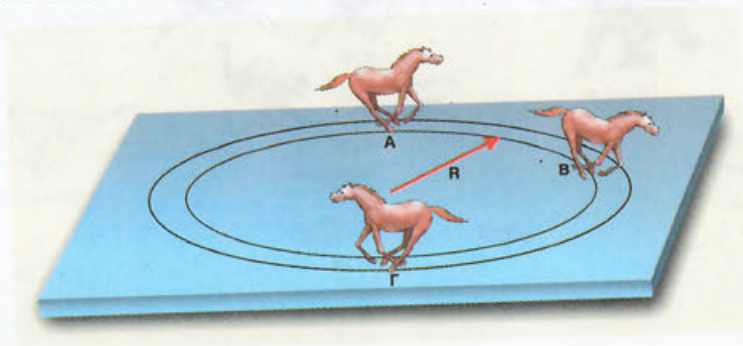
Εικόνα 4.19 Κυκλική κίνηση αλόγου
