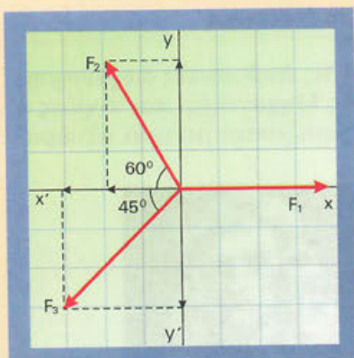
Εικόνα 2.30 Συνισταμένη τριών δυνάμεων.
