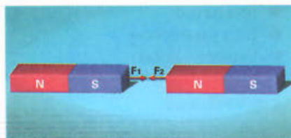
Εικόνα 2.34 Δράση-αντίδραση σε μαγνήτες
