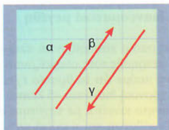
Εικόνα 1.11 Συγγραμμικά διανύσματα
