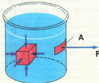
Εικόνα 7.3: Πίεση σε επιφάνεια
