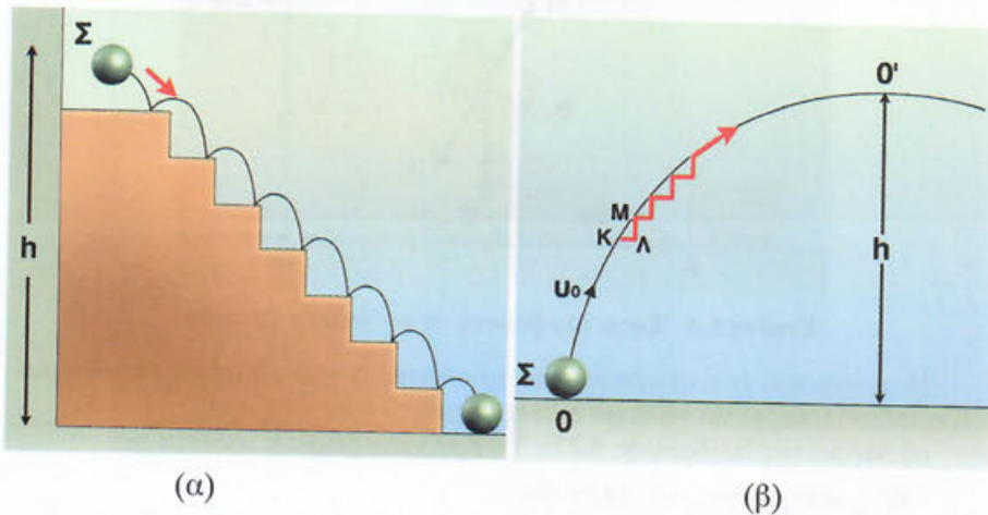
Εικόνα 5.5: Το βάρος παράγει και καταναλώνει έργο.
