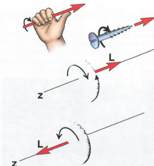
Εικόνα 6.16: Για τον προσδιορισμό του διανύσματος της στροφορμής
