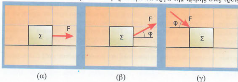
Εικόνα 5.13: Η τιμή της δύναμης τριβής εξαρτάται και από τον προσανατολισμό της δύναμης που ασκούμε στο σώμα.
