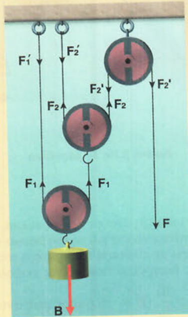
Εικόνα 5.11: Υπολογισμός δυνάμεων στο πολύσπαστο
