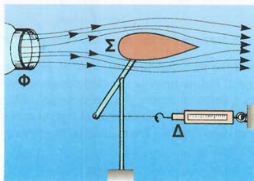
Εικόνα 7.53: Για τη μέτρηση της αντίστασης του αέρα
