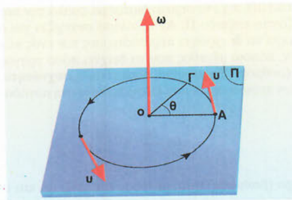
Εικόνα 6.1.(α): Για τη μελέτη της ομαλής κυκλικής κίνησης
