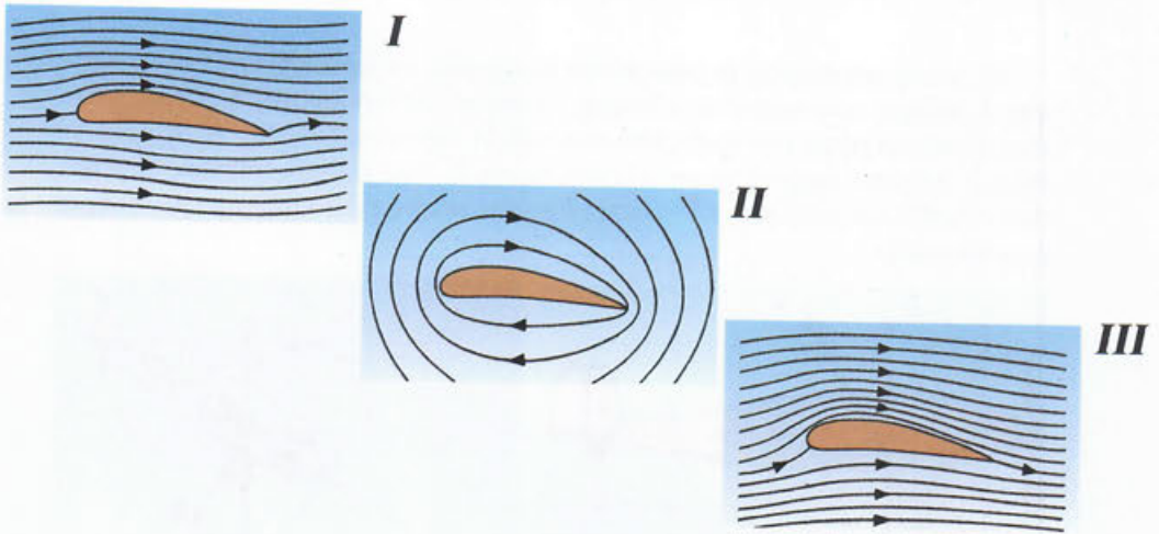
Εικόνα 7.58: Ροή γύρω από την πτέρυγα αεροπλάνου
