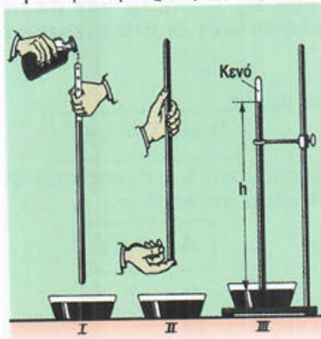
Εικόνα 7.27: Προσεγγίζοντας το πείραμα Toricelli
