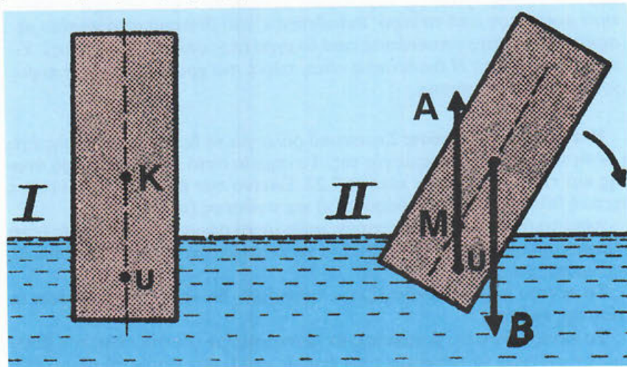
Εικόνα 7.26: Πλεύση σανίδας(ασταθής ισορροπία)
