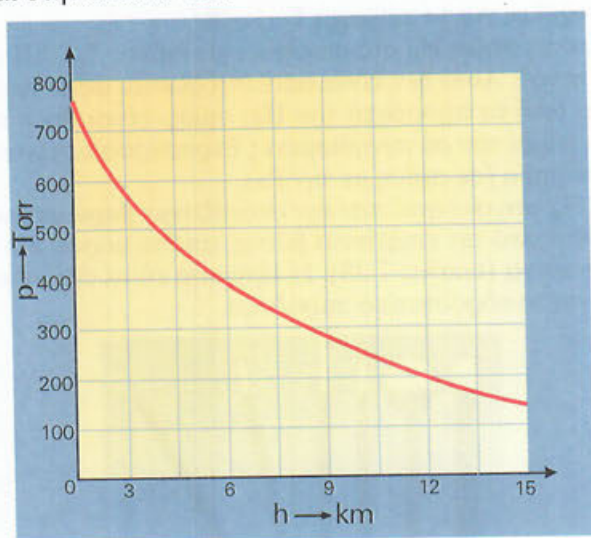
Εικόνα 7.29: Μεταβολή της ατμοσφαιρικής πίεσης με το ύψος
