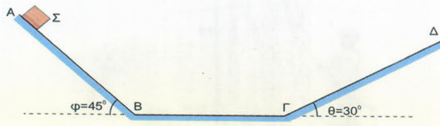
Εικόνα 5.22: Διατήρηση μηχανικής ενέργειας
