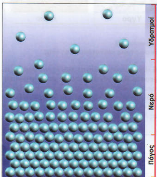
Εικόνα 2.11 Διάταξη των μορίων του H_2O στον πάγο (κάτω τμήμα της εικόνας), στο νερό (μεσαίο τμήμα) και στους υδρατμούς (άνω τμήμα)
