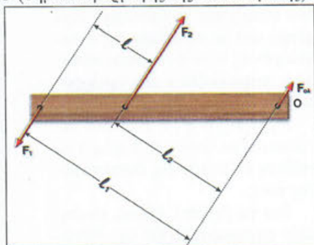
Εικόνα 3.13 Συνισταμένη δύο παράλληλων και αντίρροπων δυνάμεων
