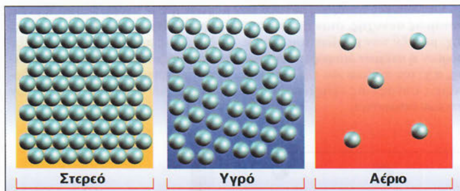
Εικόνα 2.12 Η διάταξη των μορίων στις τρεις καταστάσεις της ύλης
