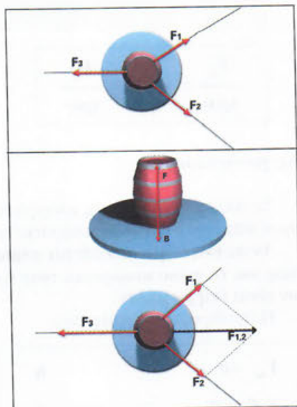
Εικόνα 2.39 Ισορροπία σώματος με την επίδραση πολλών δυνάμεων
