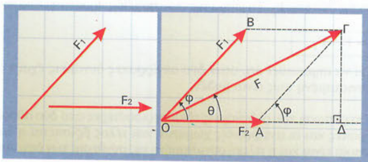
Εικόνα 2.25 Δυνάμεις που σχηματίζουν γωνία
