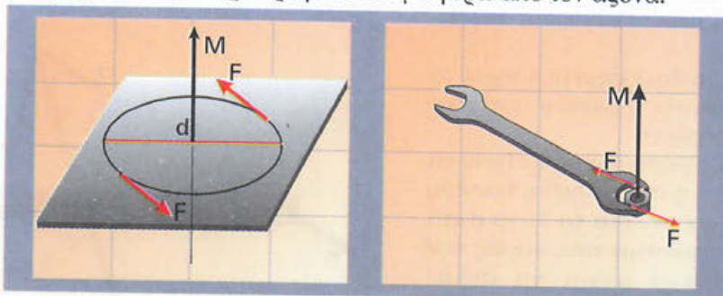
Εικόνα 3.10 Ροπή ζεύγους δυνάμεων
