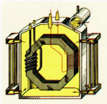
Εικόνα 3.7 Μετασχηματιστής μεγάλης ισχύος στον οποίο προβλέπεται σύστημα ψύξης
