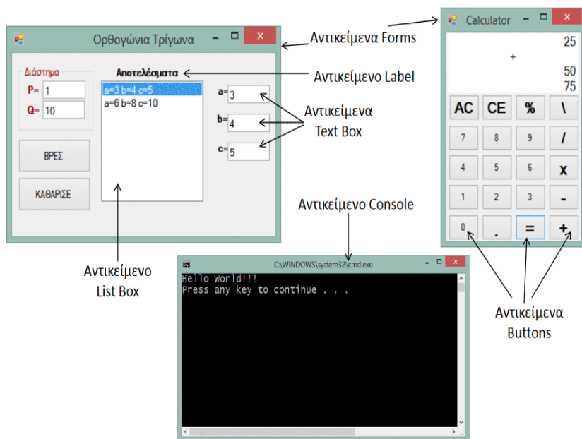
Εικόνα 2-4. Προγραμματιστικά αντικείμενα
