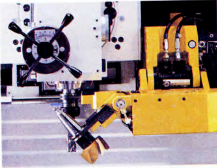
Tool changer
