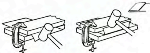
13. Hemming
