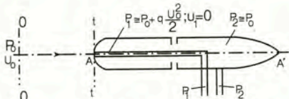
Σχήμα 16.8.ε Ταχύμετρο Pitot
