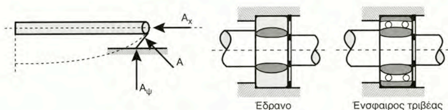
Σχήμα 8.2γ Άρθρωση
