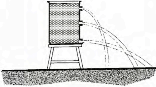
Σχήμα 15.4.6 Πειραματική απόδειξη της αύξησης της υδροστατικής πίεσης μετά του βάθους
