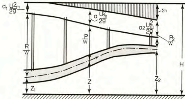
Σχήμα 16.5.6 Ο νόμος του Bernoulli σε πραγματικά υγρά
