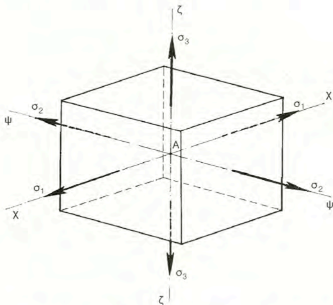
Σχήμα 12.4.3.1.α Στοιχειώδης κύβος, εντατικής κατάστασης, περί σημείο Α καταπονούμενου σώματος.
