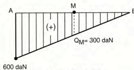
Διάγραμμα [Q]
