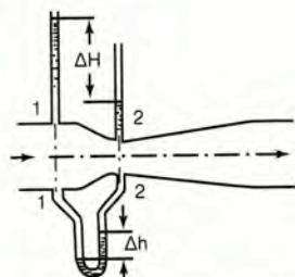
Σχήμα 16.8.α Μετρητής Βεντούρι
