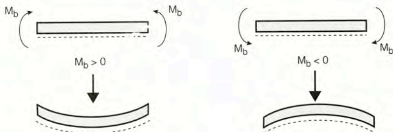
Σχήμα 8.5στ Σήμανση της M
