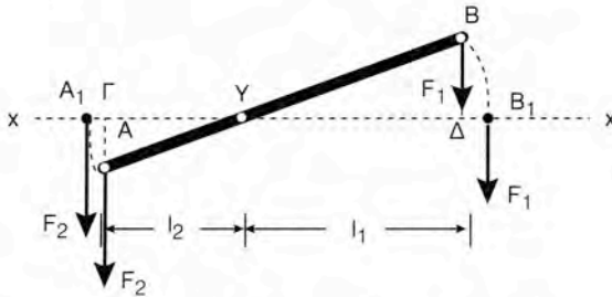
Σχήματα 13.4η και 13.4θ Χρυσούς κανών της Μηχανικής
