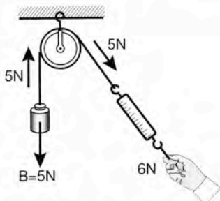
Σχήμα 13.4.2β Τροχαλία
