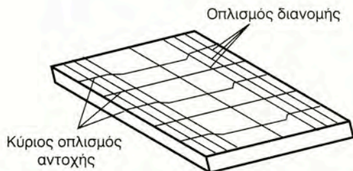
Σχήμα 10.4ε Τοποθέτηση χάλυβα σε πλάκα
