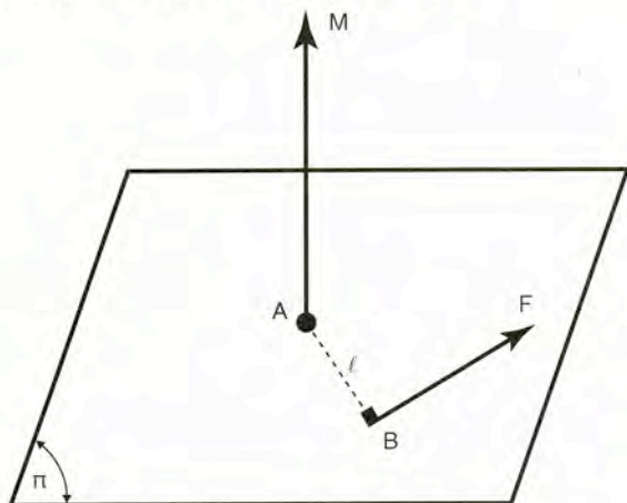
Σχήμα 2.16 Ροπή δύναμης ως προς σημείο
