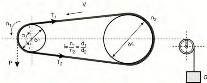
Σχήμα 13.7α Ιμαντοκίνηση
