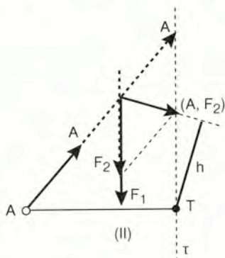
Σχήμα 8.5γ Τομή τ - τ της δοκού
