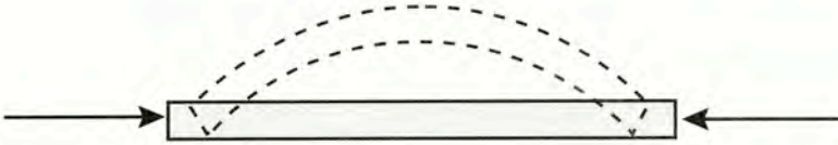
Σχήμα 10.1δ Επιμήκης κάμψη
