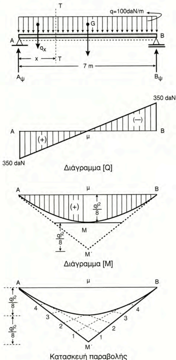
Σχήμα 8.60 Αμφιέρειστη δοκός
