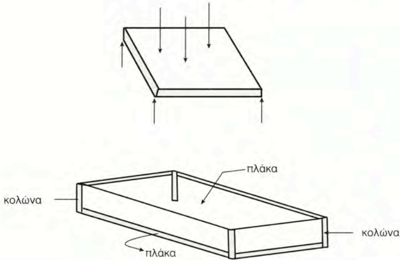
Σχήμα 8.1στ Πλάκα
