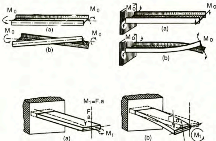
Σχήμα 11.4.6 Παραμόρφωση φορέων υποκειμένων σε στρέψη, μη κυκλικής διατομής
