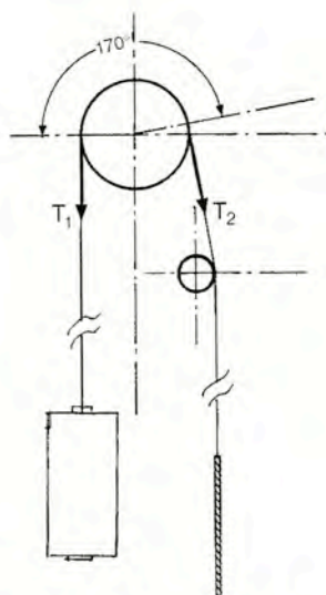
Σχήμα 14.6.2.6 Τυπική διάταξη ανελκυστήρα με τροχαλία τριβής και αντιβάρου
