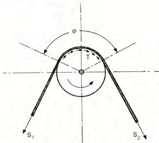
Σχήμα 14.6.2.α Η διάταξη των δυνάμεων σε τροχαλία
