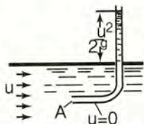
Σχήμα 16.8.δ Σωλήνας Pitot
