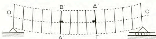
Σχήμα 8.5η Κάμψη της δοκού
