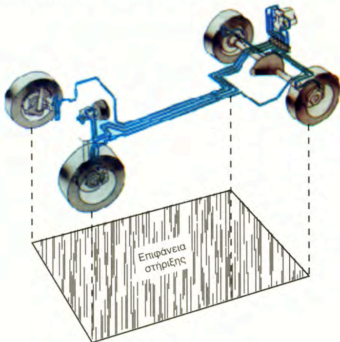
Σχήμα 4.56 Η ευστάθεια
