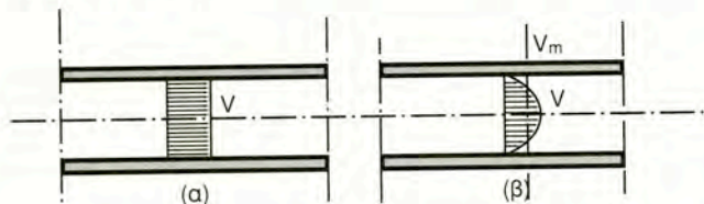
Σχήμα 16.5.α Κατανομή ταχυτήτων υγρού, μέσα σε σωλήνα α) ιδανικού υγρού β) πραγματικού υγρού
