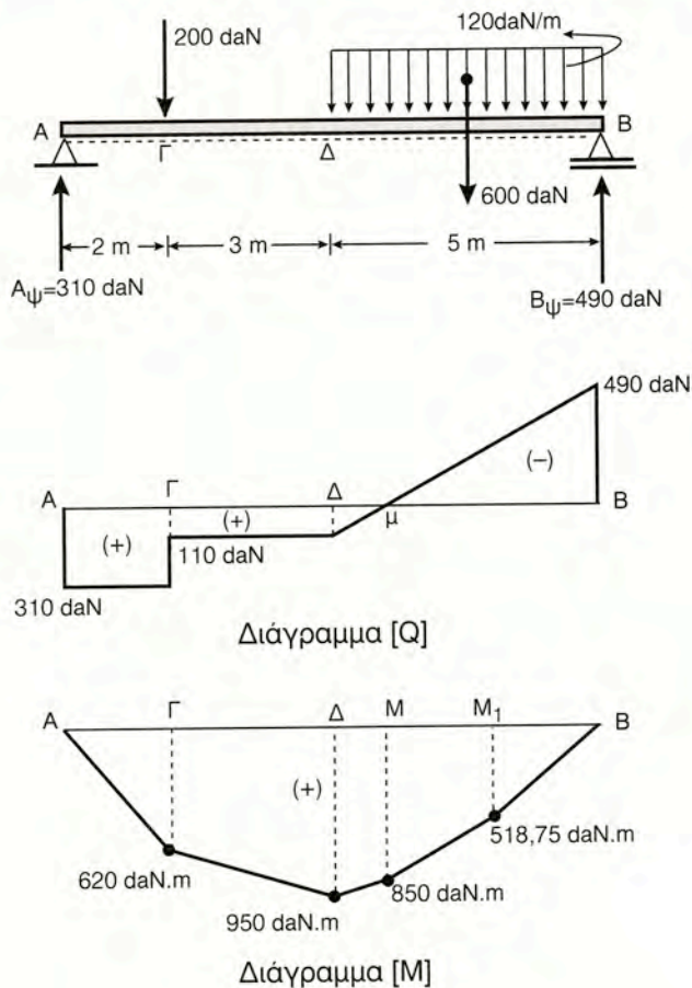
Σχήμα 8.6κ Αμφιέρειστη δοκός
