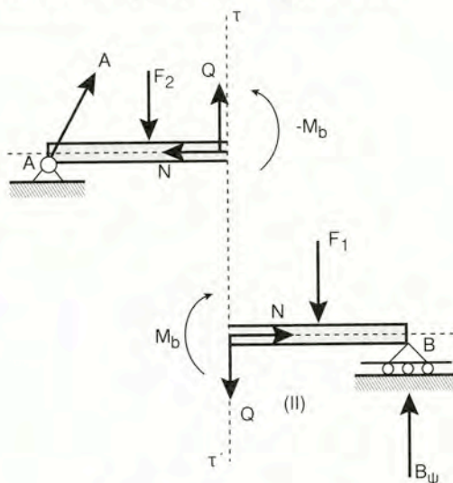
Σχήμα 8.56 Τομή τ - τ της δοκού
