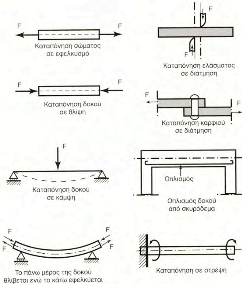
Σχήμα 5.4α Οι σπουδαιότερες καταπονήσεις
