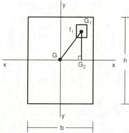
Σχήμα 7.4.2a Πολική ροπή αδράνειας διατομής
