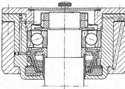
Σχήμα 14.6.4.β Εφαρμογή τριβέα κύλισης
