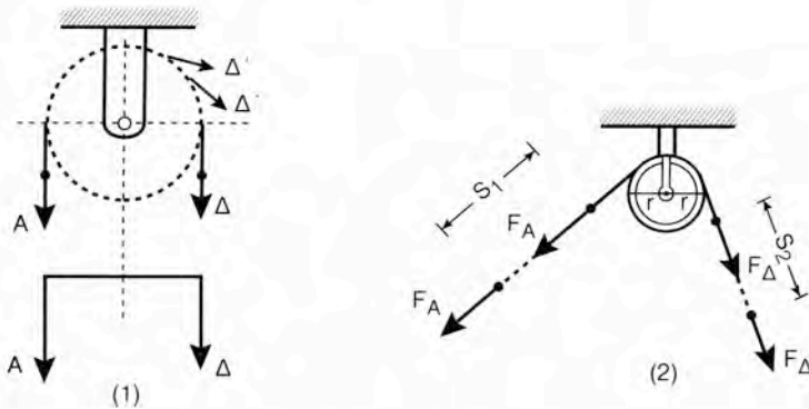
Σχήμα 13.4.2γ Τροχαλία
