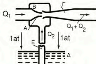
Σχήμα 16.8.γ Ψεκαστήρας
