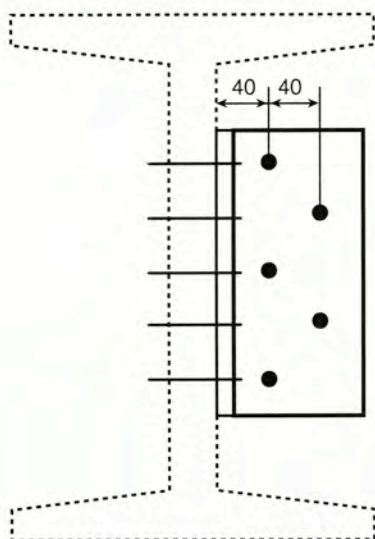
Καρφωτή σύνδεση
