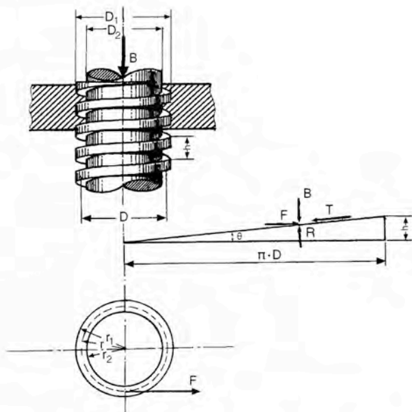
Σχήμα 14.6.3.β Κοχλίας κίνησης και το ανάπτυγμα της μέσης έλικας του σπειρώματός του.
