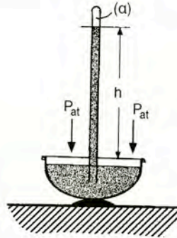
Σχήμα 15.8.β Βαρόμετρο Torricelli
