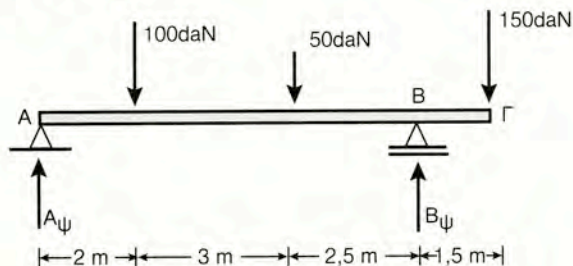
Σχήμα 8.36 Μονοπροέχουσα δοκός
