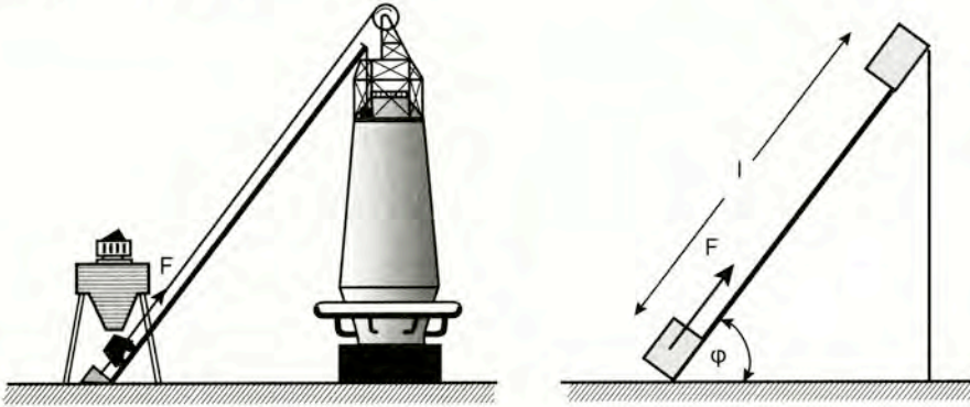
Σχήμα 13.5α Κεκλιμένο επίπεδο
