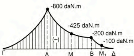
Διάγραμμα [M]
