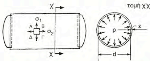
Σχήμα 12.4.3.2.α Λέβητας υπό πίεση. Υπόκειται σε διαξονική καταπόνηση
