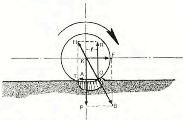
Σχήμα 14.4.γ Ισοσταχής κύλιση κύλινδρου σε οριζόντιο επίπεδο.
