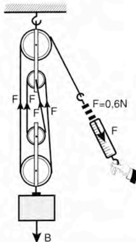
Σχήμα 13.4.2ζ Πολύσπαστο με δύο τροχαλιοθήκες των δύο τροχαλιών η κάθε μία
