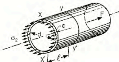
Σχήμα 12.4.3.26 Οι δυνάμεις στον πυθμένα λέβητα υπό πίεση
