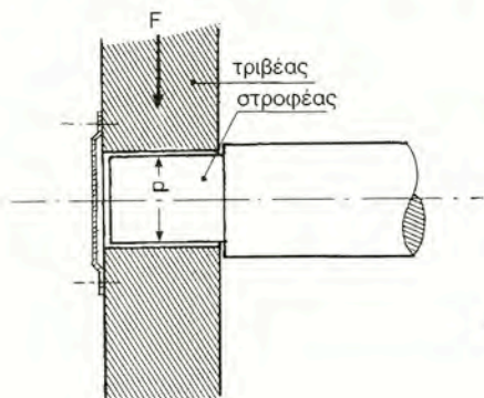
Σχήμα 14.6.1.α Ακτινικός στροφέας
