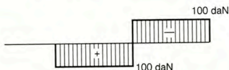
Διάγραμμα [Q]
