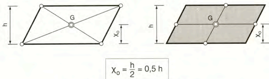
Σχήμα 4.3β Το κεντροειδές παραλληλογράμμου
