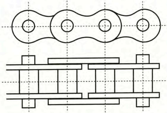
Σχήμα 13.7ζ Αλυσοκίνηση
