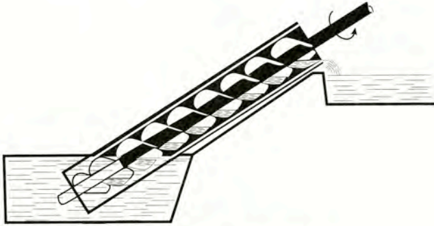
Σχήμα 13.66 Κοχλίας
