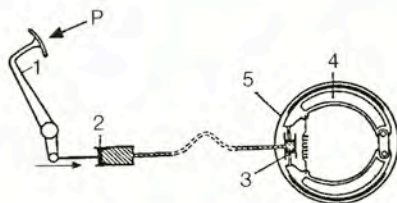
Σχήμα 15.9.2.α Υδραυλικό φρένο αυτοκινήτου
