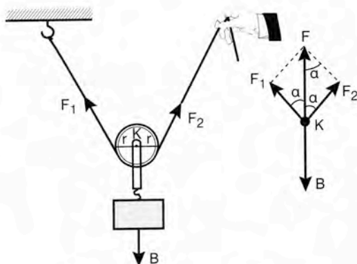
Σχήμα 13.4.2στ Κινητή τροχαλία
