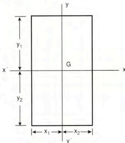
Σχήμα 7.4.1α Ροπή αντίστασης
