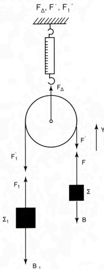
Σχήμα 13.4.2δ Πάγια τροχαλία
