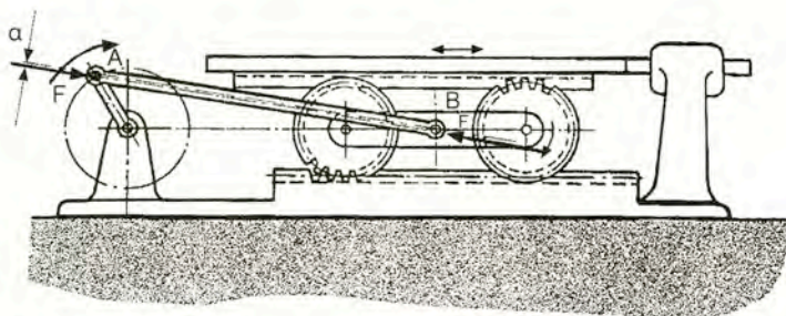
Σχήμα 12.3.3.α Στον μηχανισμό διωστήρα στροφάλου, το βάκτρο AB υπόκειται σε θλίψη και εφελκυσμό εναλλάξ
