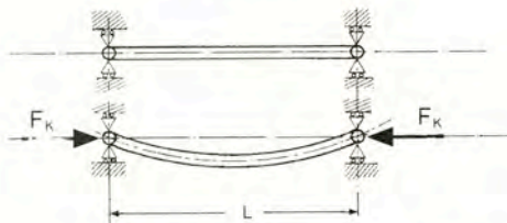
Σχήμα 12.3.4.α Η ράβδος του Euler
