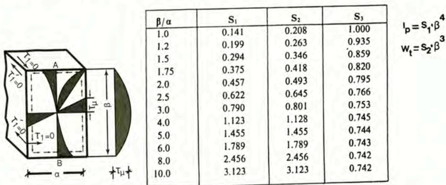
Σχήμα 11.5.δ Ορθογωνική διατομή. Η διανομή των τάσεων λόγω στρεπτικής ροπής
