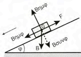
Σχήμα 13.25 Το φορτίο κατέρχεται
