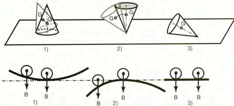
Σχήμα 4.5α Ευσταθής ισορροπία, ασταθής και αδιάφορη
