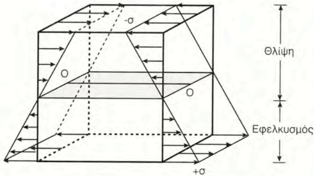
Σχήμα 8.5θ Κάμψη της διατομής της δοκού
