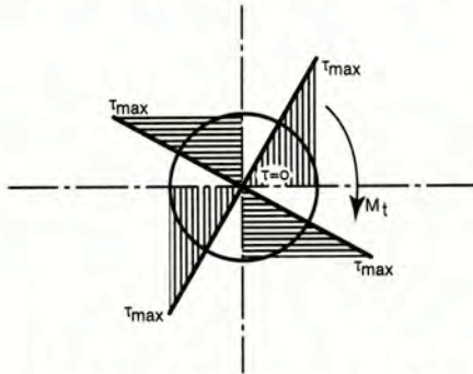
Σχήμα 11.2.6 Η διανομή των τάσεων σε κυκλική διατομή
