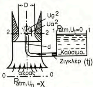
Σχήμα 16.8.β Εξαερωτής
