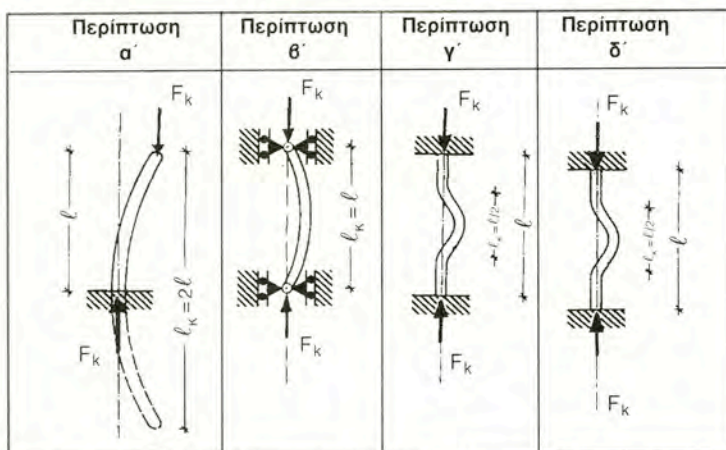
Σχήμα 12.3.5 Οι βασικές περιπτώσεις στερέωσης ράβδων, καταπονούμενων σε λυγισμό και το κατά περίπτωση ανηγμένο μήκος λυγισμού.
