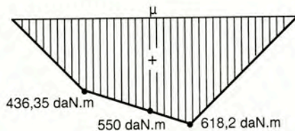
Διάγραμμα [M]
