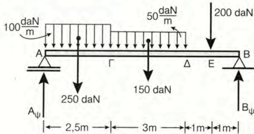
Σχήμα 8.3στ Αμφιέρειστη δοκός
