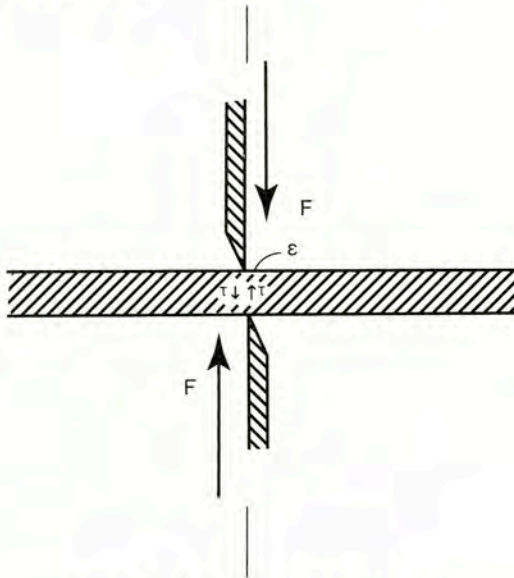
Σχήμα 9.5.α Διάτμηση ή ψαλλιδισμός
