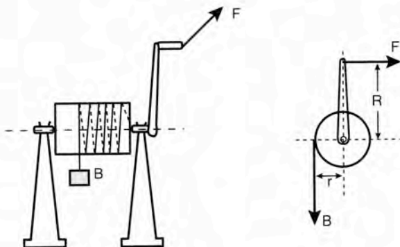
Σχήμα 13.4.3α Βαρούλκο
