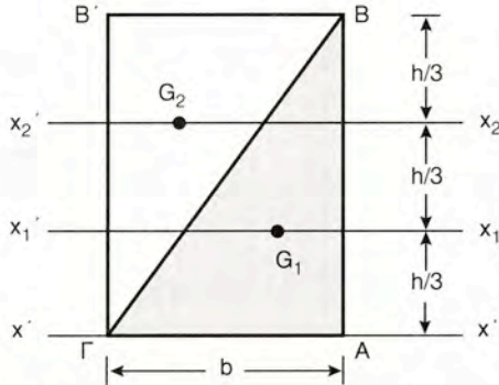
Σχήμα 7.66 Ροπή αδράνειας τριγωνικής διατομής
