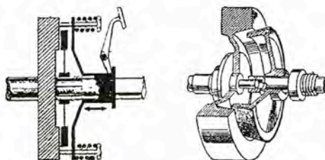
Σχήμα 14.6.6.6 Είδη συμπλεκτών
