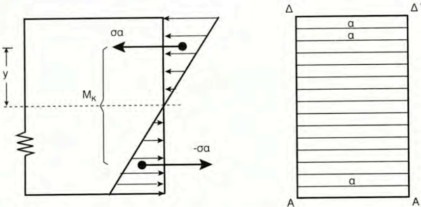
Σχήμα 10.26 Εσωτερικές δυνάμεις-τάσεις- σε διατομή της δοκού.
