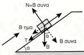
Σχήμα 13.5γ Φορτίο σε κεκλιμένο επίπεδο
