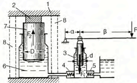
Σχήμα 15.9.1.6 Παράσταση υδραυλικού πιεστήριου
