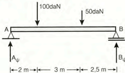
Σχήμα 8.3α Αμφιέρειστη δοκός
