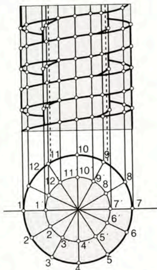
Σχήμα 13.6δ Τετραγωνικό σπείρωμα
