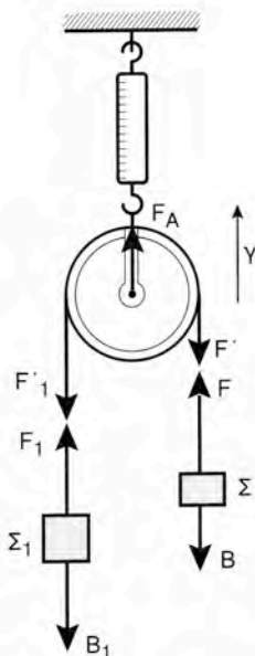
Σχήμα 13.4.2α Τροχαλία
