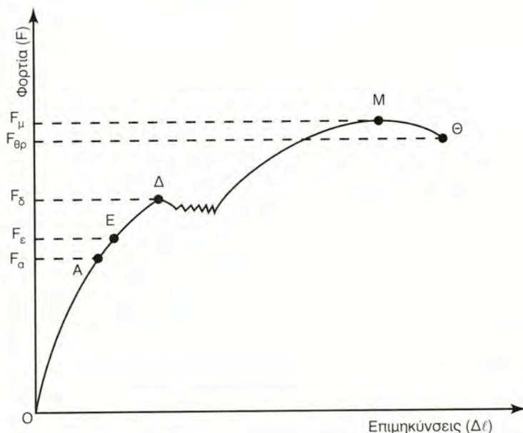
Σχήμα 5.8β Διάγραμμα επιμηκύνσεων - Φορτίων
