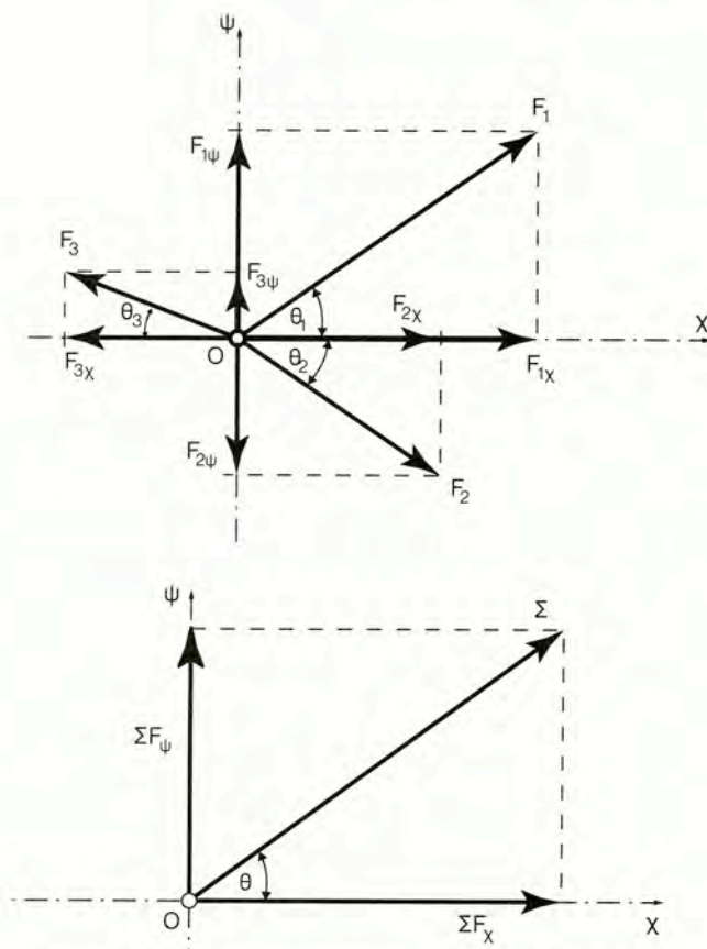
Σχήμα 3.26 Συνισταμένη πολλών ομοεπιπέδων δυνάμεων.
