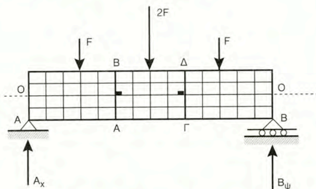
Σχήμα 8.5ζ Κάμψη της δοκού. Ουδέτερος άξονας 0-0
