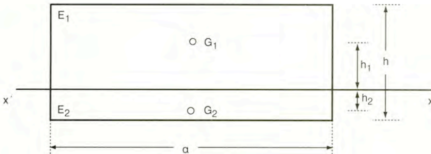
Σχήμα 7.36 Στατική ροπή ορθογωνικής διατομής
