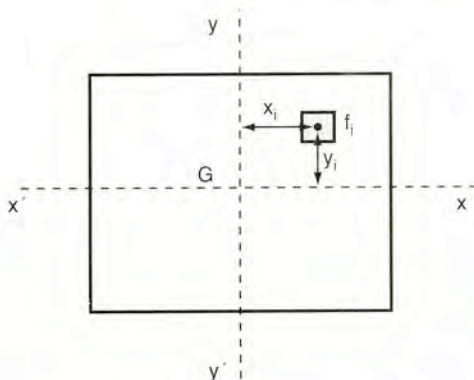
Σχήμα 7.2α Εύρεση ροπής αδράνειας διατομής
