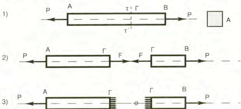
Σχήμα 5.5α Οι ορθές εφελκυστικές τάσεις
