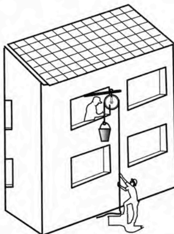
Σχήμα 13.1α Ανύψωση βάρους
