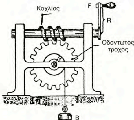
Σχήμα 13.6στ Ατέρμων κοχλίας
