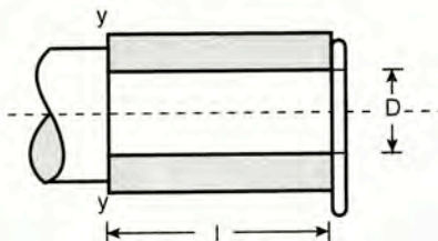
Σχήμα 10.4ζ Στροφέας καταπονούμενος σε κάμψη
