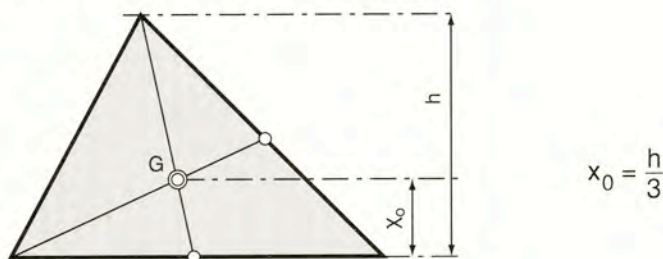
Σχήμα 4.3δ Κεντροειδές επιφάνειας τριγώνου
