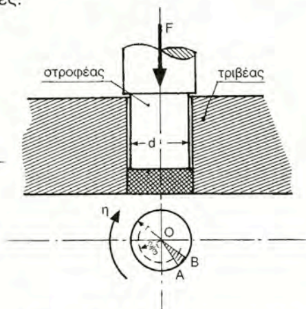
Σχήμα 14.6.1.β Αξονικός στροφέας
