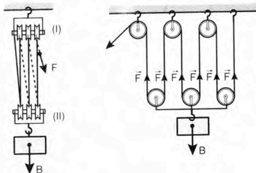
Σχήμα 13.4.2η Κινητή τροχαλιοθήκη
