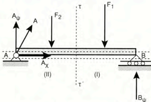
Σχήμα 8.5α Δοκός σταθερής διατομής
