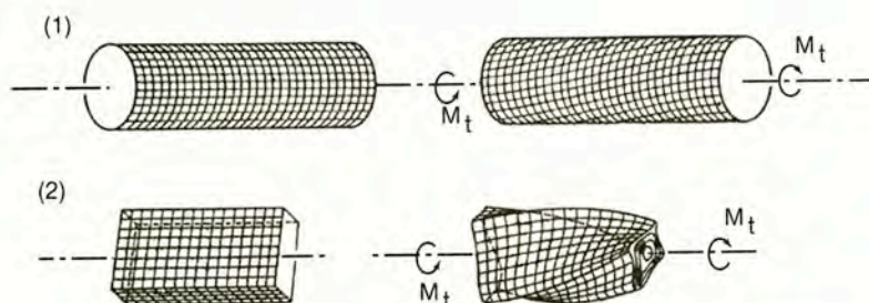
Σχήμα 11.4.α Η πειραματική απόδειξη της ιδιομορφίας της στρέψης
