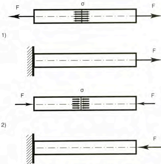
Σχήμα 6.1α Εφελκυσμός και θλίψη ράβδου.
