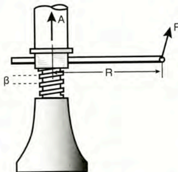
Σχήμα 13.6ε Κοχλίας
