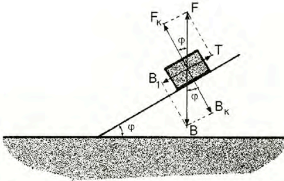
Σχήμα 14.4.8 Σώμα ολισθαίνον σε κεκλιμένο επίπεδο
