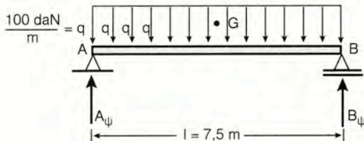
Σχήμα 8.3δ Αμφιέρειστη δοκός
