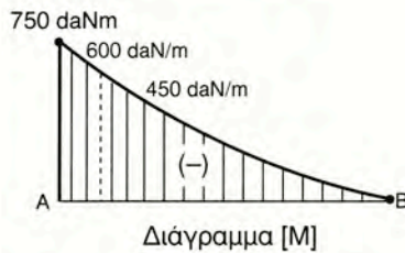
Σχήμα 8.6η Πρόβολος
