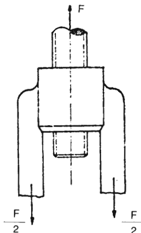
Εικ.14.4.6 Σφιγκτήρας παραδείγματος 2
