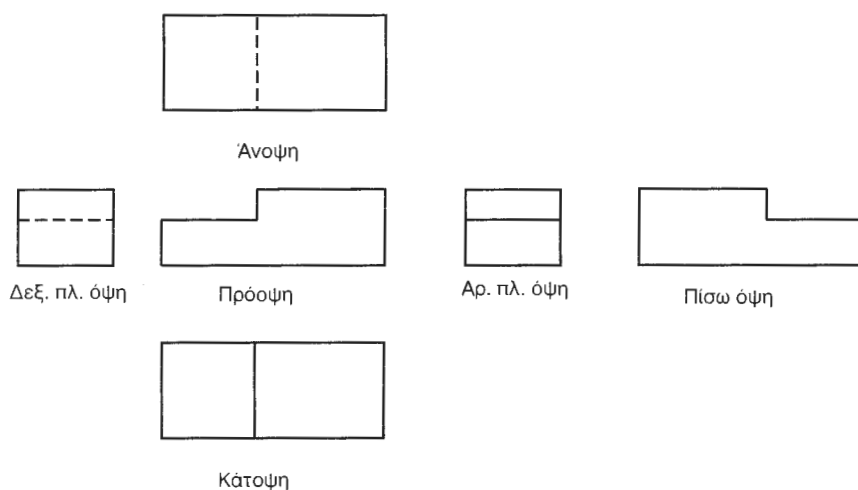
Εικ. 4.1 η Οι θέσεις των εξι όψεων στο χαρτί σχεδίασης
