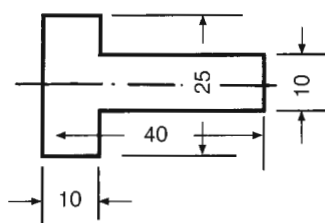
Εικ. 6.3ε Οι γραμμές διαστάσεων δεν πρέπει να κόβουν τις γραμμές του σχεδίου.
