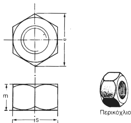
Εικ. 7.3ζ Διαστάσεις περικοχλίου
