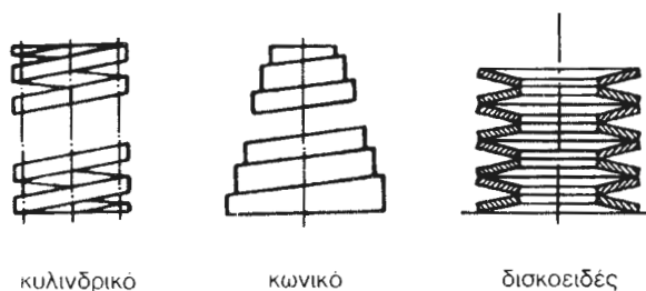
Εικ. 7.6α Ελικοειδή ελατήρια - δισκοειδή ελατήρια
