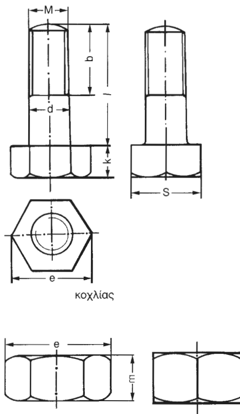
Εικ. 7.31γ Σχεδίαση εξάγωνου κοχλίας και περικοχλίου
