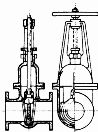
Εικ.12.4δ Βάνα
