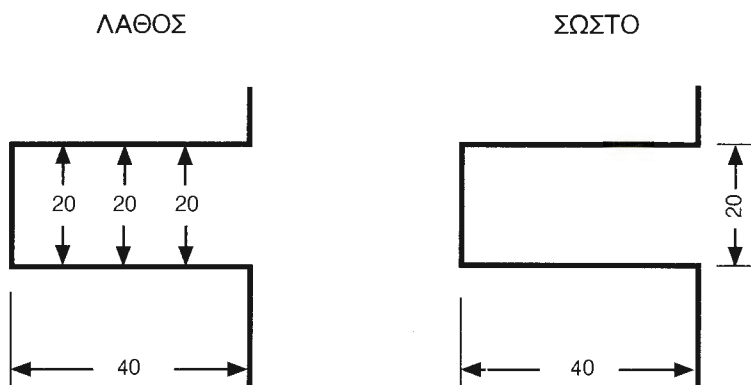
Εικ. 6.39 Οι αριθμοί των διαστάσεων στο μηχανολογικό σχέδιο συμβολίζουν πάντα mm γι' αυτό και δεν αναγράφεται η μονάδα μέτρησης δίπλα τους. Οι αριθμοί των διαστάσεων είναι γραμμένοι κατακόρυφα ή οριζόντια (στροφή 90^\circ αντίστροφα από τους δείκτες του ωρολογίου).
