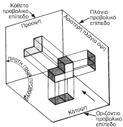
Εικ. 6.2α Τα προβολικά επίπεδα σχηματίζουν τέσσερις γωνίες καθώς αλληλοτέμνονται
