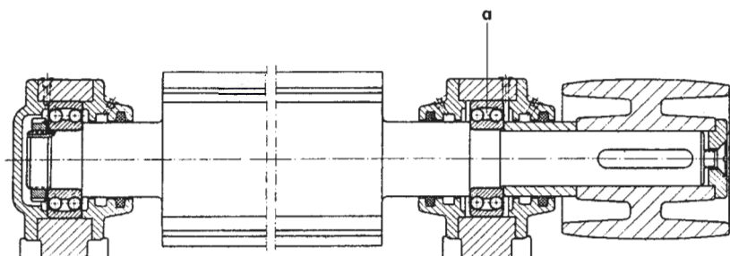
Εικ. 13.1ε Άξονας μηχανής πλανίσματος ξύλων, ο οποίος φέρει στο κέντρο του το κοπτικό εργαλείο και στην άκρη του τύμπανο για την περιστροφή του με τη βοήθεια επίπεδου μάντα
