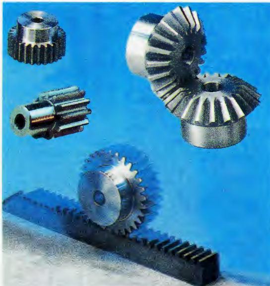
Εικ. 10.1.6 Οδοντώσεις: Παράλληλοι, κωνικοί τροχοί, οδοντωτός κανόνας.
