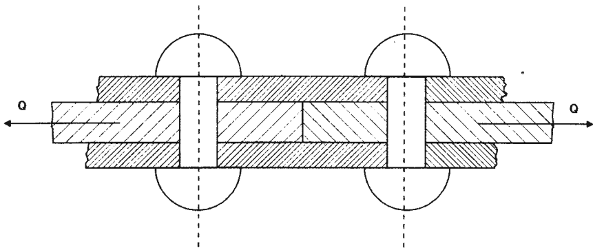
Εικ. 14.3.6 Ήλωση παραδείγματος 1
