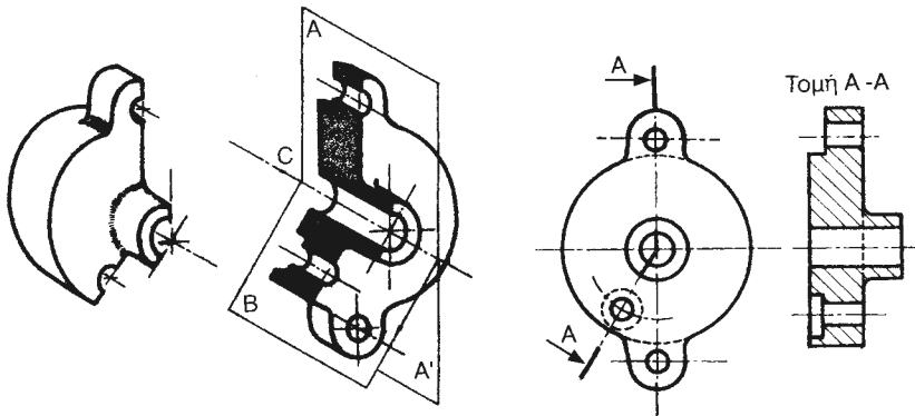
Εικ. 6.20 Ημιτομή κατά το επίπεδο Α-Α
