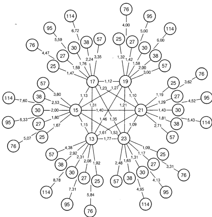
Εικ. 10.3.16 Αριθμοί δοντιών τυποποιημένων αλυσοτροχών και αντίστοιχες δυνατές σχέσεις μετάδοσης
