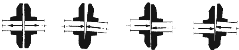
Εικ. 9.3ια Γεωμετρικά σφάλματα τοποθέτησεως εύκαμπτων συνδέσμων
