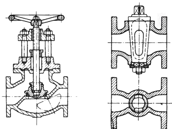
Εικ.12.4ε Κρουνός
