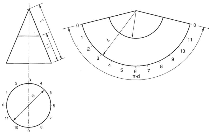
Εικ. 5.7στ Ανάπτυγμα κóλουρου κώνου
