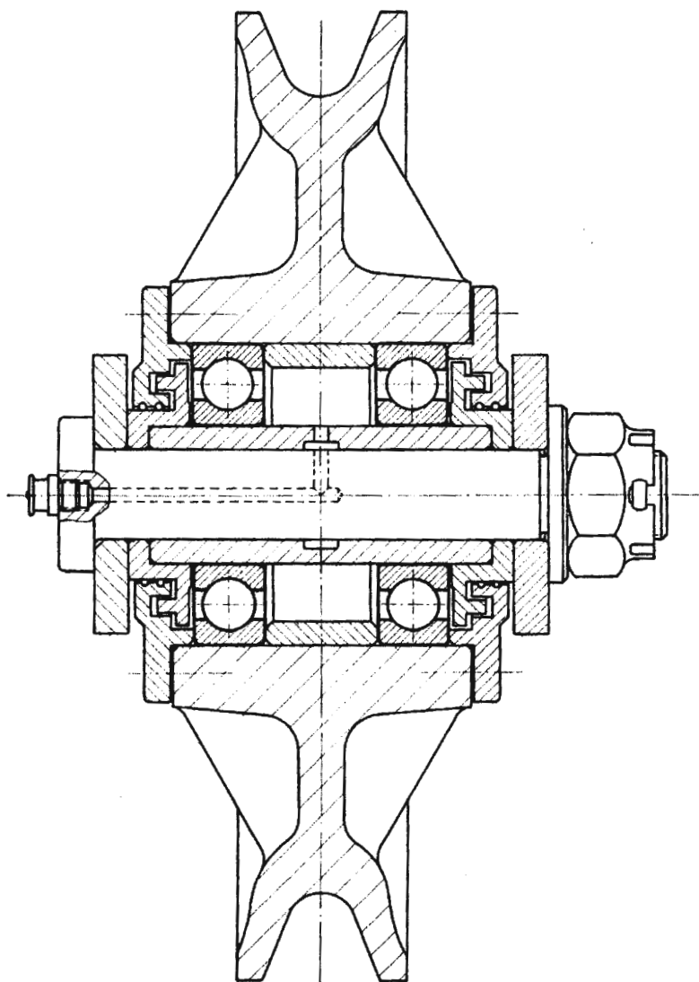
Εικ. 13.1στ Τροχαλία συρματόσχοινου
