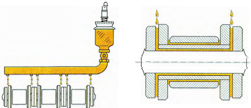
Εικ.10.3.1δ Λίπανση σταγόνων. Δεξιά φαίνονται τα σημεία που πρέπει να λιπανθούν
