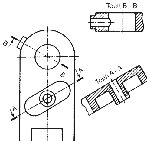
Εικ. 6.21 Μερικές τομές κατά τα επίπεδα Α-Α και Β-Β
