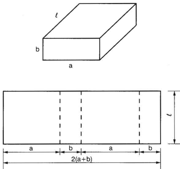
Εικ. 5.7α Ανάπτυγμα ορθογωνίου
