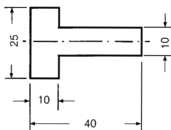
Εικ. 6.3ε Οι γραμμές διαστάσεων δεν πρέπει να κόβουν τις γραμμές του σχεδίου.
