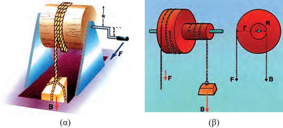
Εικόνα 5.10: Το βαρούλκο
