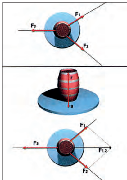
Εικόνα 2.39 Ισορροπία σώματος με την επίδραση πολλών δυνάμεων
