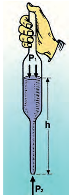
Εικόνα 7.31: Το σιφώνι
