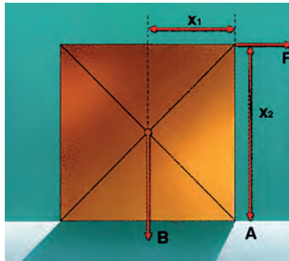
Εικόνα 3.20 Ισορροπία κιβωτίου
