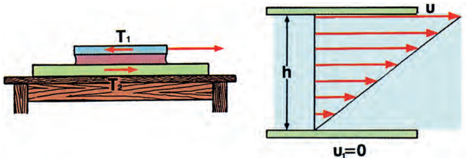
Εικόνα 7.47: Για τη μελέτη της εσωτερικής τριβής στα υγρά
