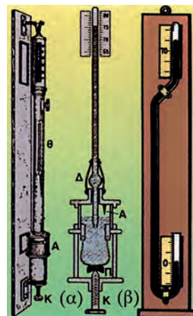
Εικόνα 7.36: Βαρόμετρα
