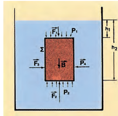
Εικόνα 7.23: Υπολογισμός της άνωσης
