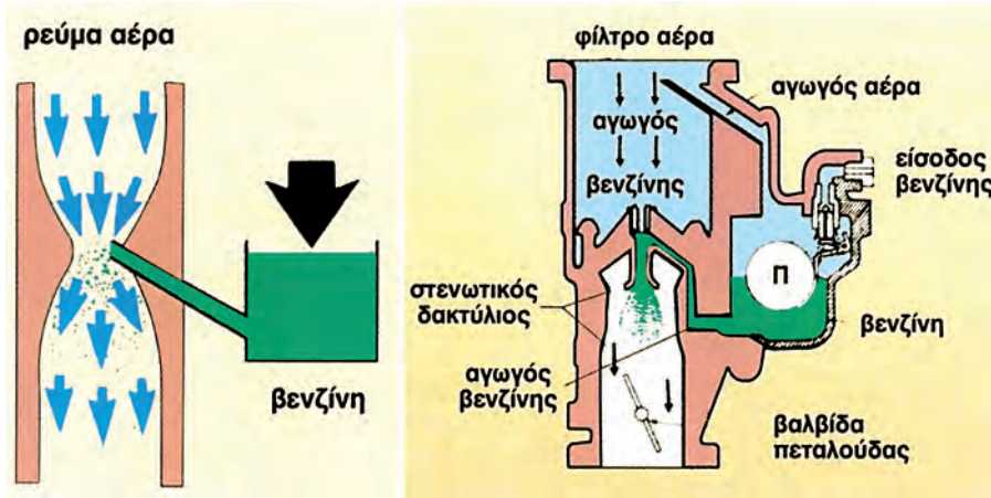
Εικόνα 7.44 (δ, ε): Η αρχή λειτουργίας και η διάταξη στον εξασερωτήρα (καρπιρατέρ) αυτοκινήτου
