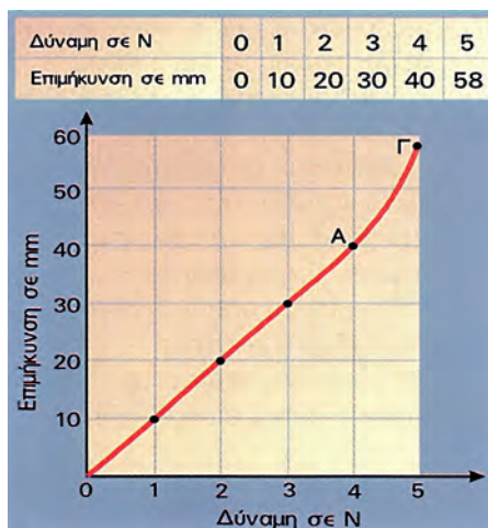
Εικόνα 2.17 Χαρακτηριστική ελατηρίου
